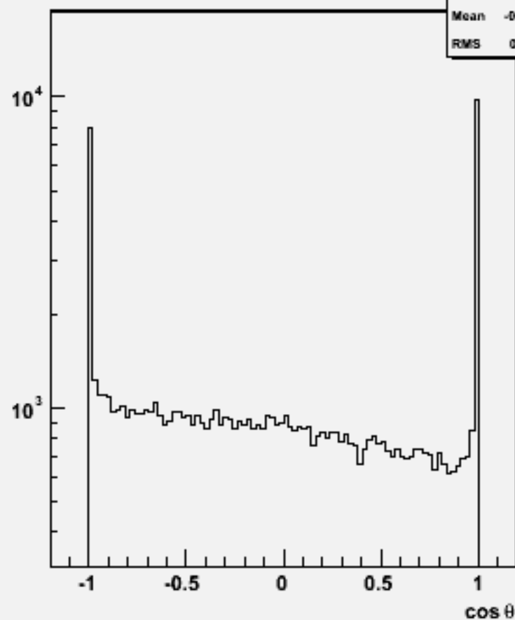
Particle cos \theta : w100385 n1e1e3n3_o
