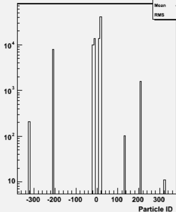
Particle ID : w100385 n1e1e3n3_o
