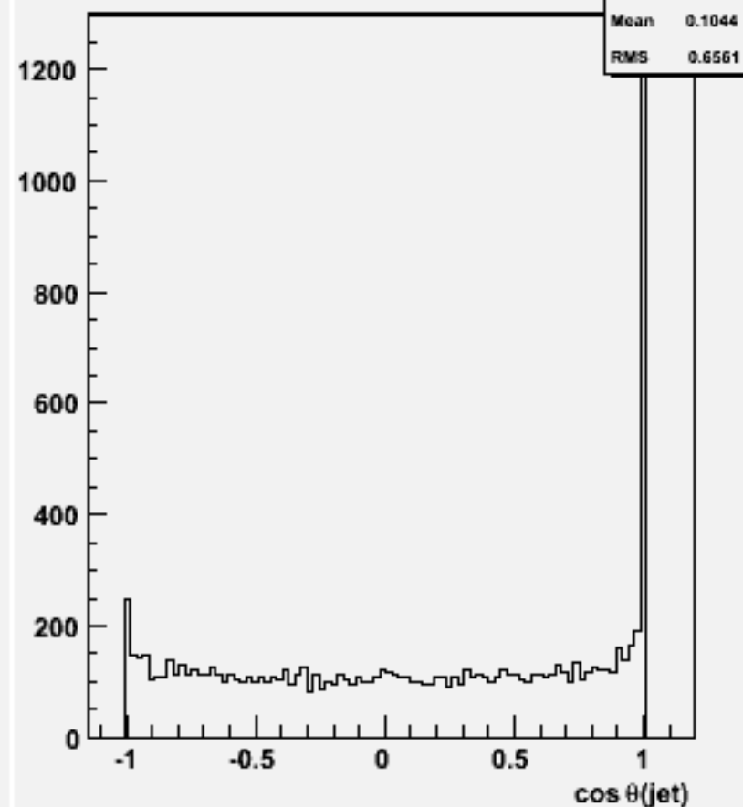
cos \theta for 2-jets :w100385 n1e1e3n3_o
