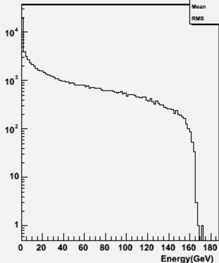
Particle Energy : w100385 n1e1e3n3_o
