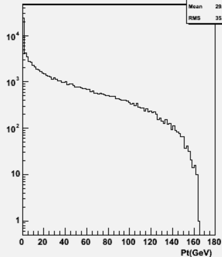
Particle Pt : w100385 n1e1e3n3_o
