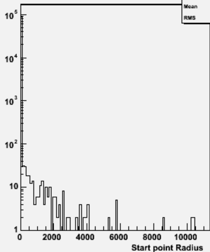
Start point R : w100385 n1e1e3n3_o
