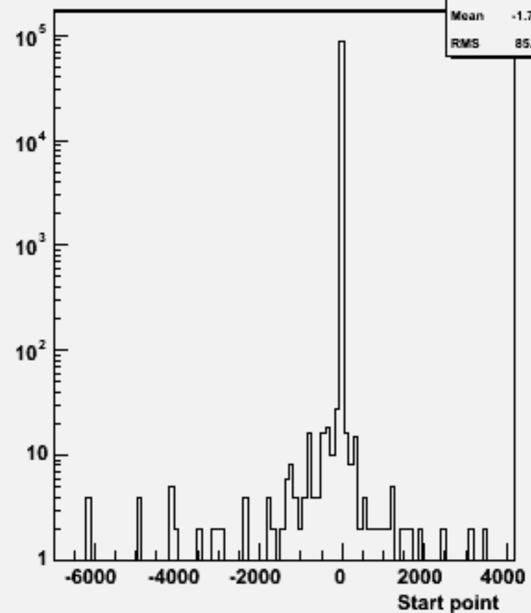
Start point Z : w100385 n1e1e3n3_o
