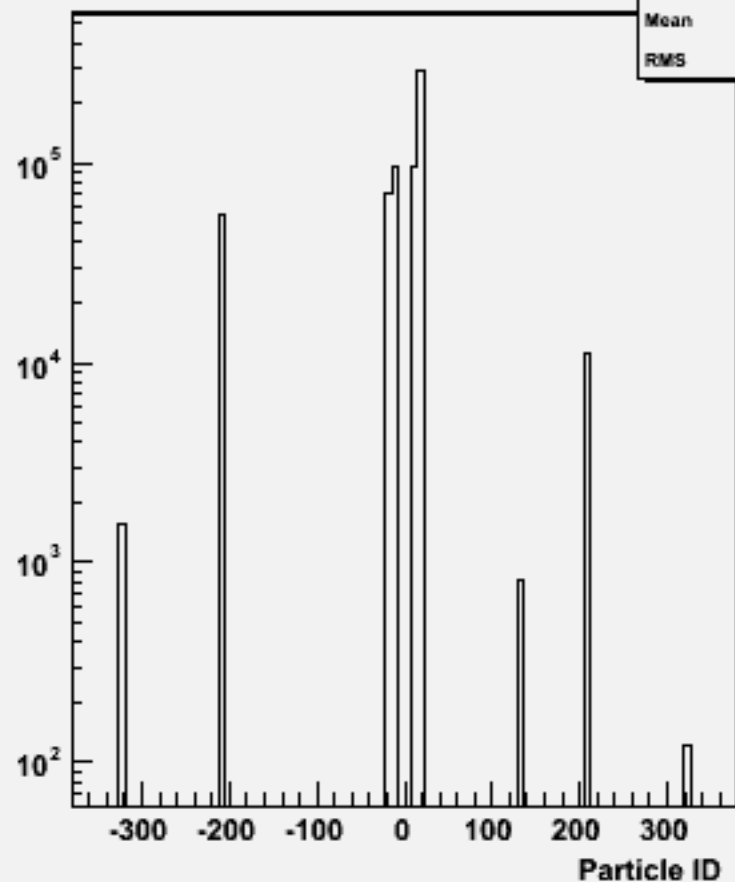
Particle ID : w100383 n1e1e3n3_o
