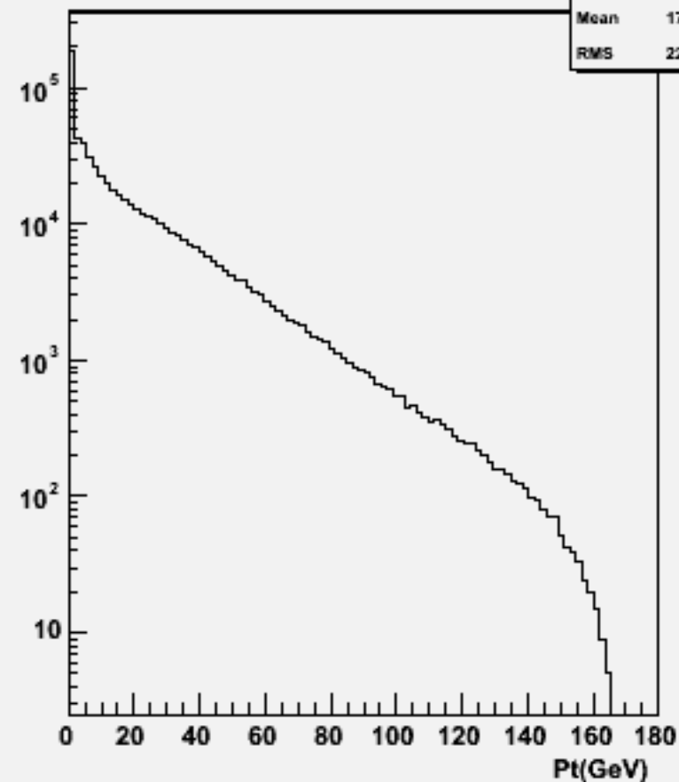
Particle Pt : w100383 n1e1e3n3_o
