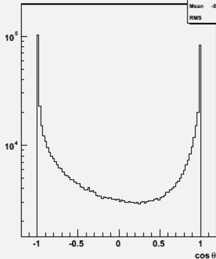
Particle cos \theta : w100383 n1e1e3n3_o
