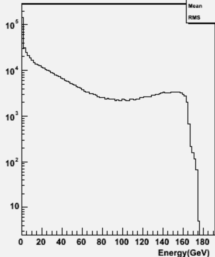
Particle Energy : w100383 n1e1e3n3_o
