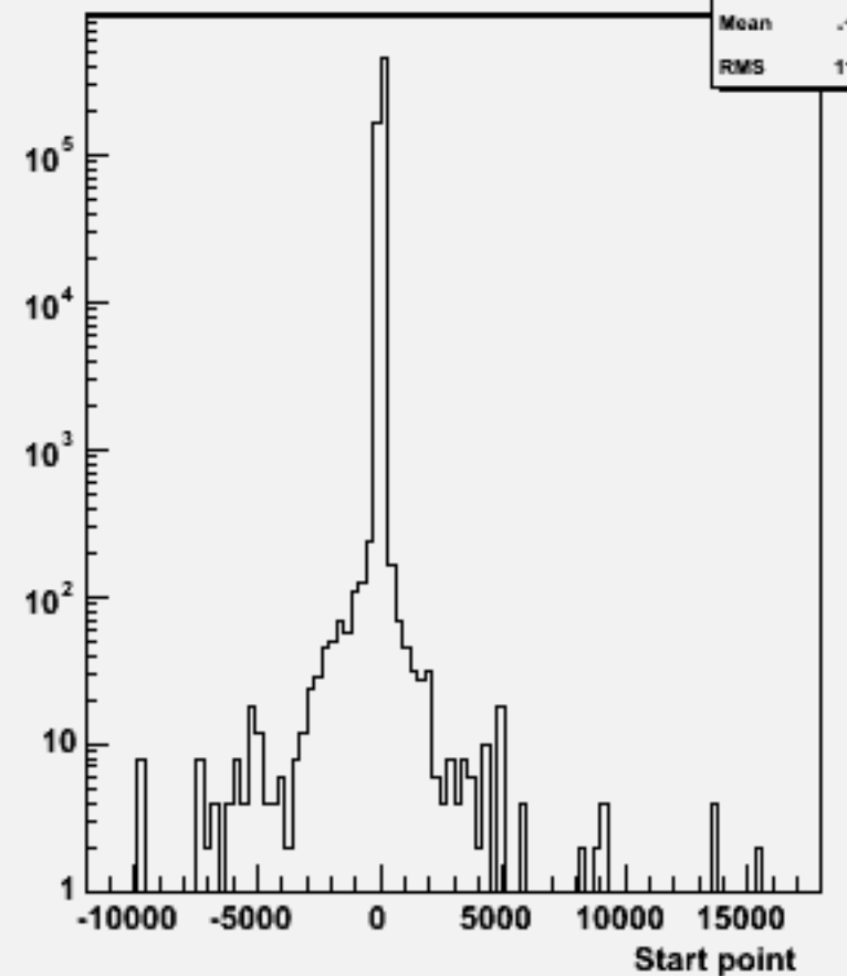
Start point Z : w100383 n1e1e3n3_o
