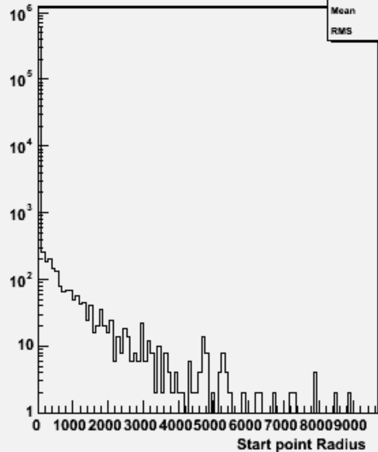
Start point R : w100383 n1e1e3n3_o
