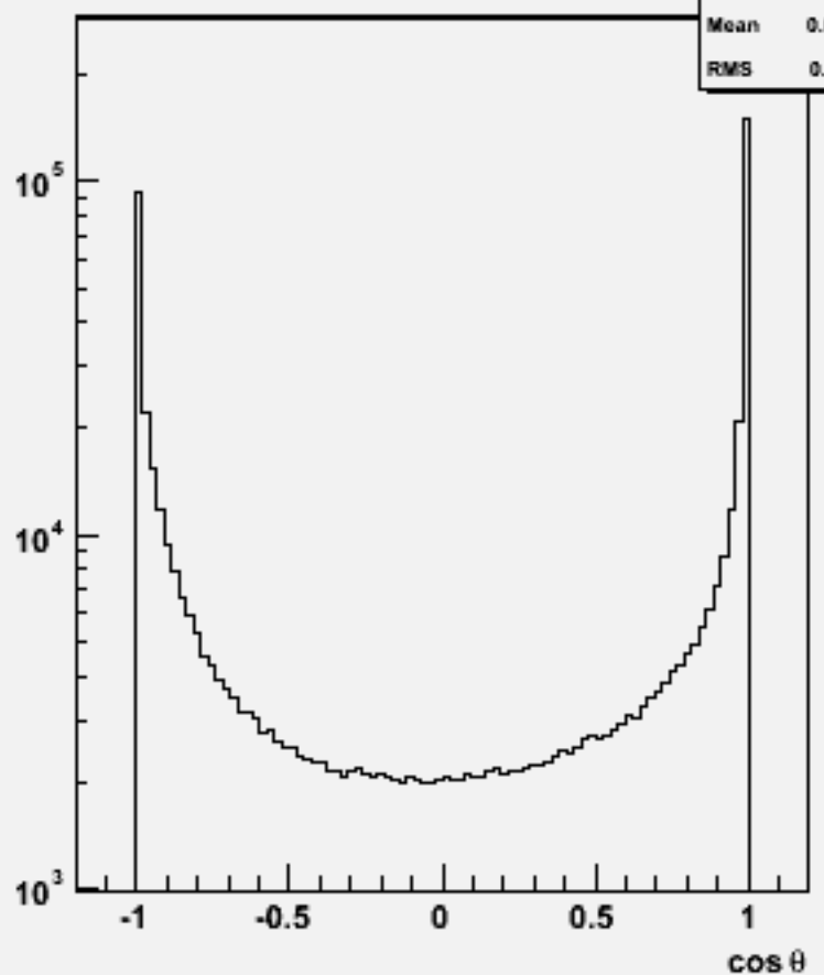
Particle cos \theta : w100378 n1e1e1n1_o
