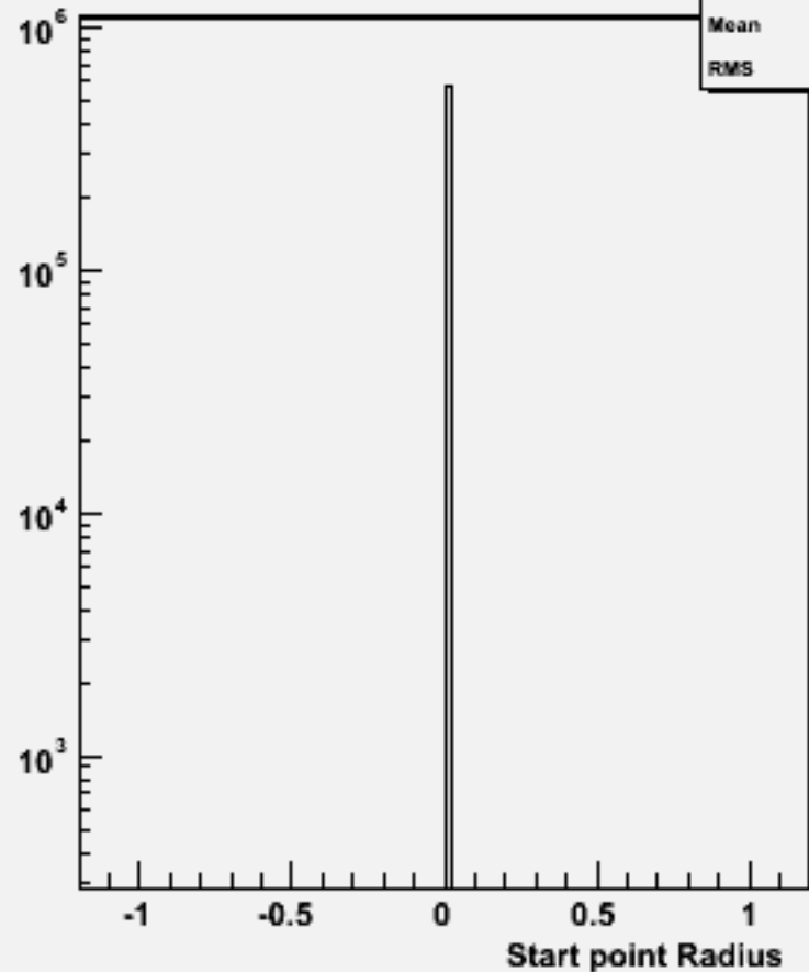
Start point R : w100378 n1e1e1n1_o
