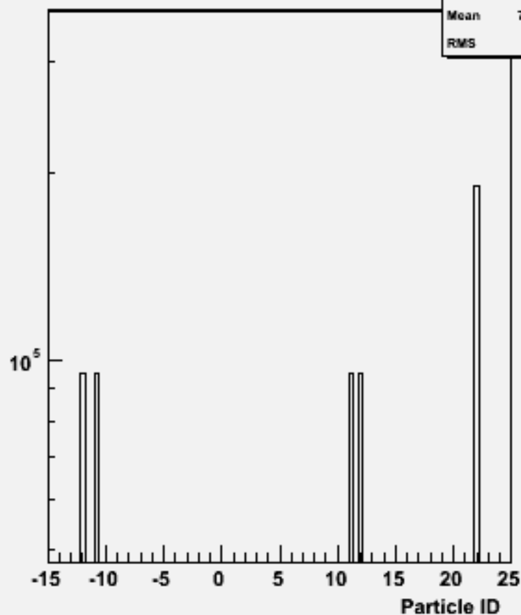
Particle ID : w100378 n1e1e1n1_o
