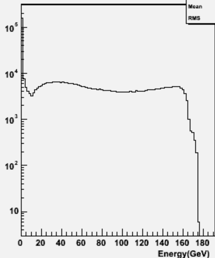
Particle Energy : w100378 n1e1e1n1_o
