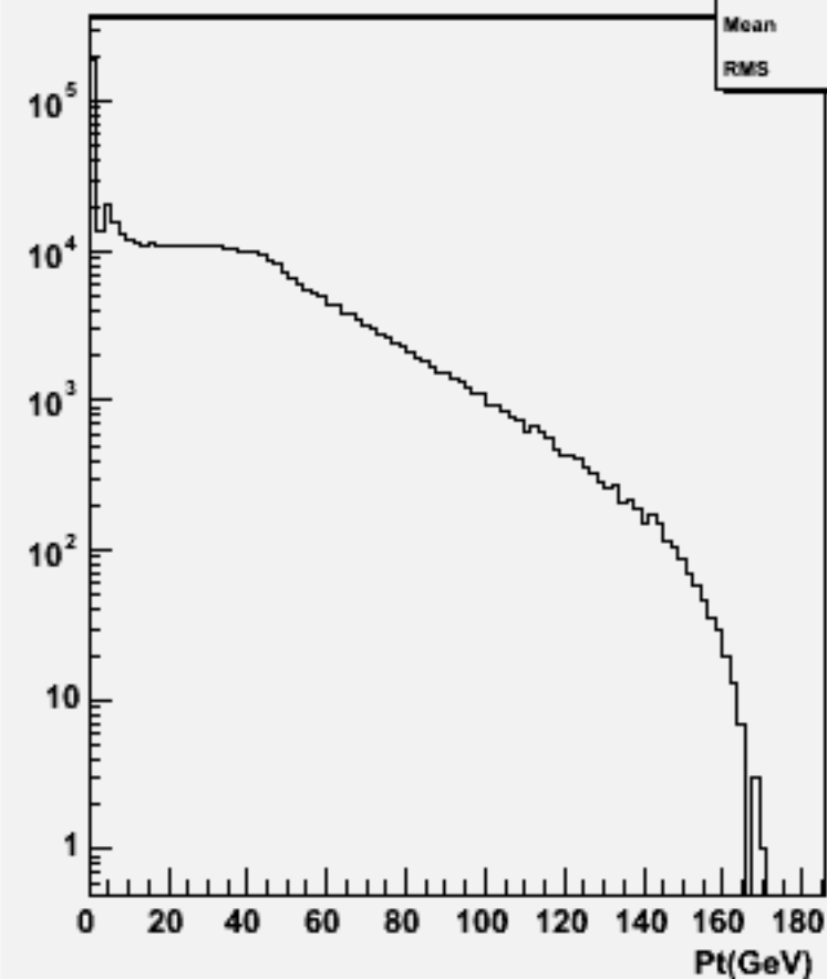
Particle Pt : w100378 n1e1e1n1_o
