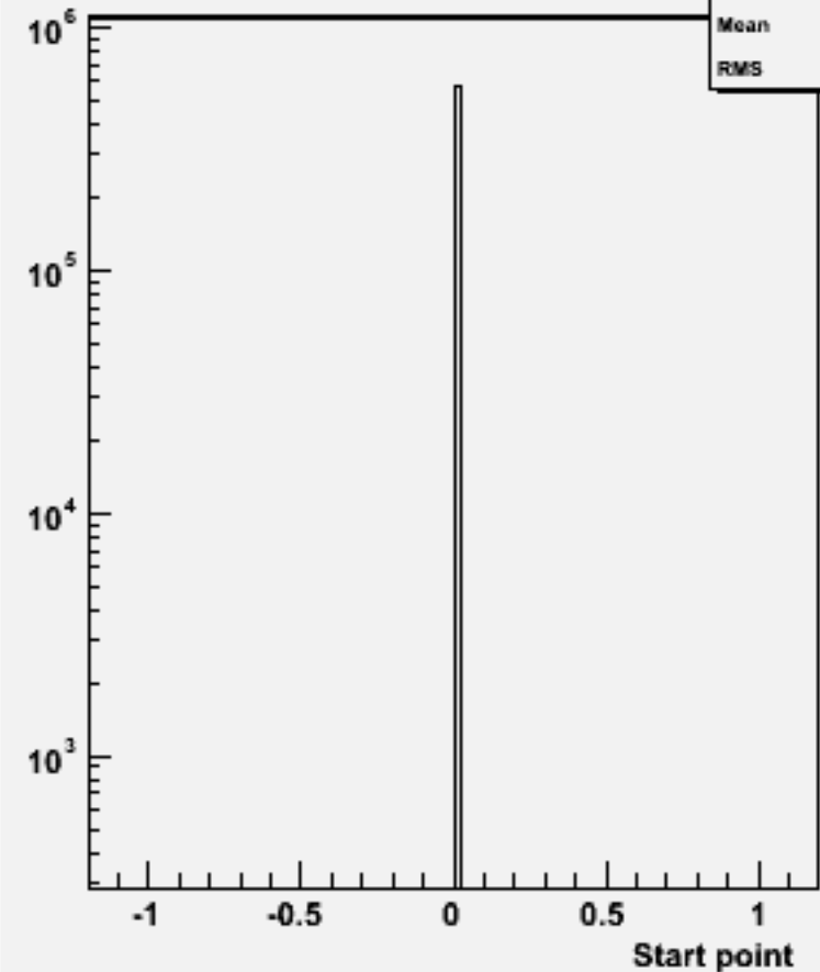
Start point Z : w100378 n1e1e1n1_o
