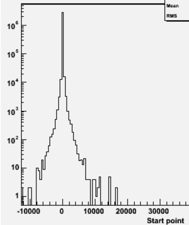
Start point Z : w100356 e2e2h_o
