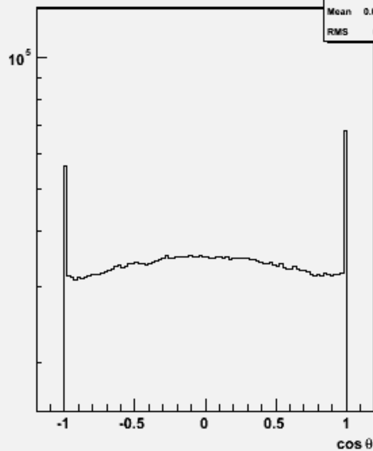
Particle cosθ : w100356 e2e2h_o
