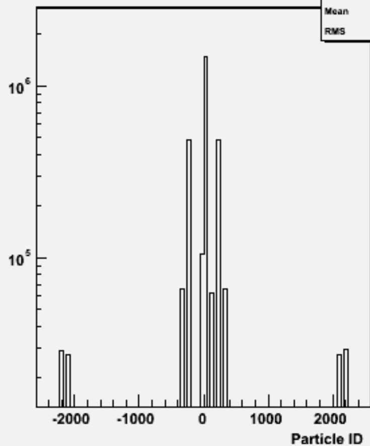
Particle ID : w100356 e2e2h_o
