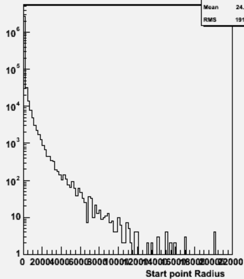
Start point R : w100356 e2e2h_o
