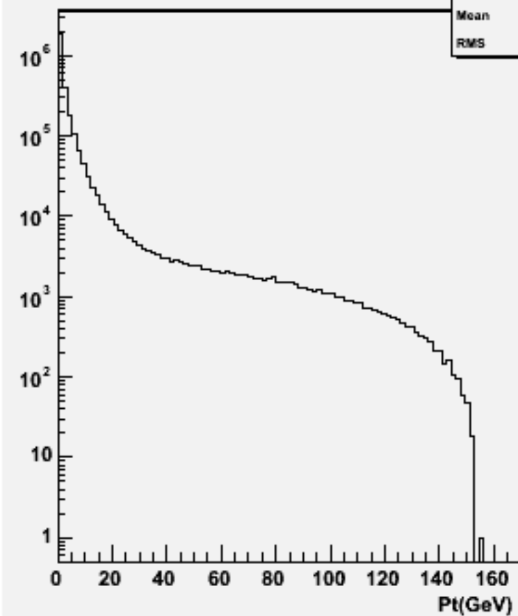
Particle Pt : w100356 e2e2h_o
