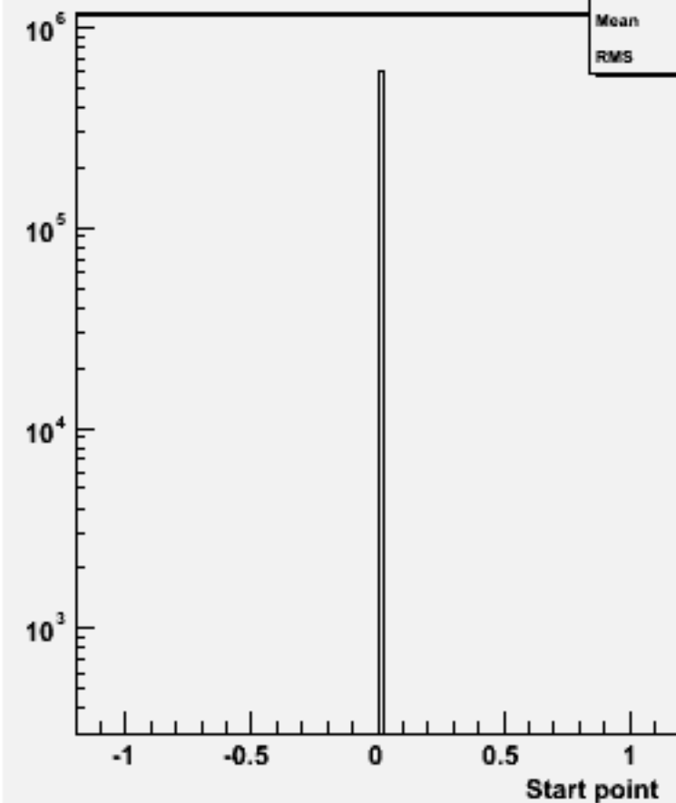
Start point Z : p105013 bbe1n1e3n3_p
