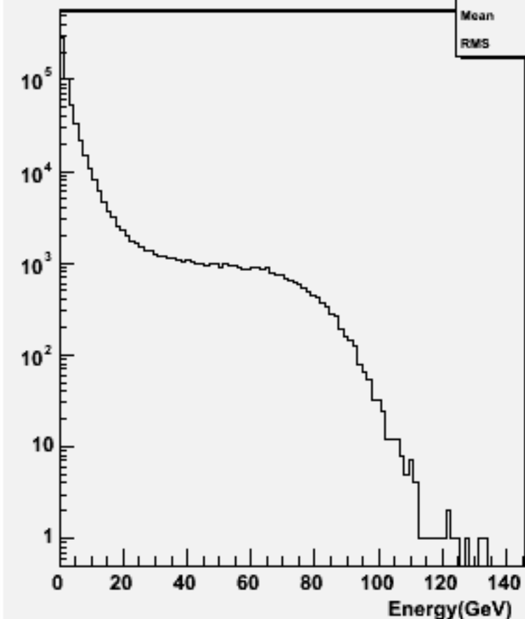
Start point R : p105013 bbe1n1e3n3_p
