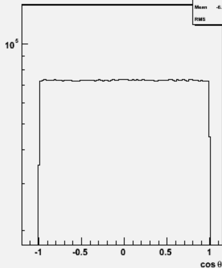
Particle cos \theta : p105007 bbe3n3qq_p
