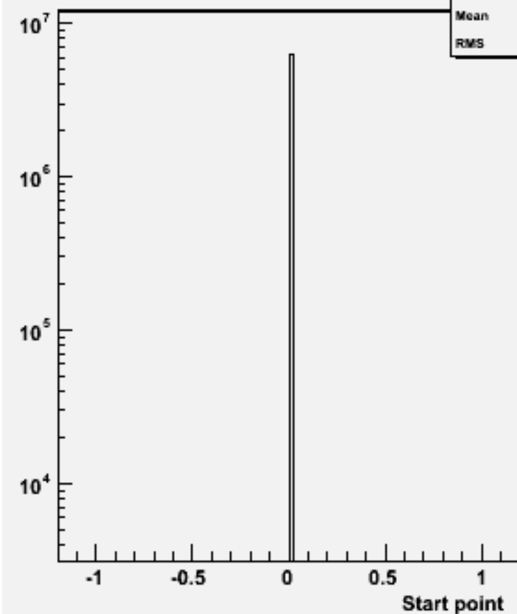
Start point Z : p105007 bbe3n3qq_p
