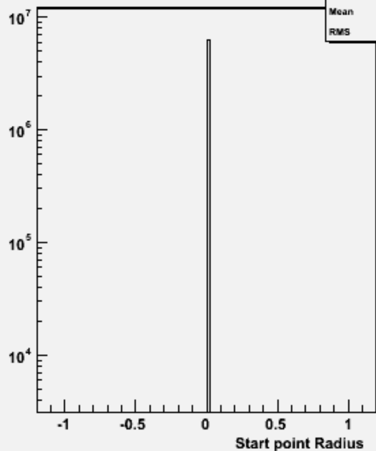
Start point R : p105007 bbe3n3qq_p
