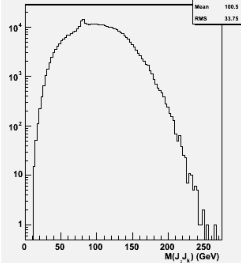
2jets mass(All comb)p105007 bbe3n3qq_p
