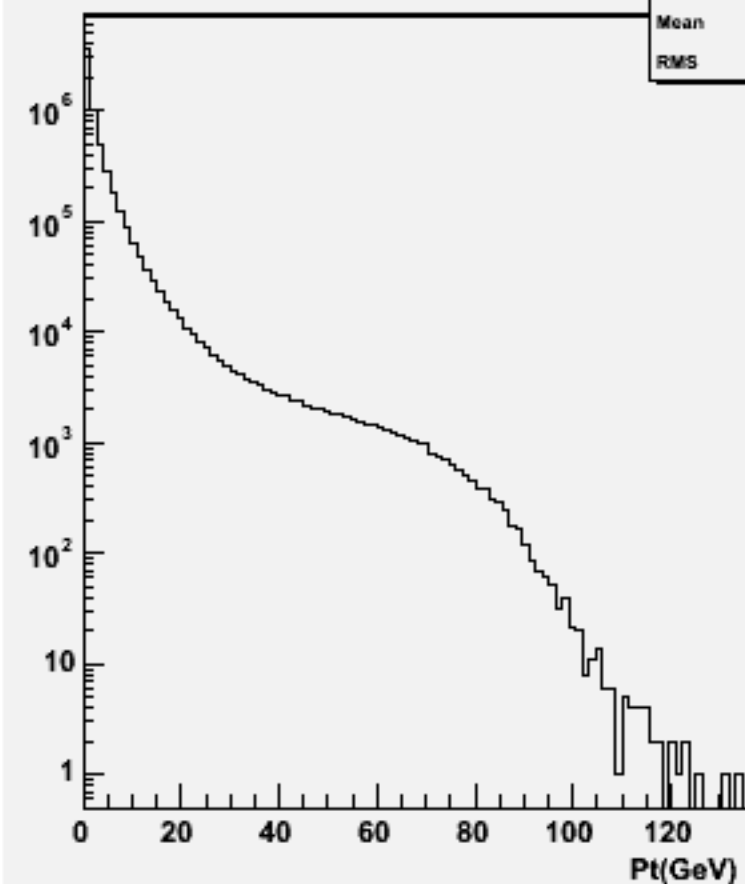
Particle Pt : p105007 bbe3n3qq_p
