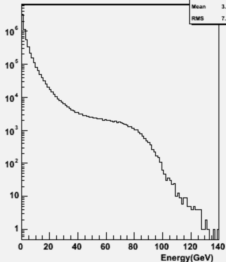
Particle Energy : p105007 bbe3n3qq_p
