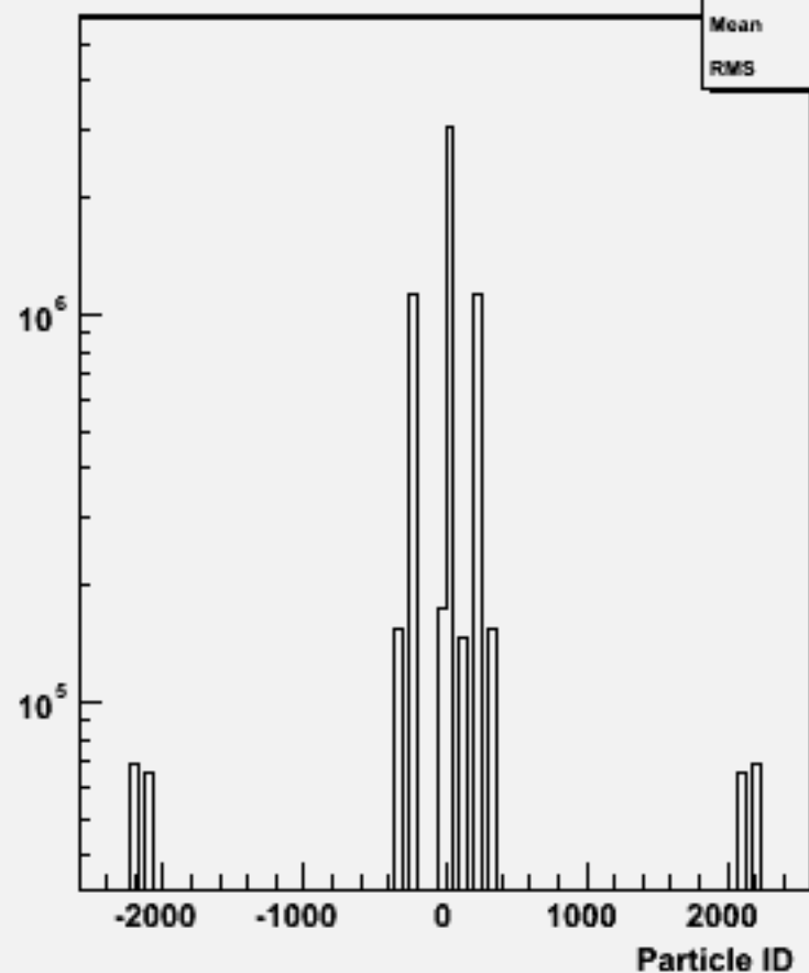
Particle ID : p105007 bbe3n3qq_p
