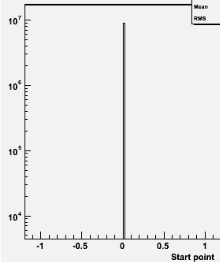
Start point Z : p105006 bbe3n3qq_p
