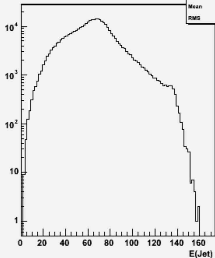
Jet energies(All jets)p105006 bbe3n3qq_p
