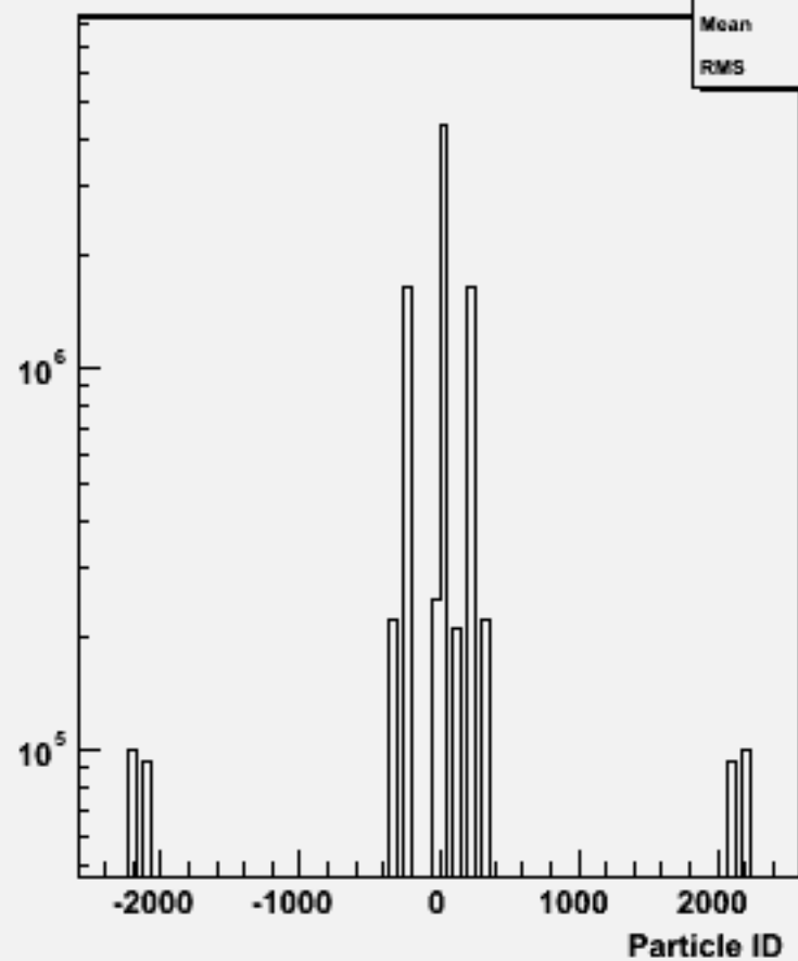
Particle ID : p105006 bbe3n3qq_p
