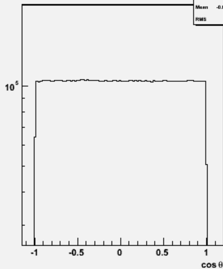
Particle cos \theta : p105006 bbe3n3qq_p
