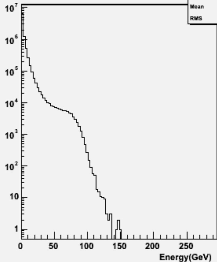
Particle Energy : p105006 bbe3n3qq_p
