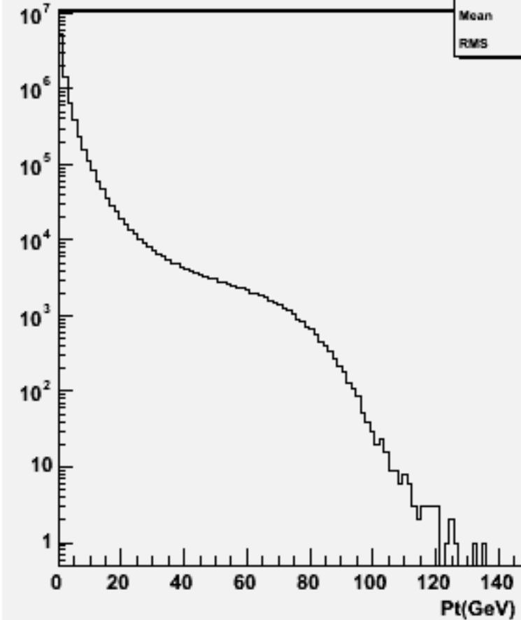
Particle Pt : p105006 bbe3n3qq_p
