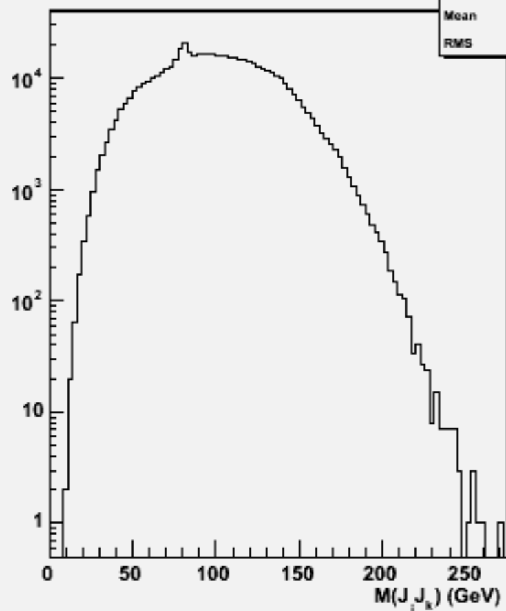
2jets mass(All comb)p105006 bbe3n3qq_p
