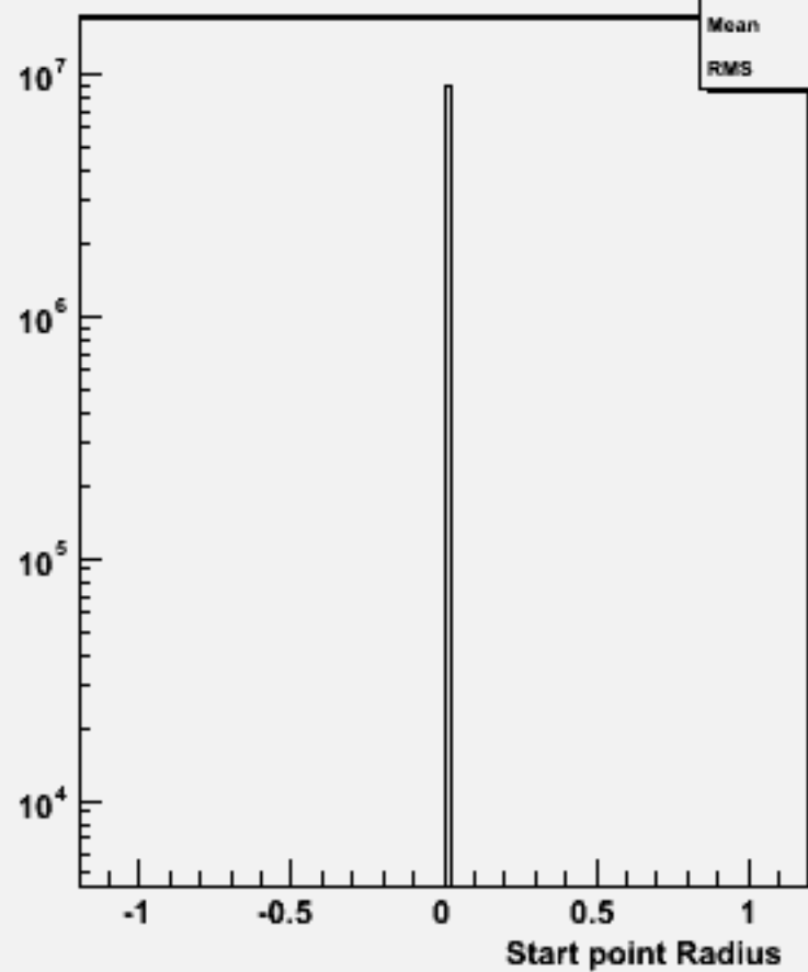
Start point R : p105006 bbe3n3qq_p
