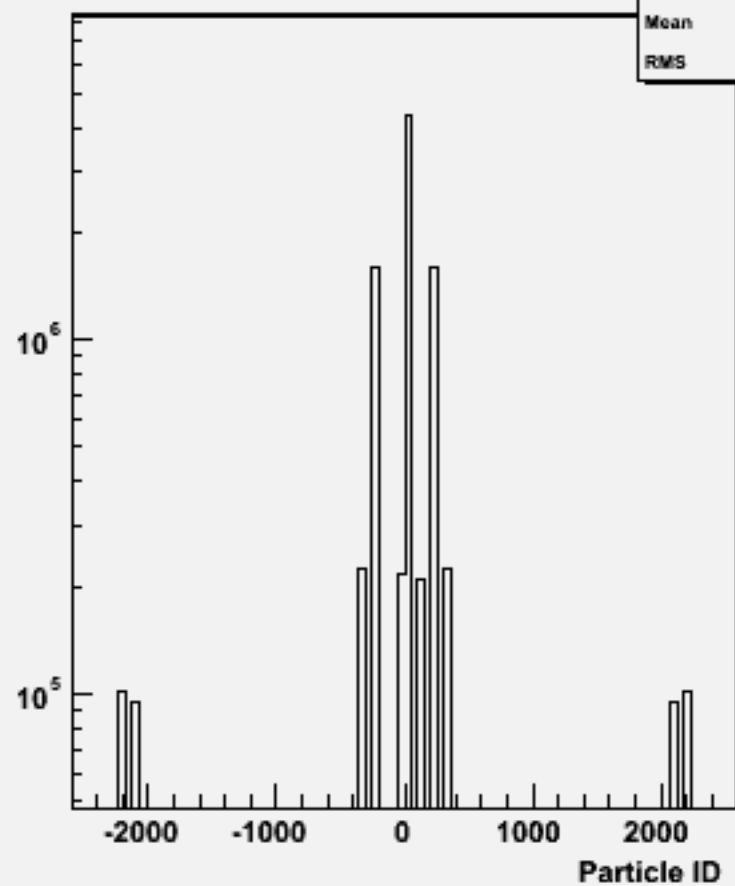
Particle ID : p105002 bbe1n1qq_p
