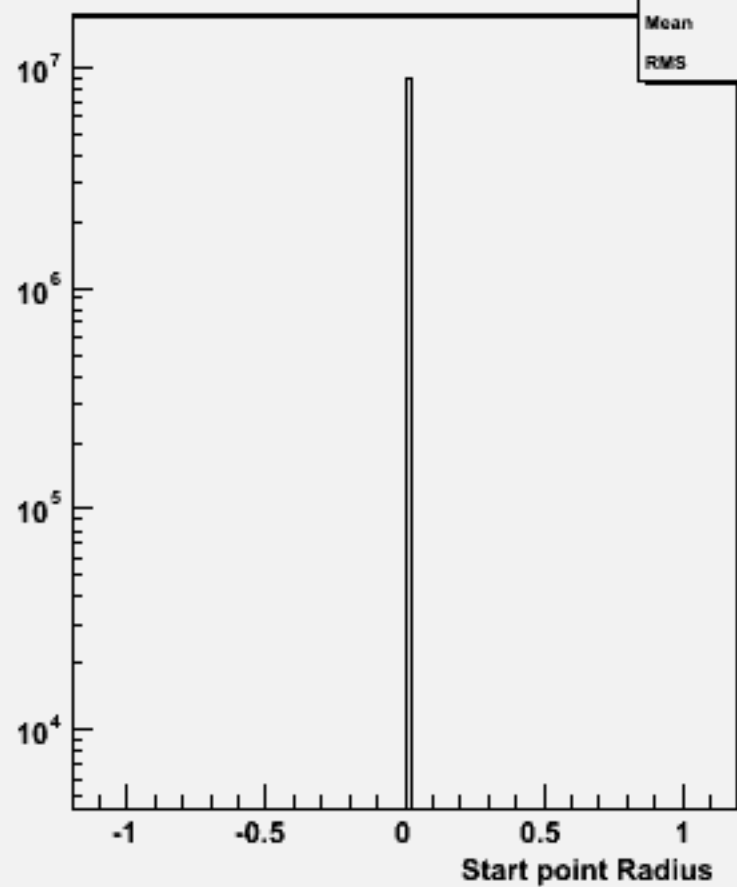
Start point R : p105002 bbe1n1qq_p
