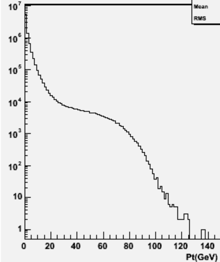
Particle Pt : p105002 bbe1n1qq_p
