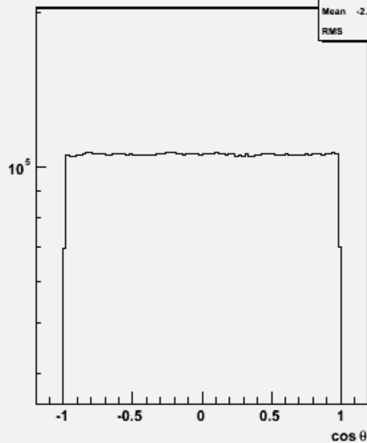
Particle cos \theta : p105002 bbe1n1qq_p
