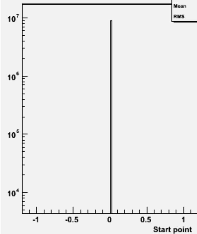
Start point Z : p105002 bbe1n1qq_p
