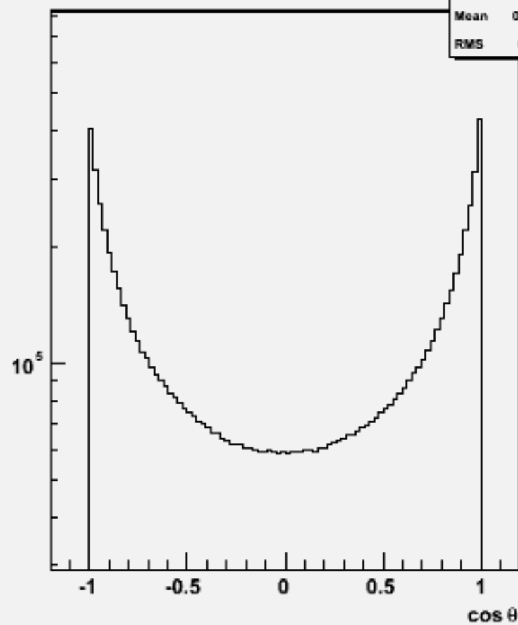
Particle cosθ : w104764 ss_o
