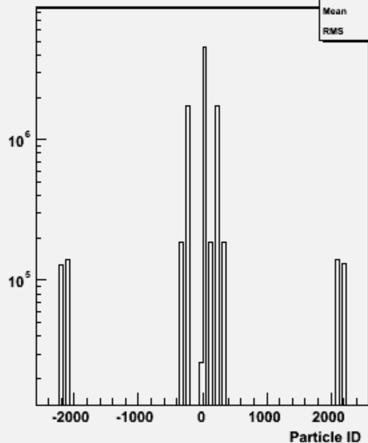
Particle ID : w104760 dd_o
