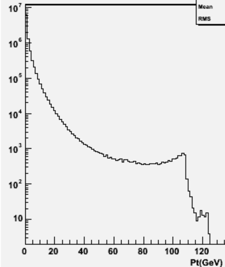
Particle Pt : w104760 dd_o
