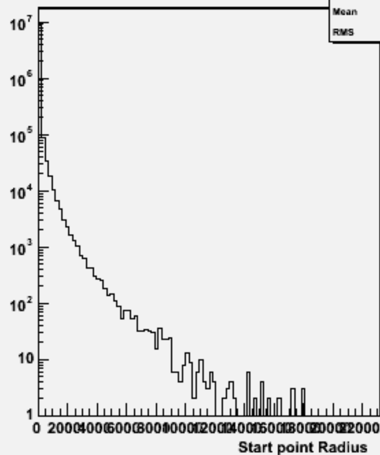
Start point R : w104760 dd_o
