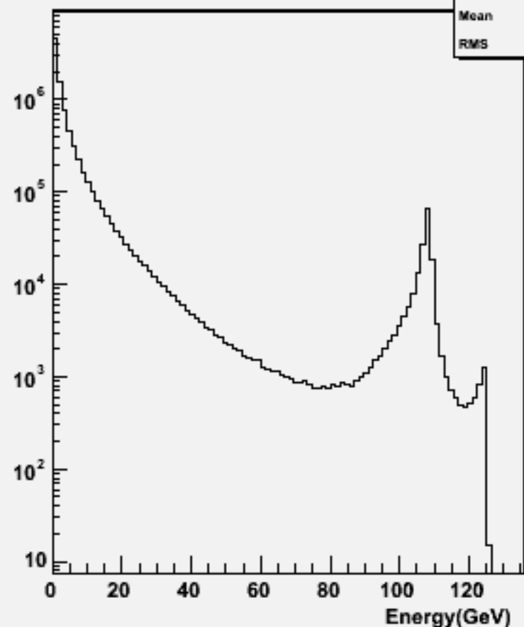
Particle Energy : w104760 dd_o
