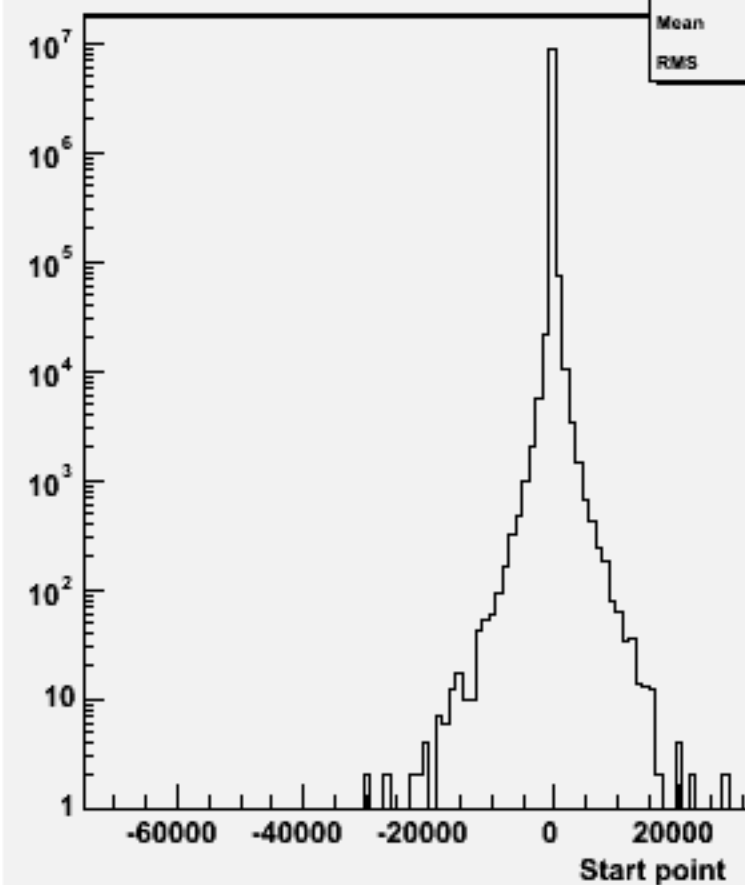
Start point Z : w104760 dd_o
