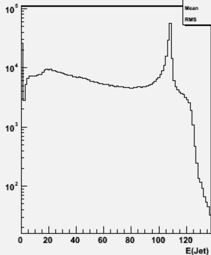
Jet energies(All jets)w104760 dd_o
