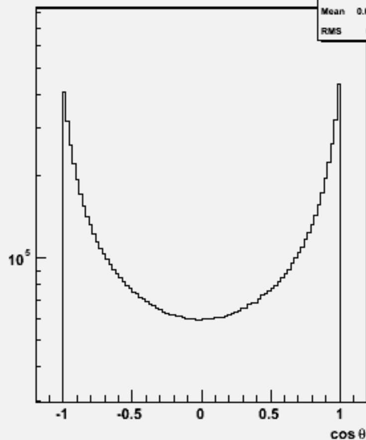
Particle cosθ : w104760 dd_o
