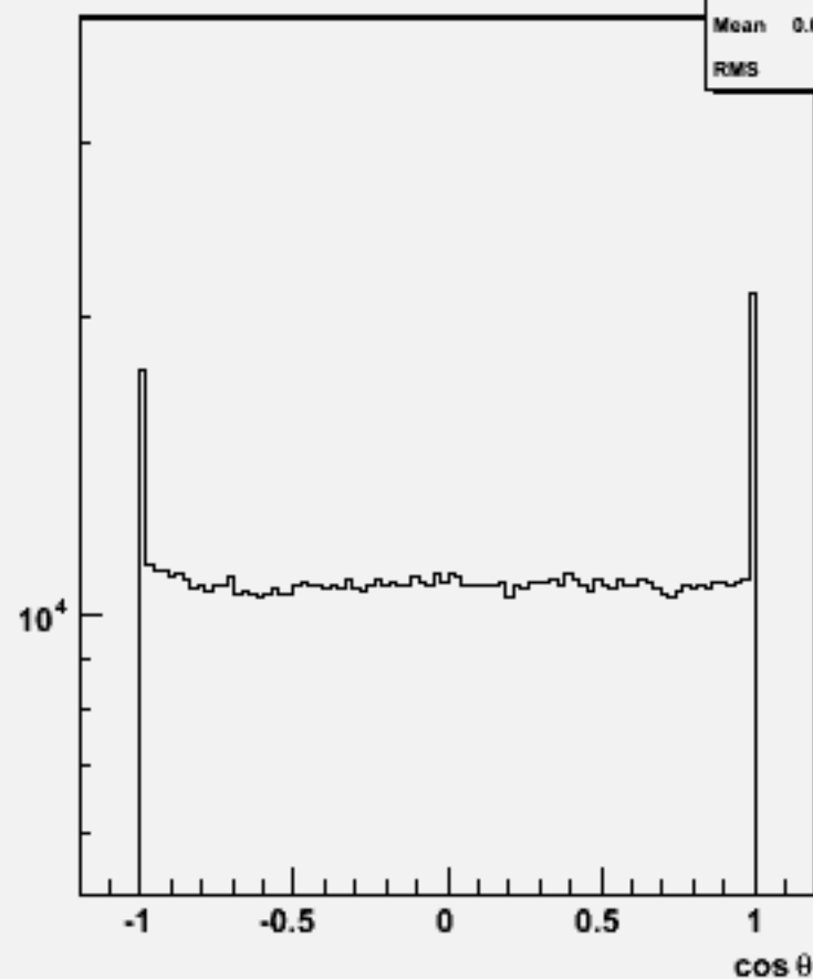
Particle cosθ : w104730 e3e3h_o
