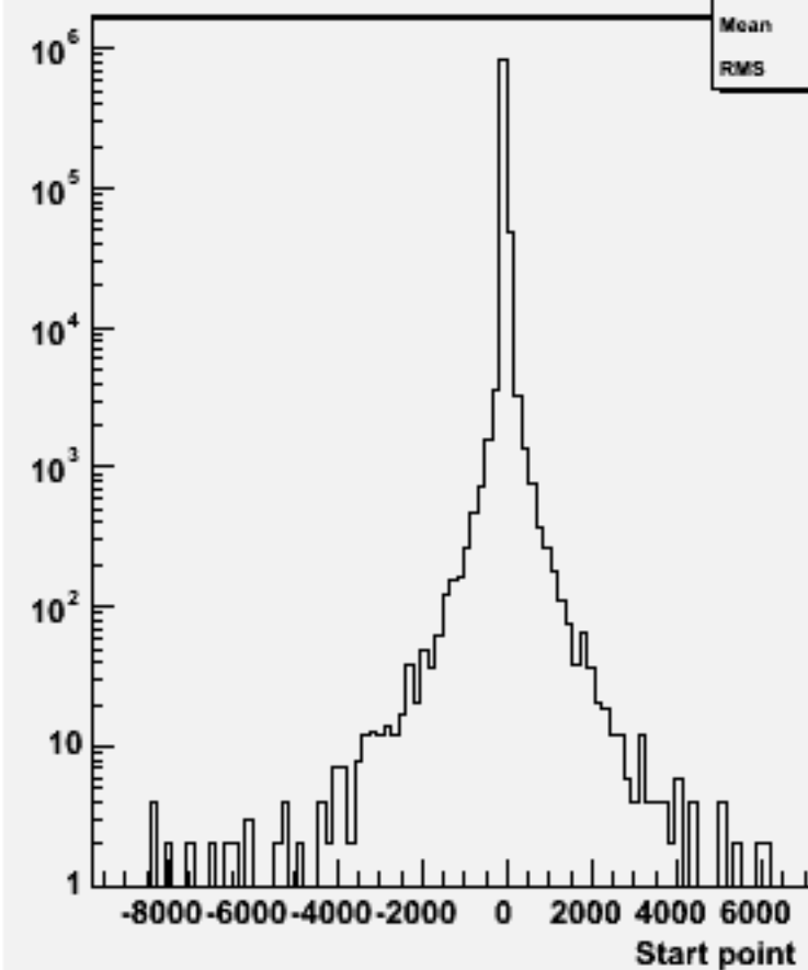
Start point Z : w104730 e3e3h_o
