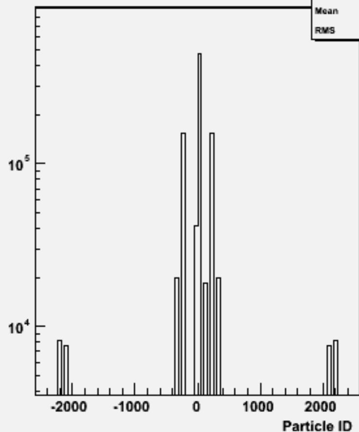
Particle ID : w104730 e3e3h_o
