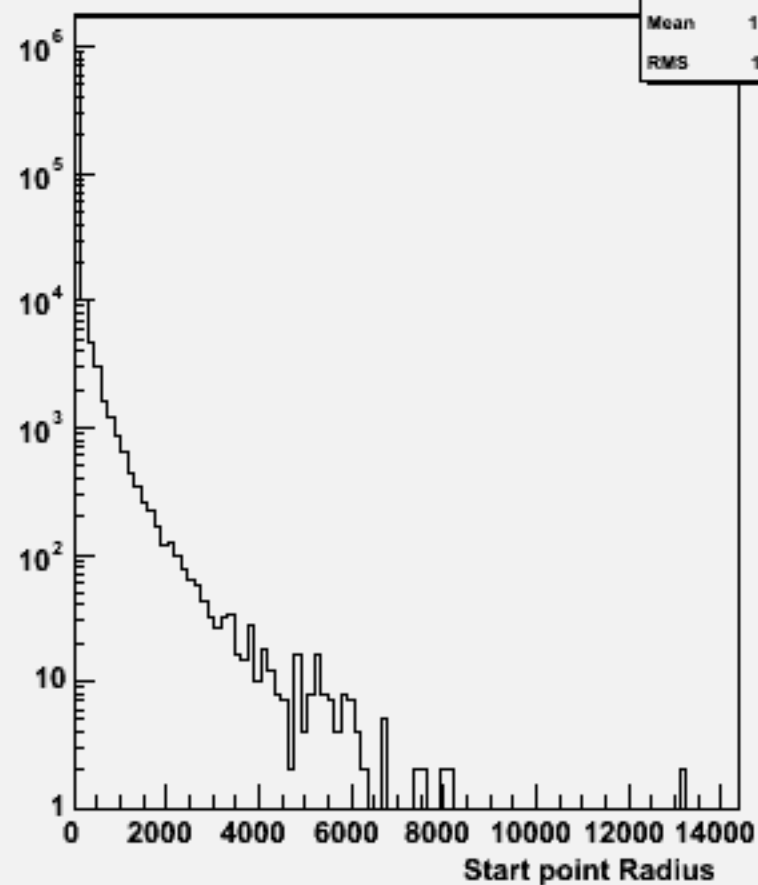
Start point R : w104730 e3e3h_o
