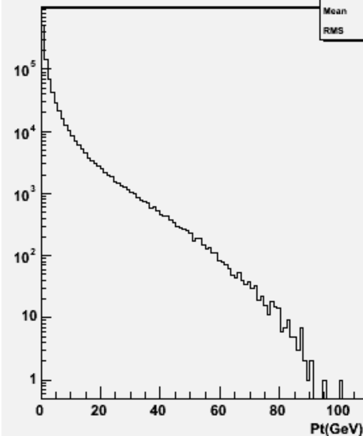
Particle Pt : w104730 e3e3h_o
