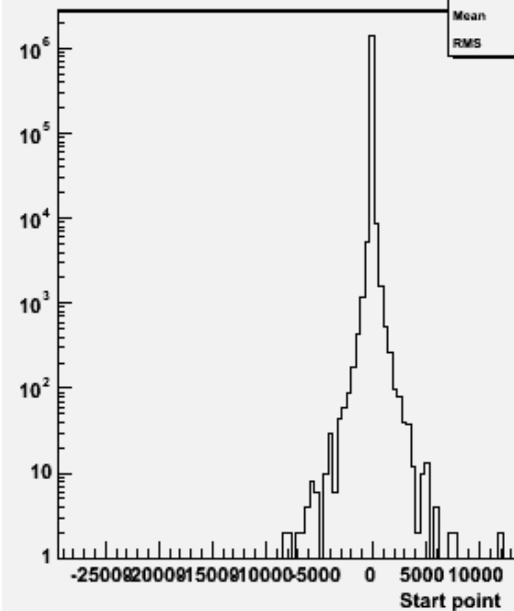
Start point Z : w104729 e3e3h_o
