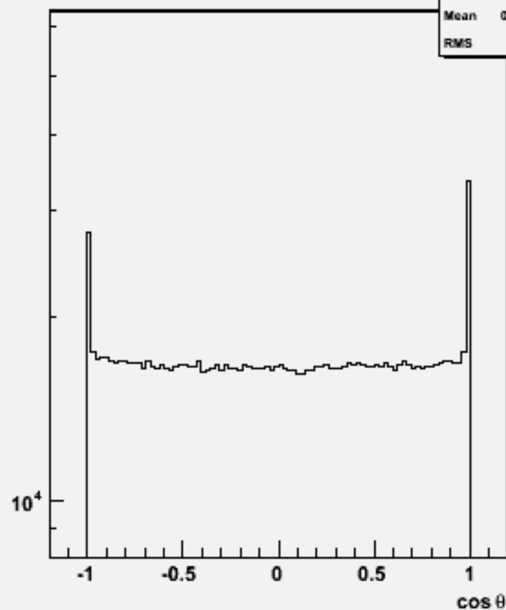
Particle cosθ : w104729 e3e3h_o
