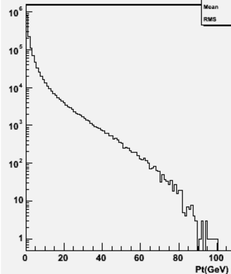
Particle Pt : w104729 e3e3h_o
