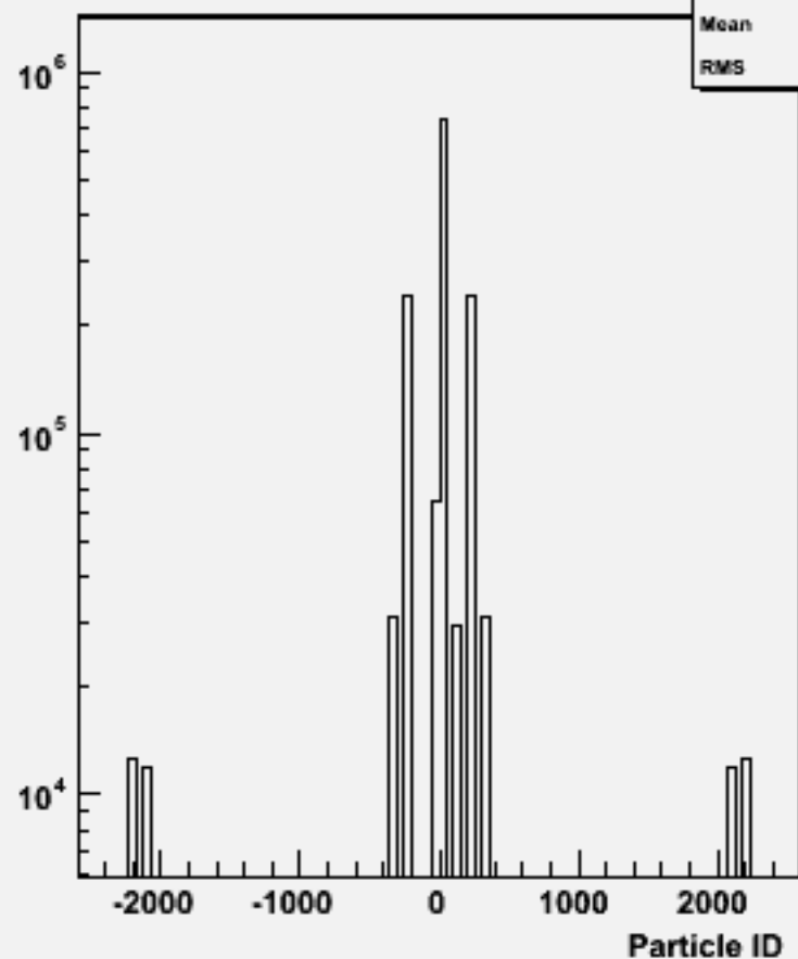
Particle ID : w104729 e3e3h_o
