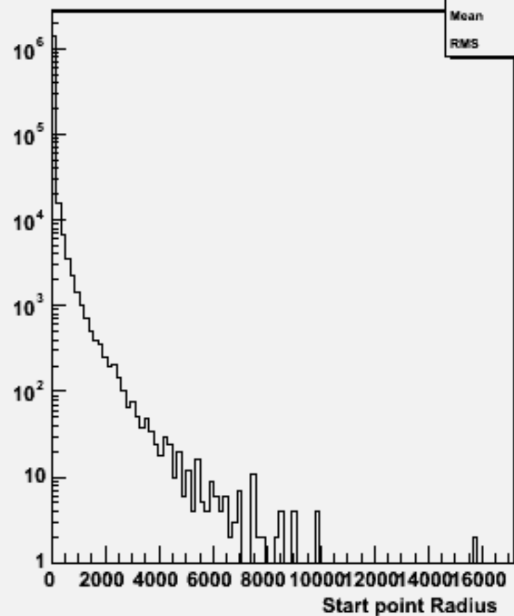
Start point R : w104729 e3e3h_o
