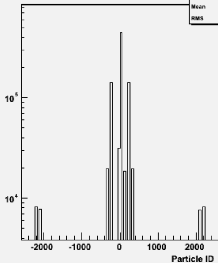
Particle ID : w104726 e2e2h_o
