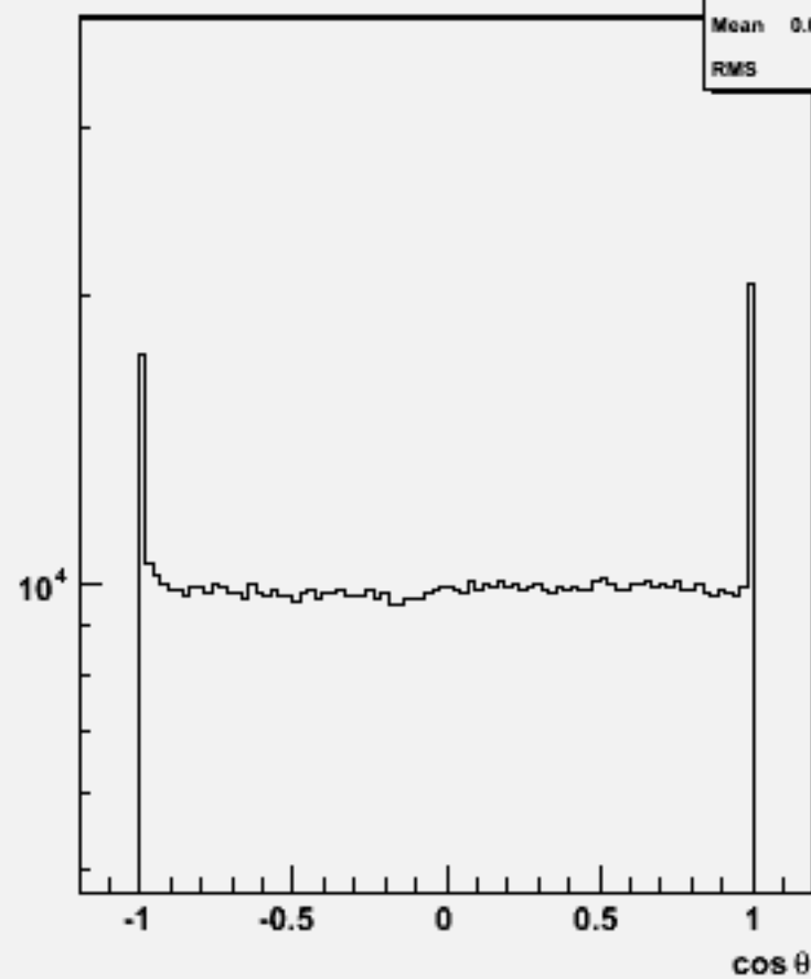
Particle cos \theta : w104726 e2e2h_o
