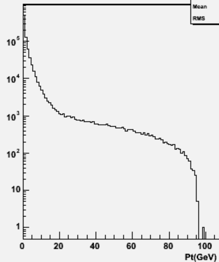
Particle Pt : w104726 e2e2h_o
