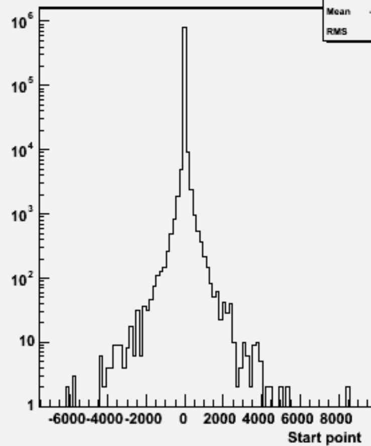
Start point Z : w104726 e2e2h_o
