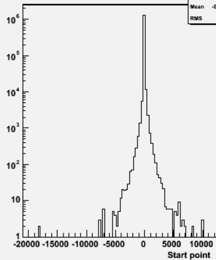
Start point Z : w104725 e2e2h_o
