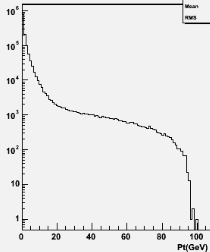
Particle Pt : w104725 e2e2h_o
