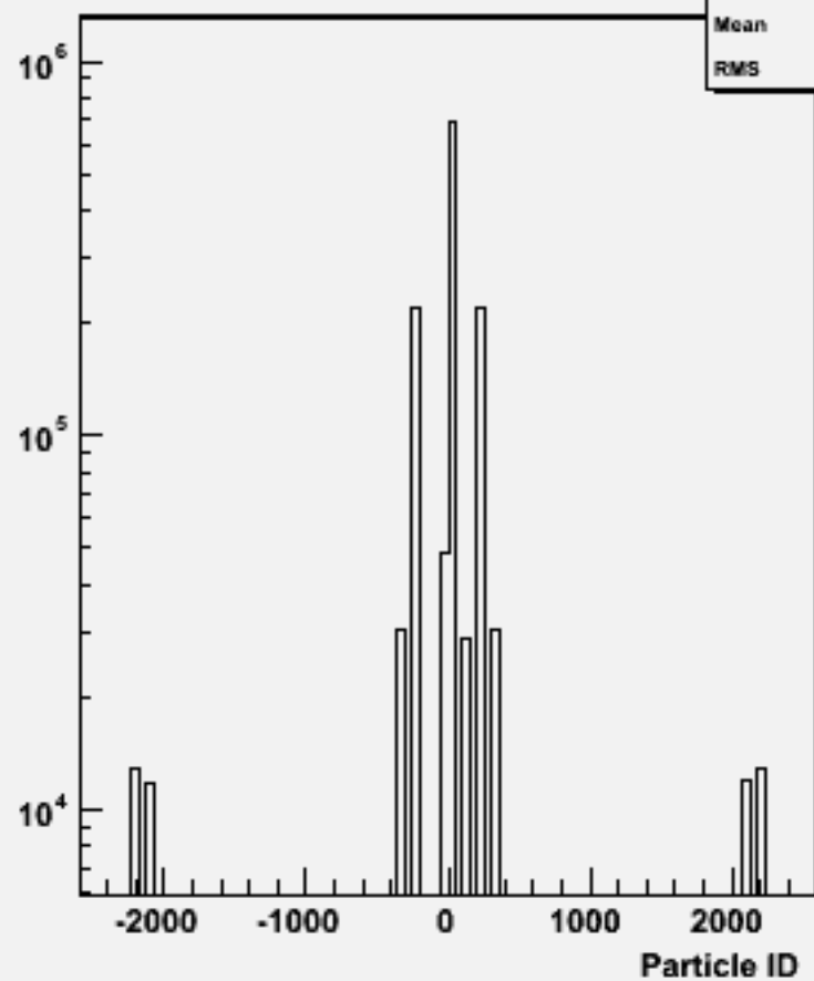
Particle ID : w104725 e2e2h_o
