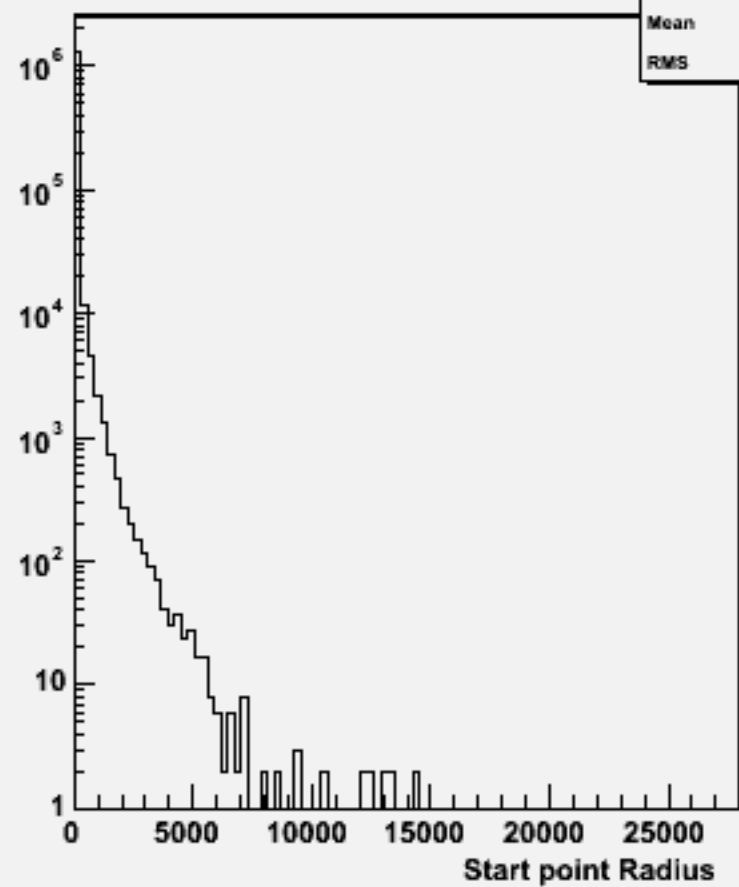
Start point R : w104725 e2e2h_o
