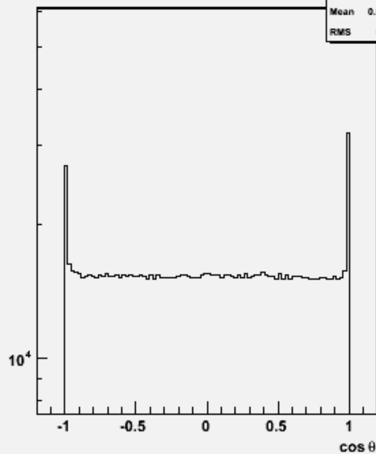
Particle cos \theta : w104725 e2e2h_o
