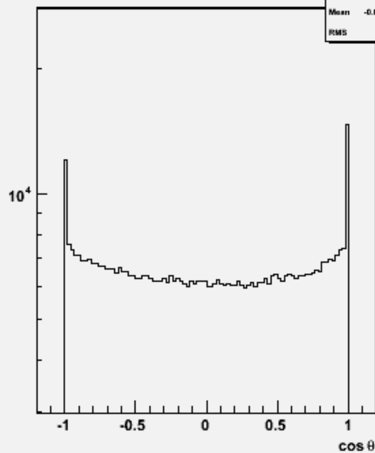
Particle cosθ : w104723 e1e1h_o
