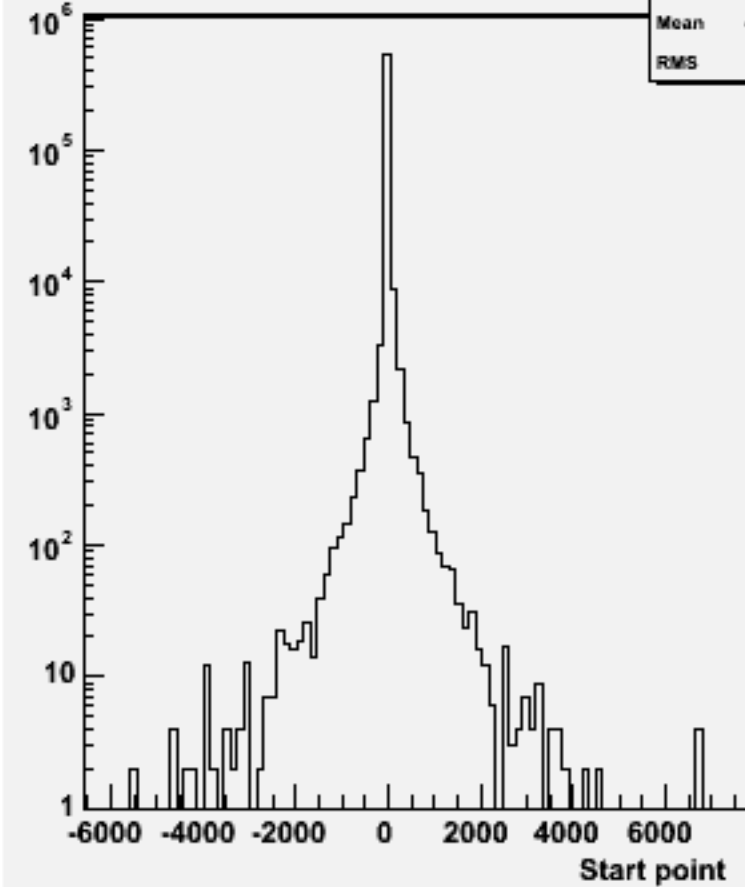
Start point Z : w104723 e1e1h_o
