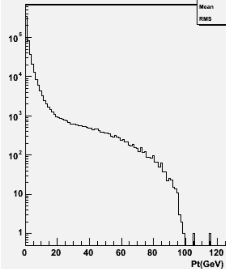
Particle Pt : w104723 e1e1h_o
