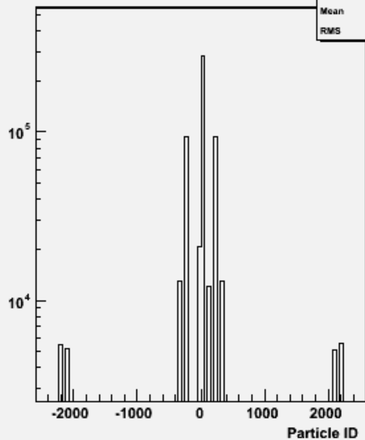
Particle ID : w104723 e1e1h_o
