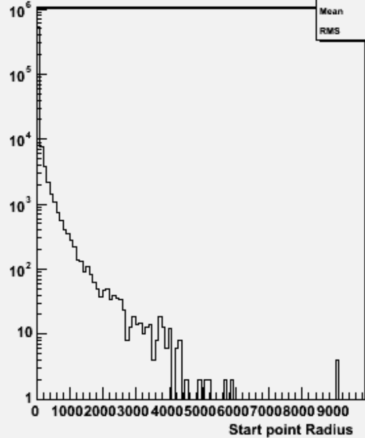
Start point R : w104723 e1e1h_o
