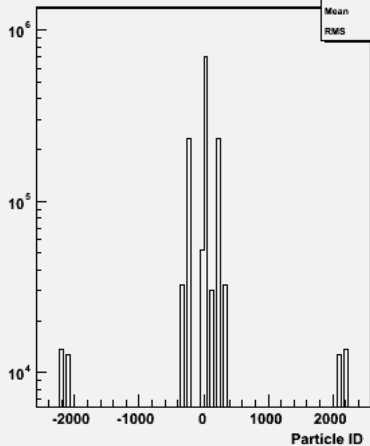
Particle ID : w104721 e1e1h_o
