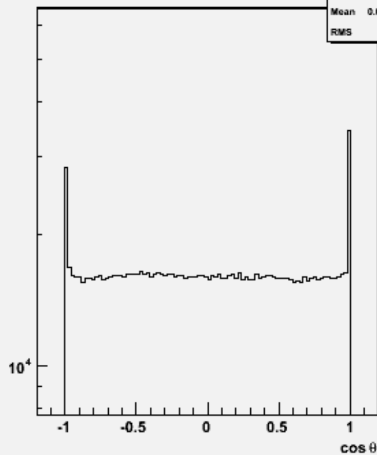
Particle cosθ : w104721 e1e1h_o
