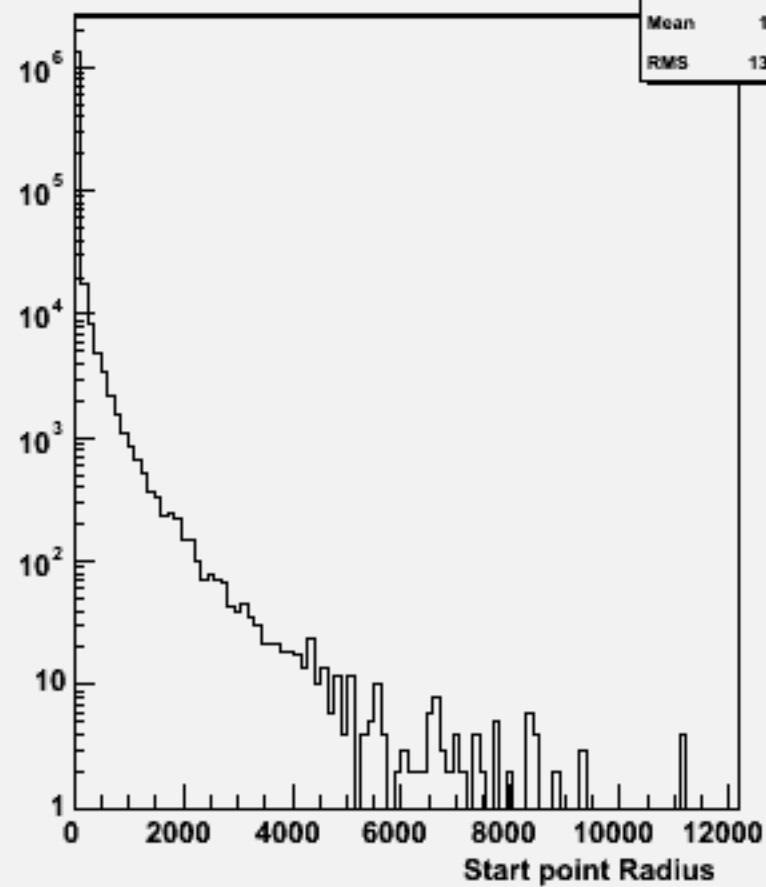
Start point R : w104721 e1e1h_o
