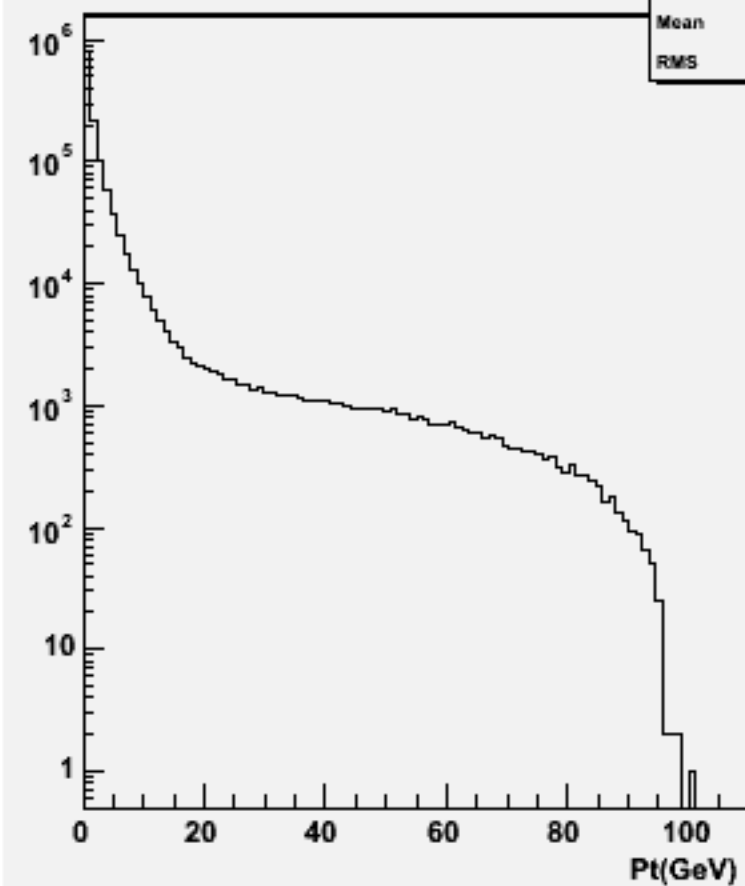
Particle Pt : w104721 e1e1h_o
