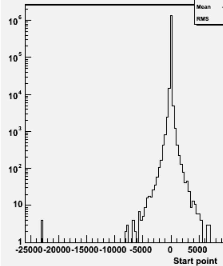
Start point Z : w104721 e1e1h_o
