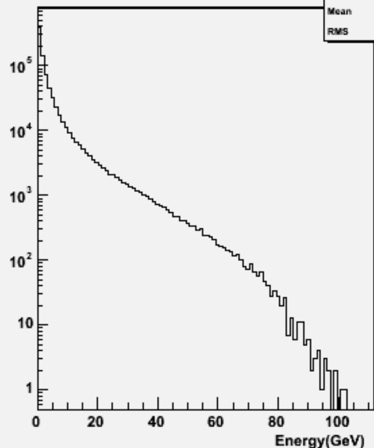
Particle Energy : w104680 e3e3h_o
