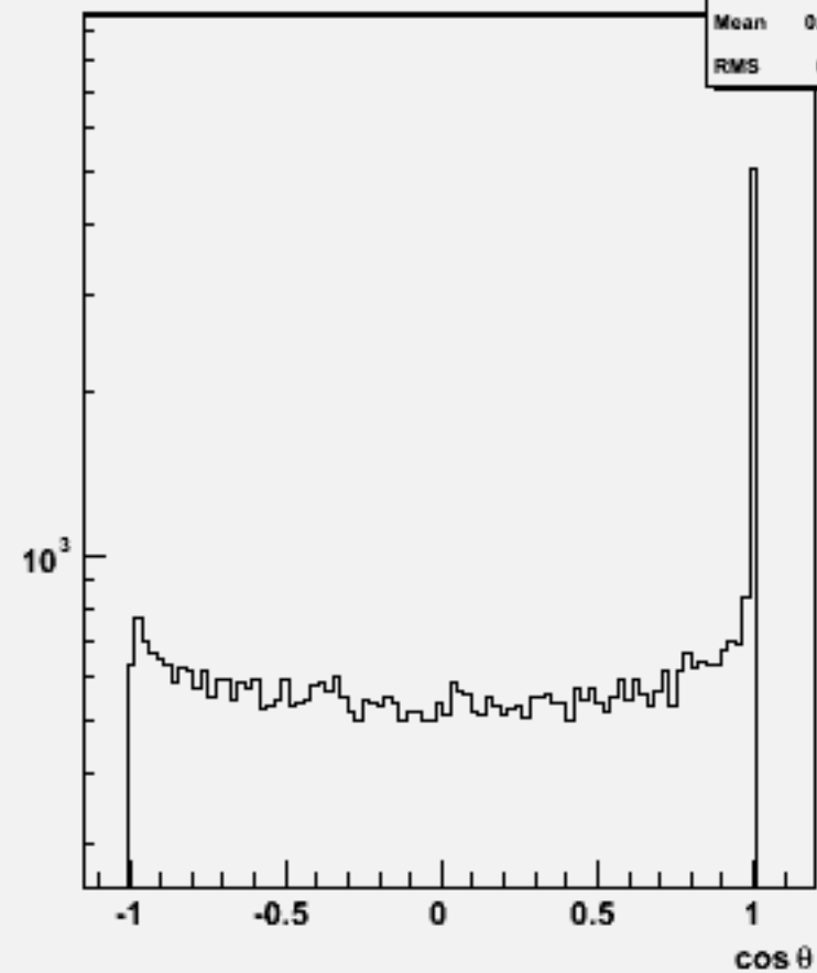
Jet cos \theta (All jets)w104680 e3e3h_o
