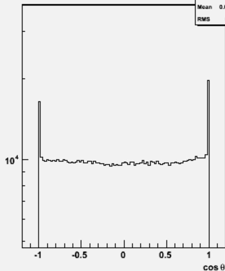
Particle cosθ : w104680 e3e3h_o
