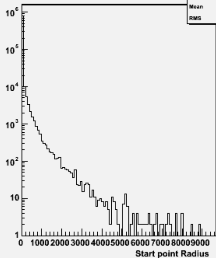
Start point R : w104680 e3e3h_o
