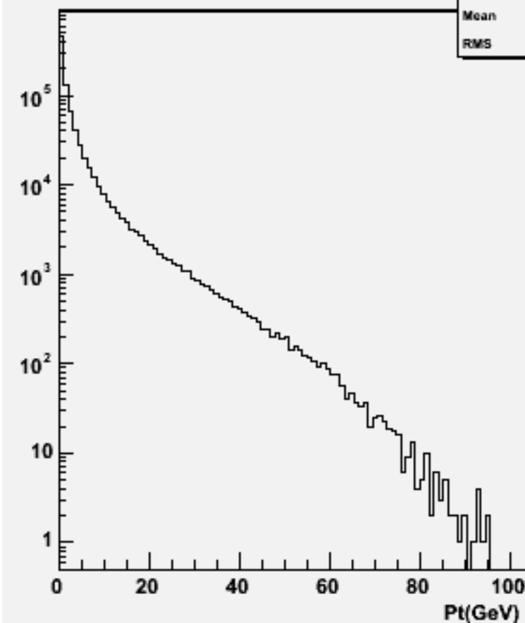
Particle Pt : w104680 e3e3h_o
