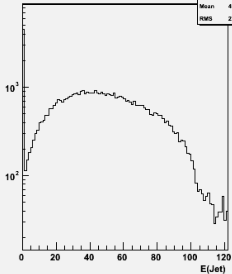
Jet energies(All jets)w104680 e3e3h_o
