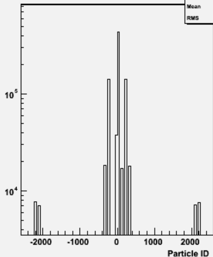
Particle ID : w104680 e3e3h_o
