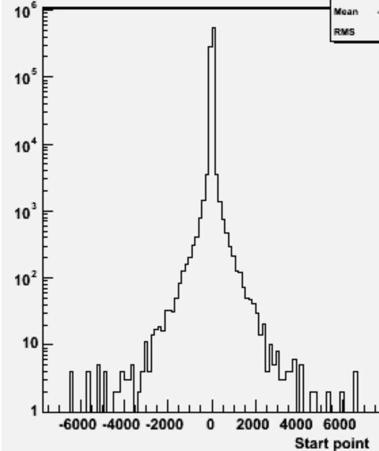
Start point Z : w104680 e3e3h_o
