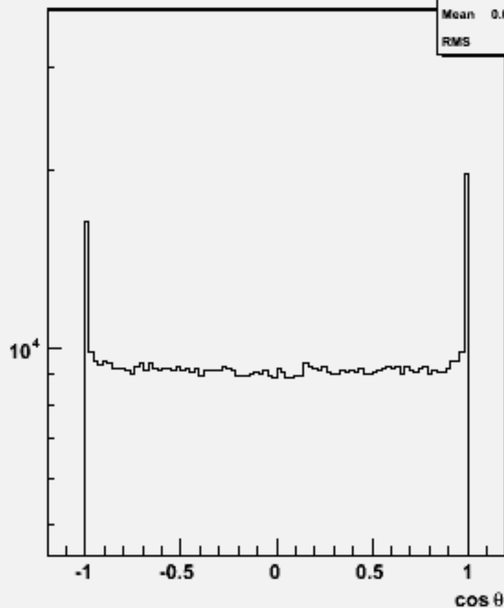
Particle cosθ : w104672 e1e1h_o
