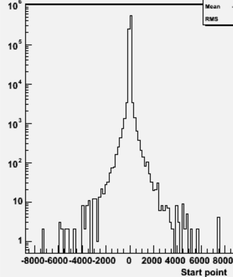
Start point Z : w104672 e1e1h_o
