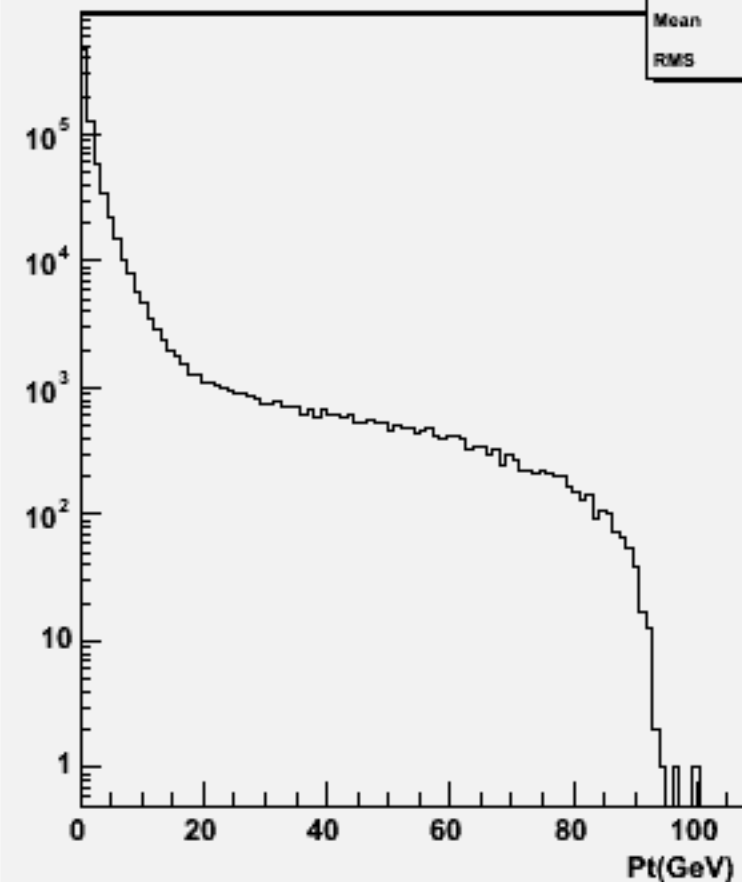
Particle Pt : w104672 e1e1h_o
