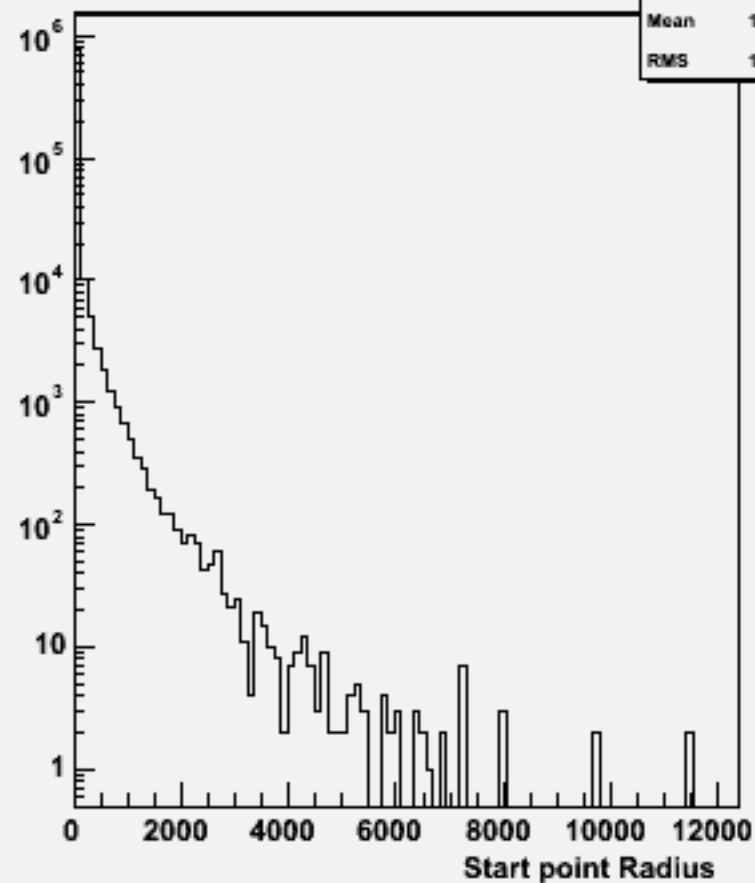
Start point R : w104672 e1e1h_o
