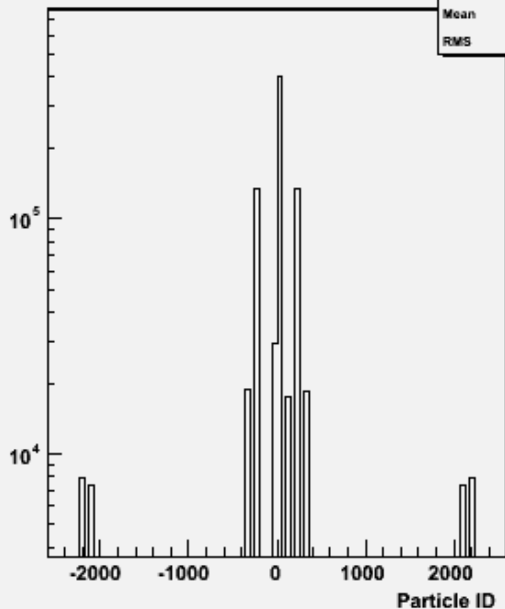
Particle ID : w104672 e1e1h_o
