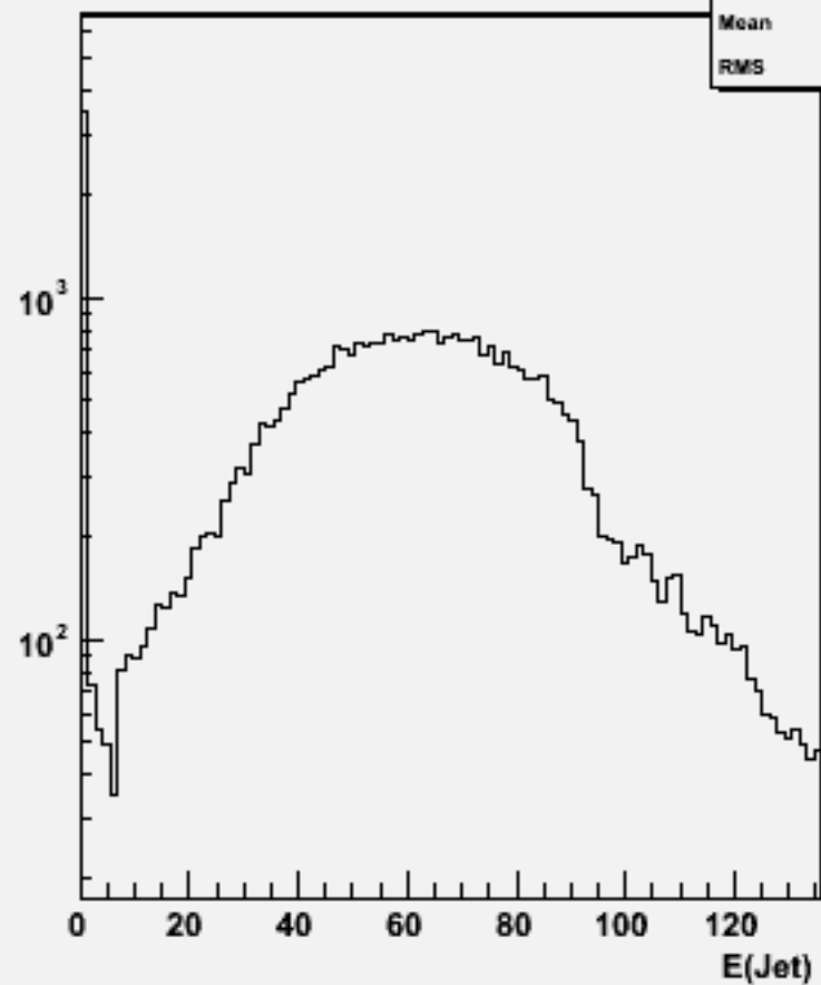
Jet energies(All jets)w104670 e1e1h_o
