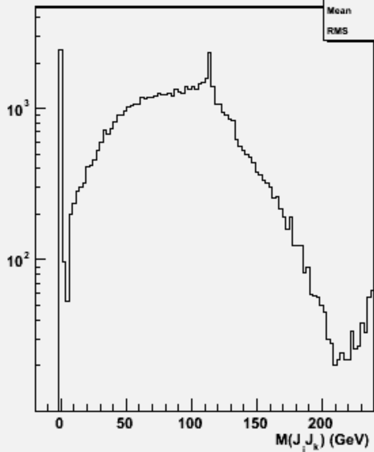
2jets mass(All comb)w104670 e1e1h_o
