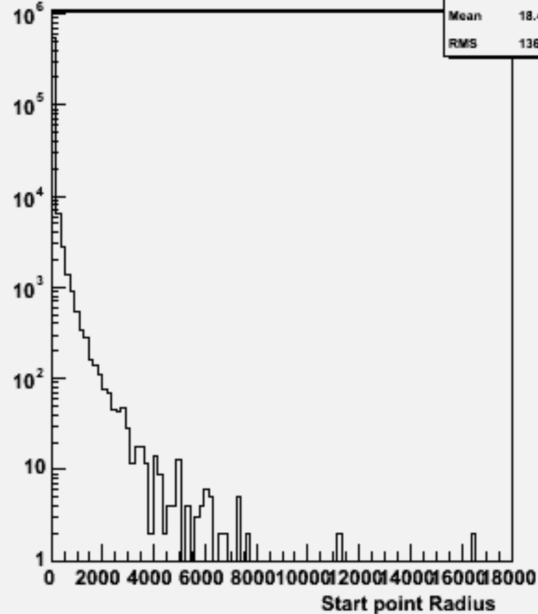
Start point R : w104670 e1e1h_o
