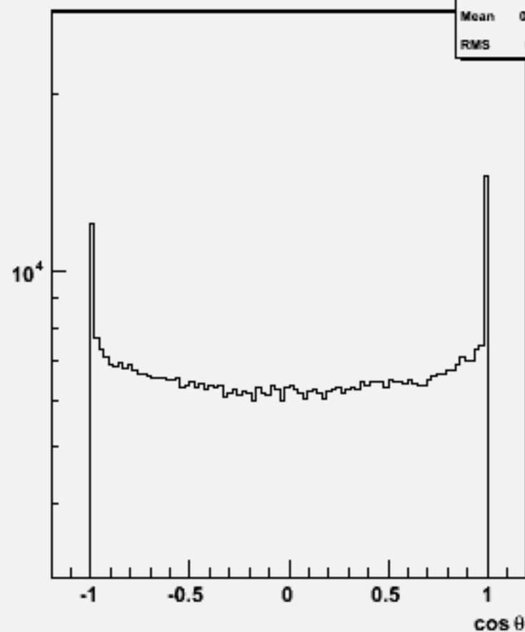
Particle cosθ : w104670 e1e1h_o
