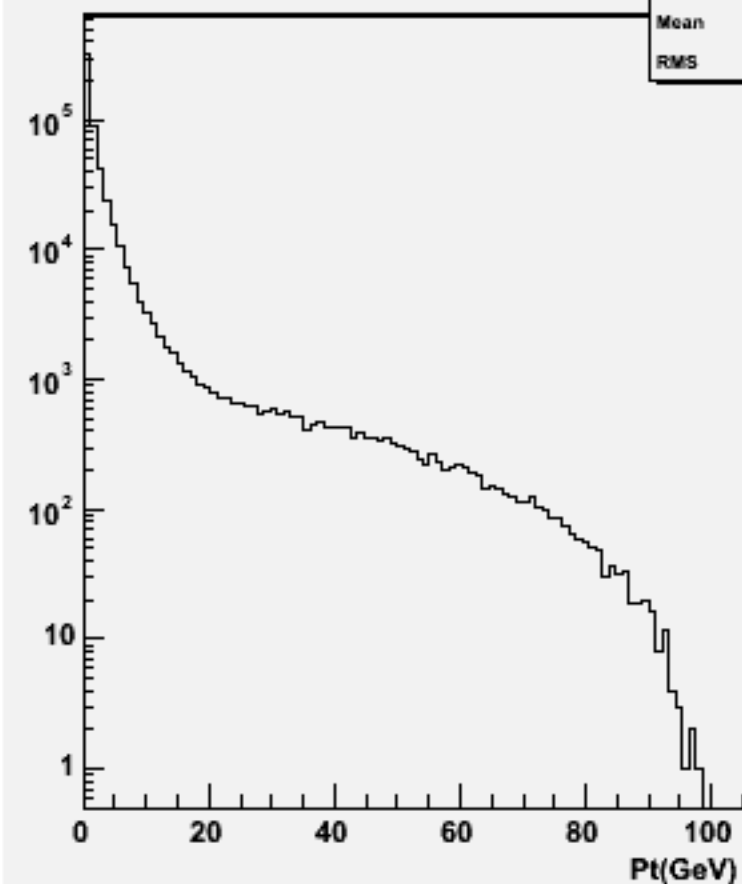
Particle Pt : w104670 e1e1h_o
