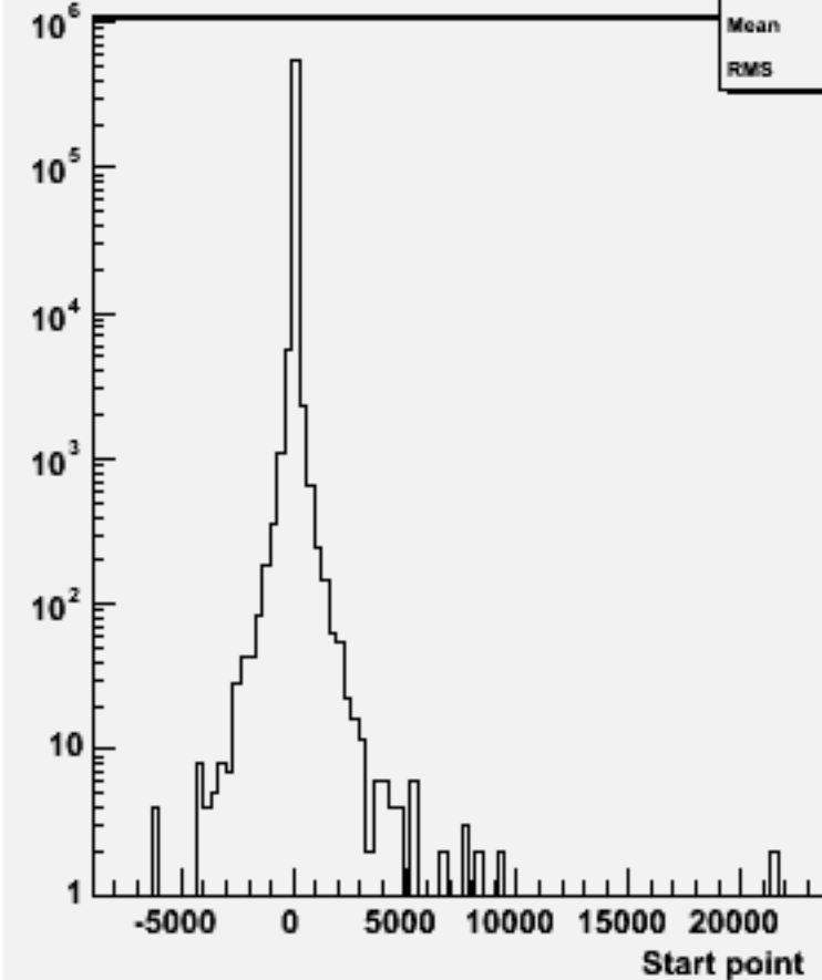
Start point Z : w104670 e1e1h_o
