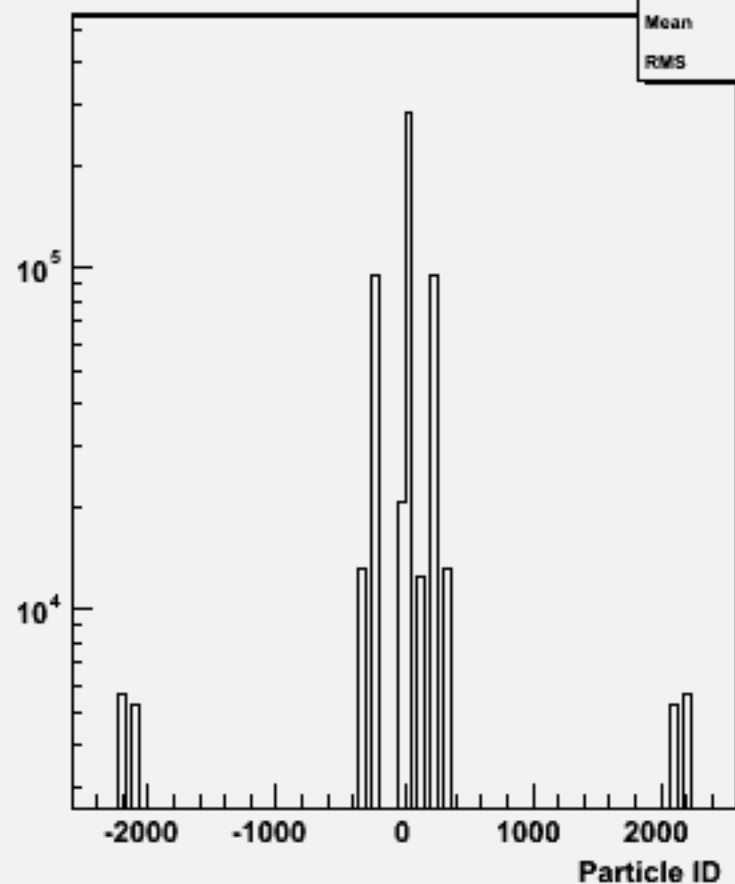
Particle ID : w104670 e1e1h_o
