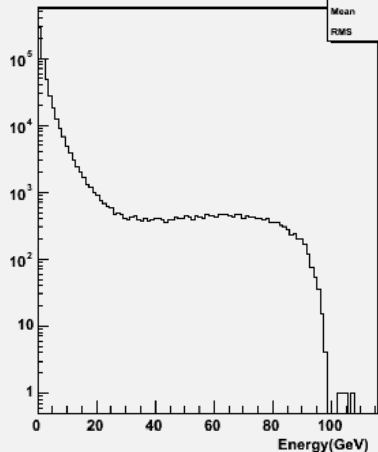
Particle Energy : w104670 e1e1h_o
