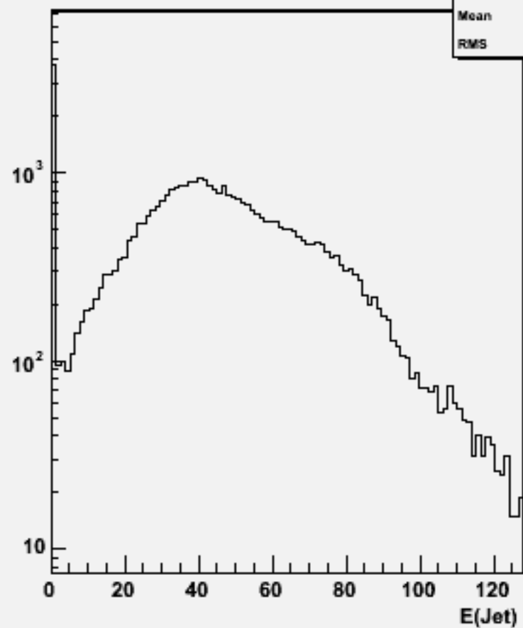
Jet energies(All jets)w104630 e3e3h_o
