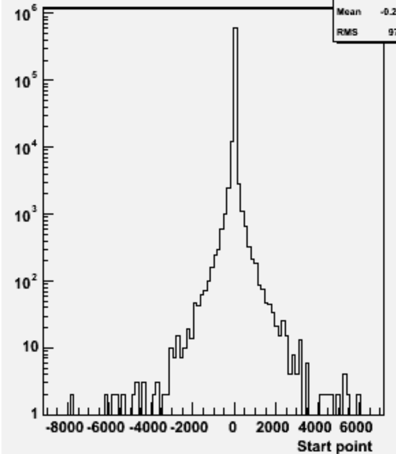
Start point Z : w104630 e3e3h_o
