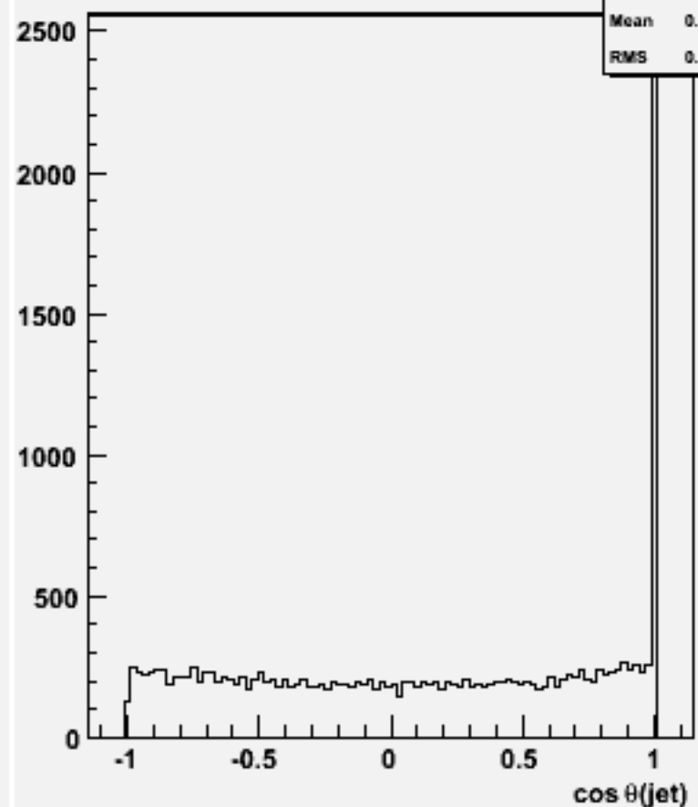
cos \theta for 2-jets :w104630 e3e3h_o
