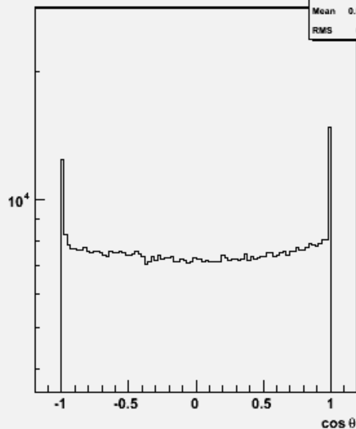
Particle cosθ : w104630 e3e3h_o
