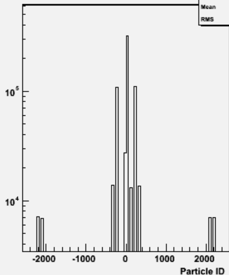
Particle ID : w104630 e3e3h_o
