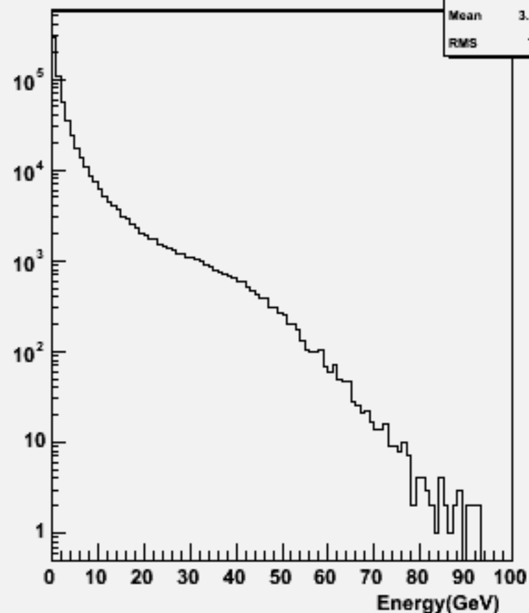
Particle Energy : w104630 e3e3h_o
