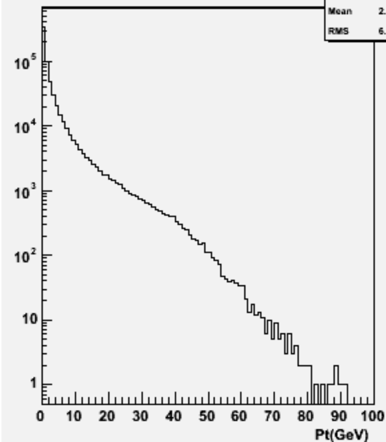
Particle Pt : w104630 e3e3h_o
