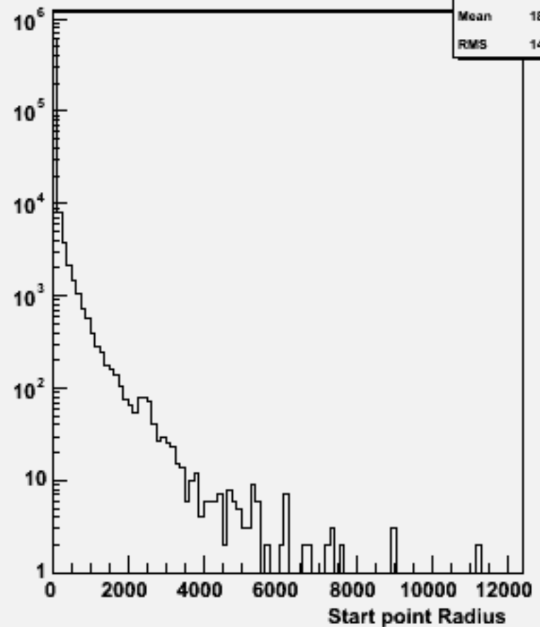
Start point R : w104630 e3e3h_o
