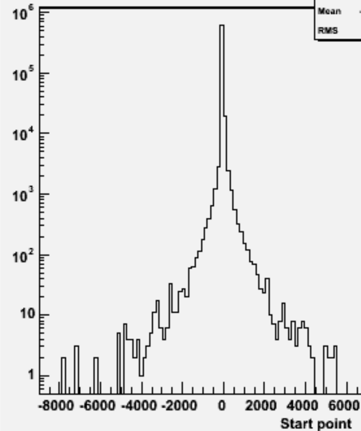
Start point Z : w104629 e3e3h_o
