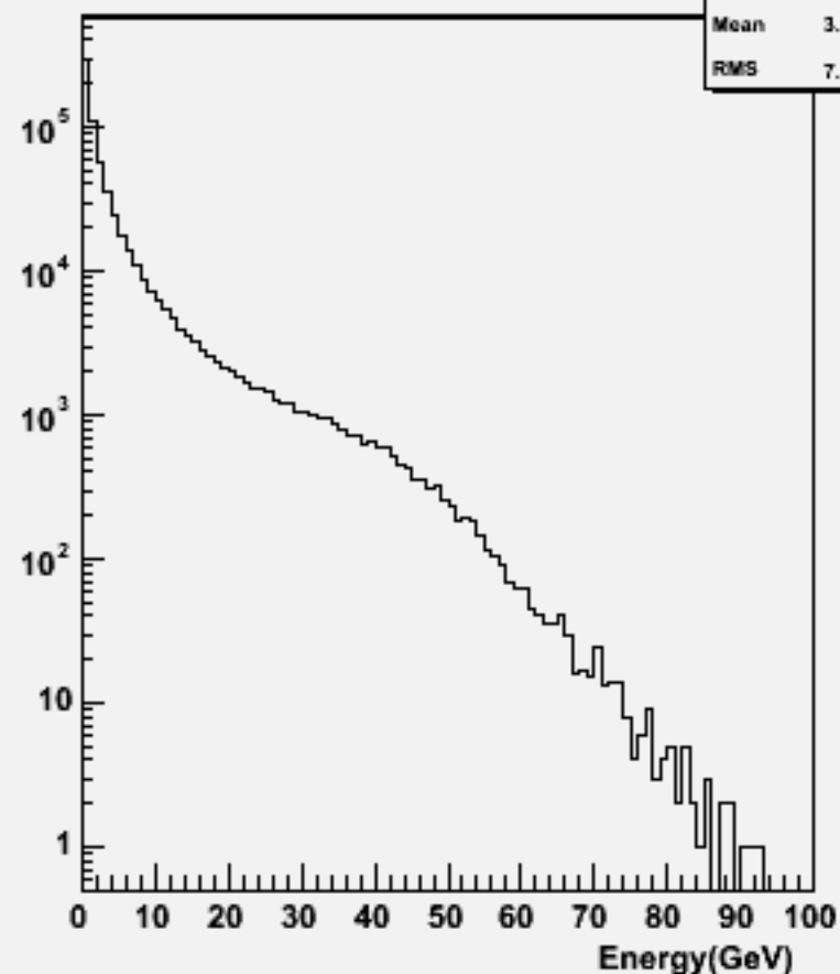
Particle Energy : w104629 e3e3h_o
