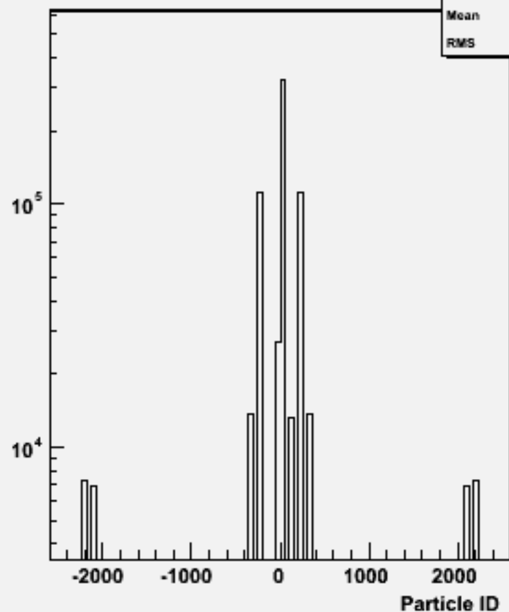
Particle ID : w104629 e3e3h_o
