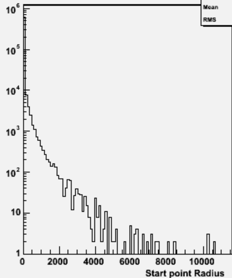
Start point R : w104629 e3e3h_o
