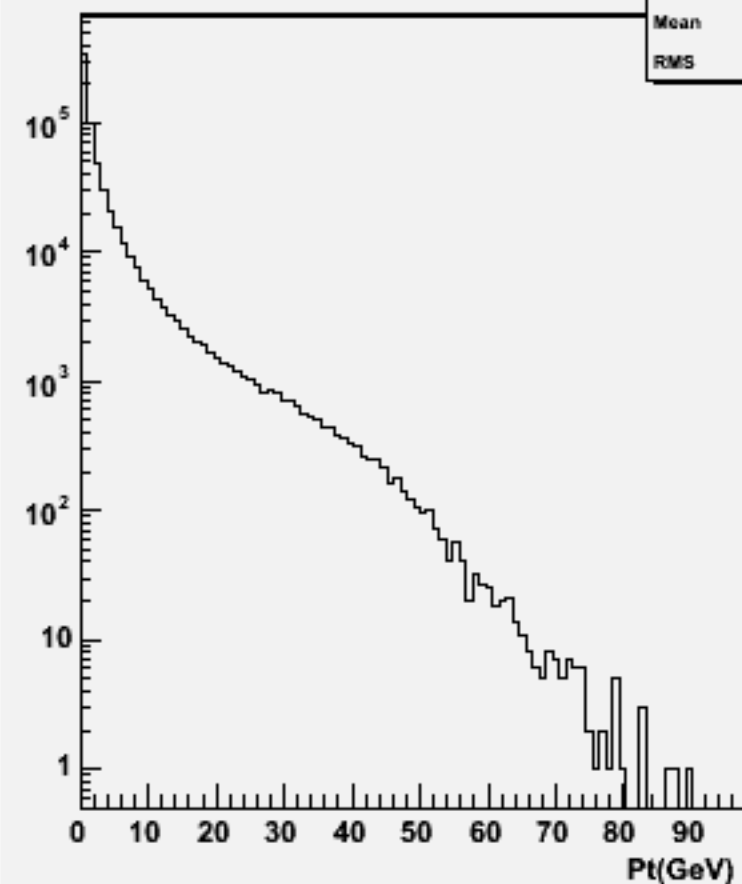
Particle Pt : w104629 e3e3h_o
