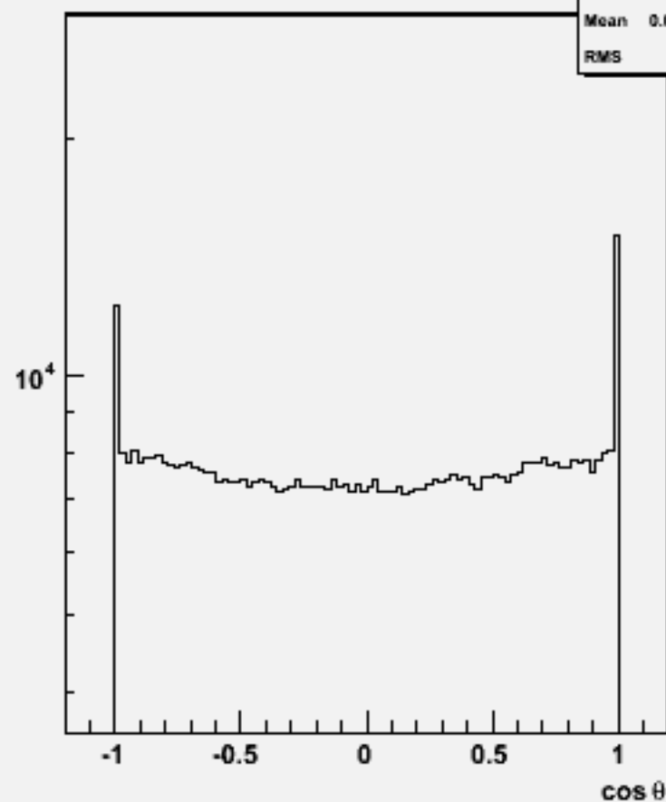
Particle cos \theta : w104629 e3e3h_o
