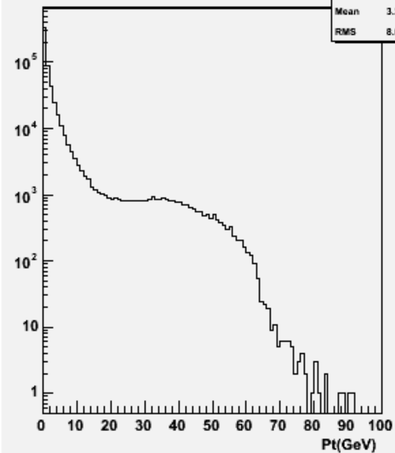
Particle Pt : w104626 e2e2h_o
