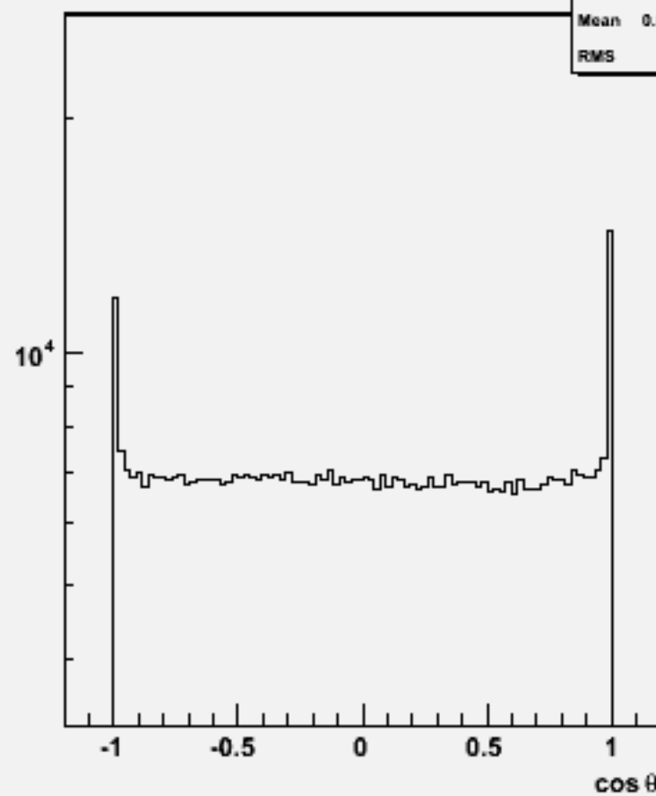
Particle cosθ : w104626 e2e2h_o
