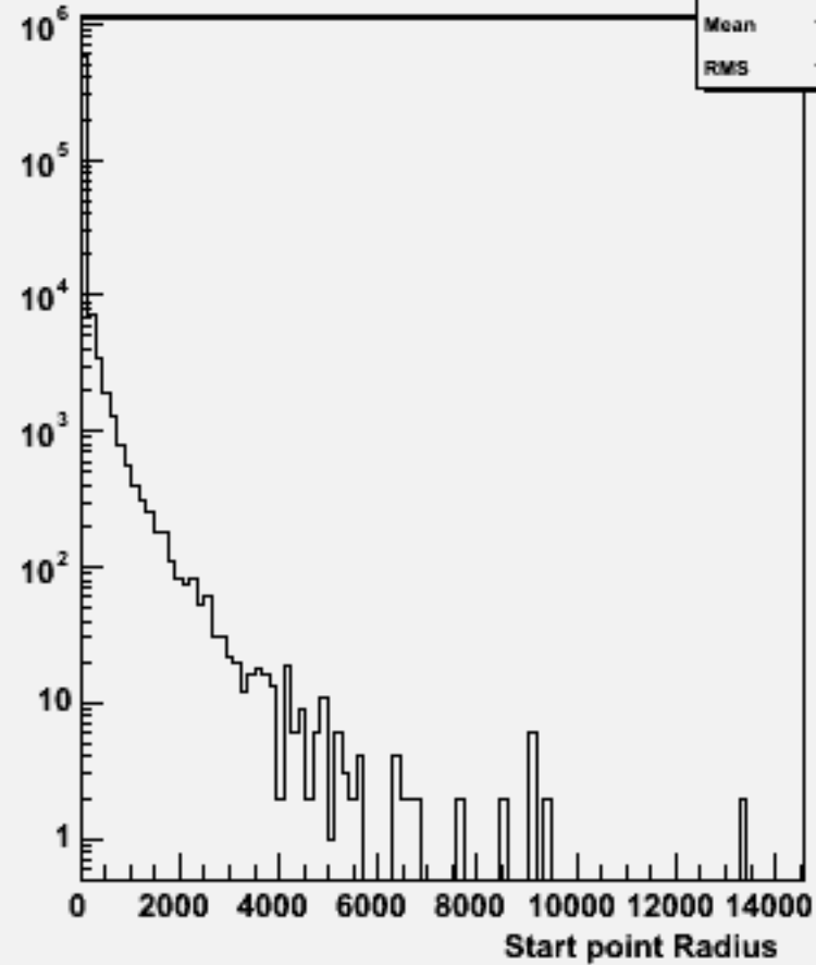
Start point R : w104626 e2e2h_o
