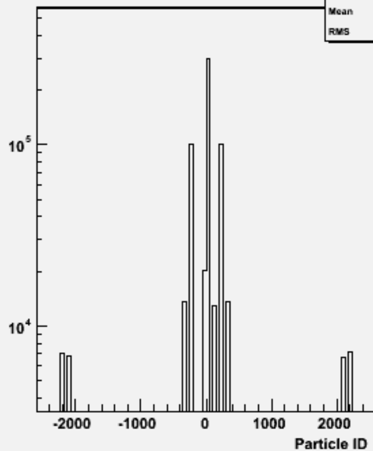
Particle ID : w104626 e2e2h_o
