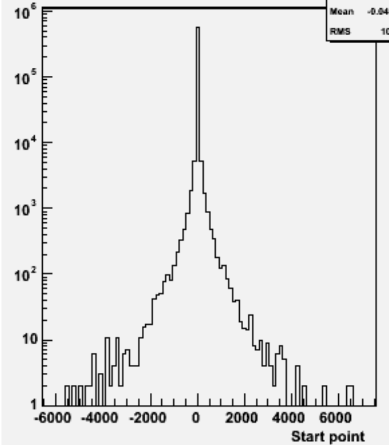
Start point Z : w104626 e2e2h_o
