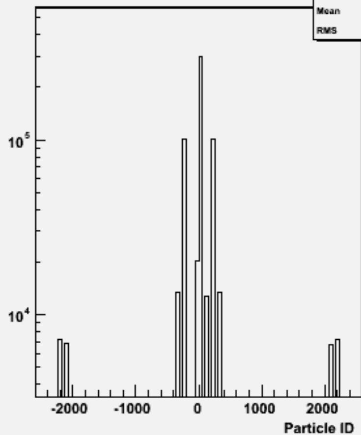
Particle ID : w104625 e2e2h_o
