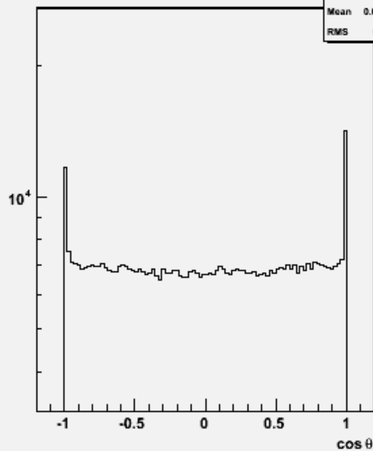
Particle cos \theta : w104625 e2e2h_o
