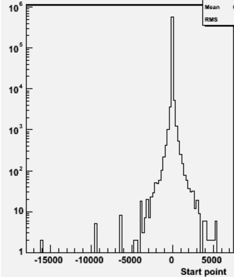
Start point Z : w104625 e2e2h_o
