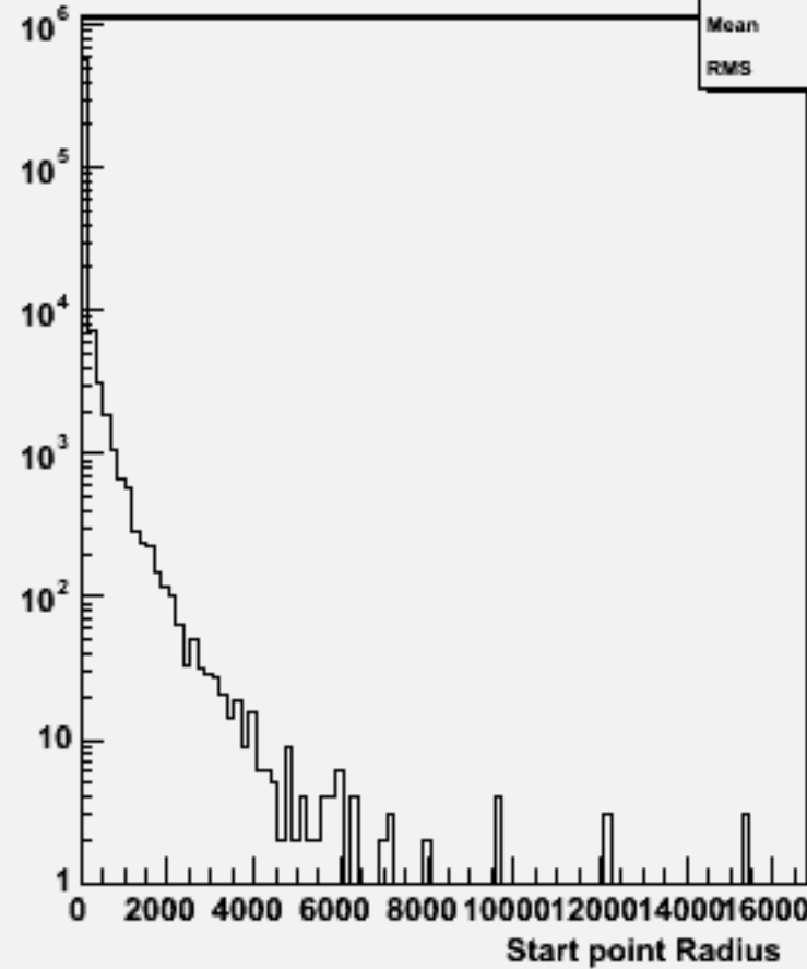
Start point R : w104625 e2e2h_o
