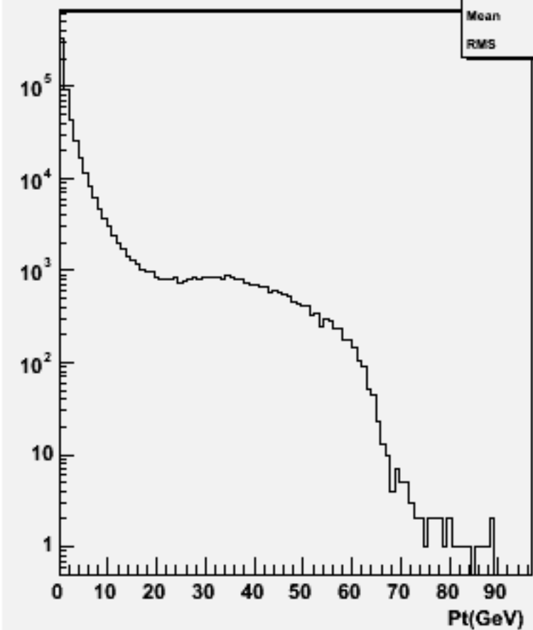
Particle Pt : w104625 e2e2h_o
