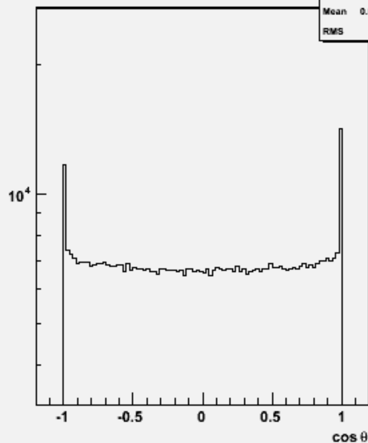
Particle cosθ : w104623 e1e1h_o
