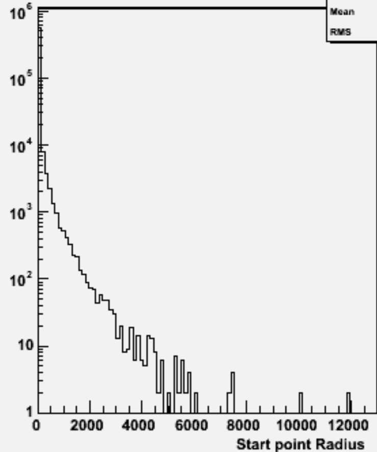
Start point R : w104623 e1e1h_o
