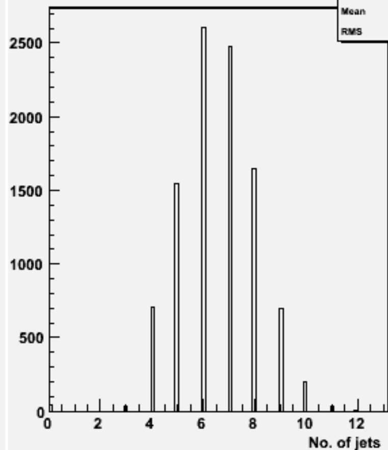
No. jets (ycut=0.001) : w104623 e1e1h_o
