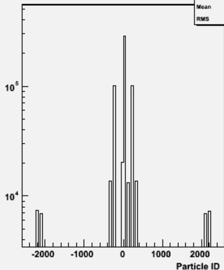
Particle ID : w104623 e1e1h_o
