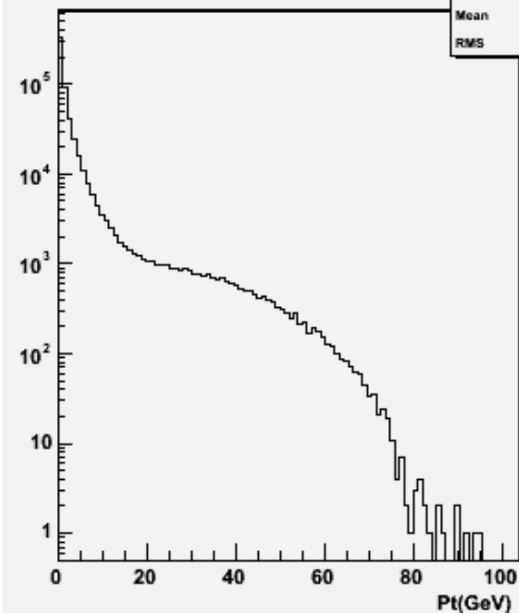
Particle Pt : w104623 e1e1h_o
