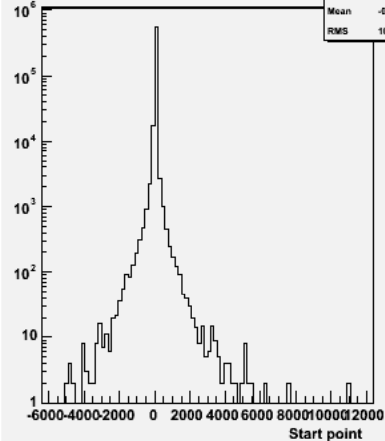
Start point Z : w104623 e1e1h_o
