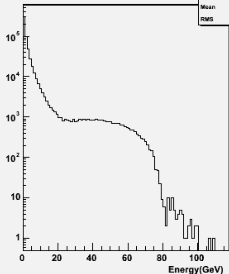
Particle Energy : w104623 e1e1h_o
