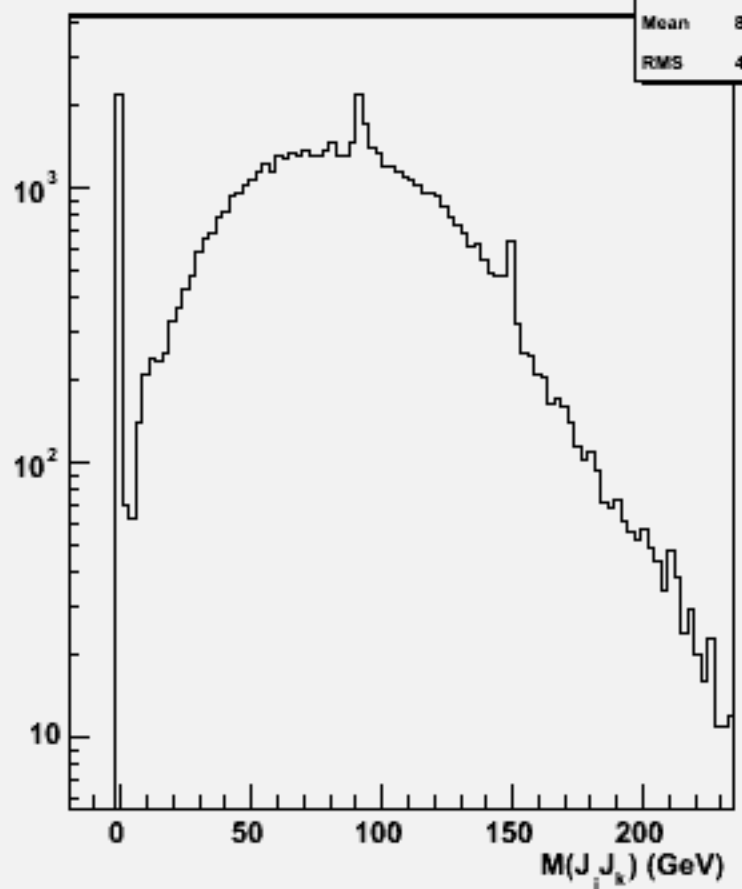
2jets mass(All comb)w104621 e1e1h_o
