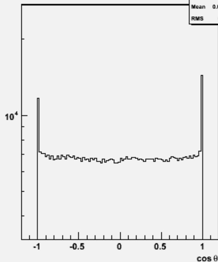
Particle cos \theta : w104621 e1e1h_o
