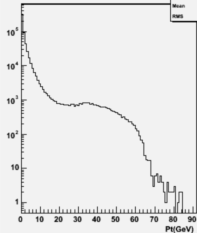
Particle Pt : w104621 e1e1h_o
