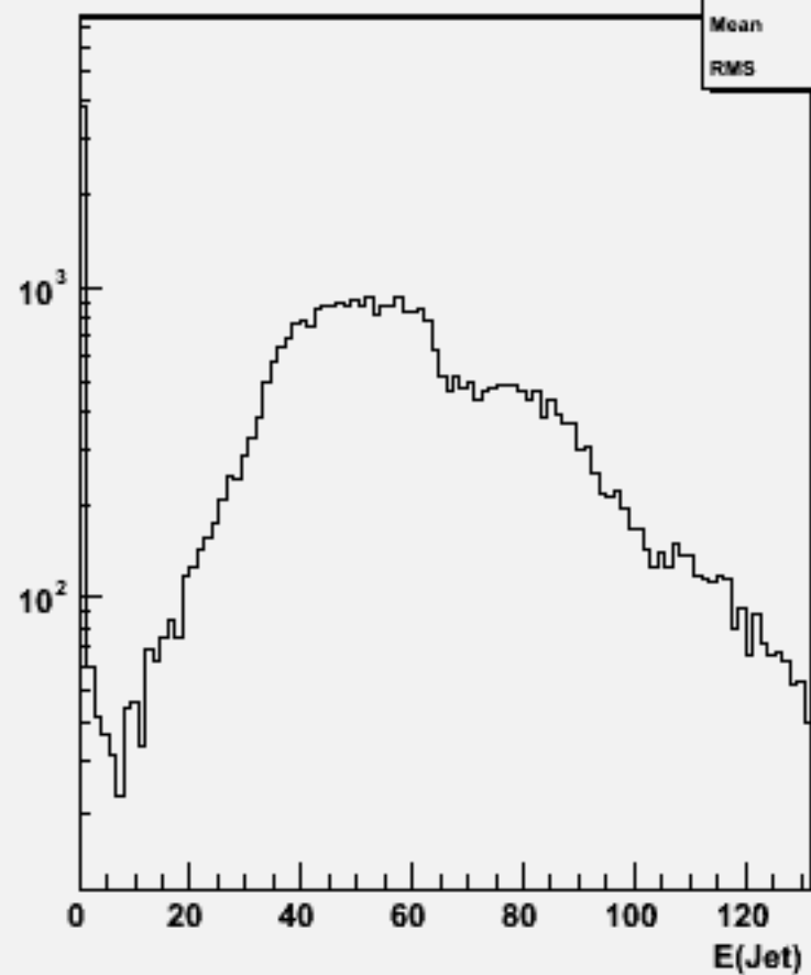
Jet energies(All jets)w104621 e1e1h_o
