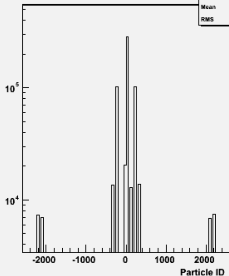
Particle ID : w104621 e1e1h_o
