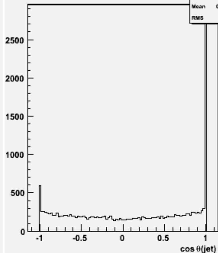
cos \theta for 2-jets :w104621 e1e1h_o
