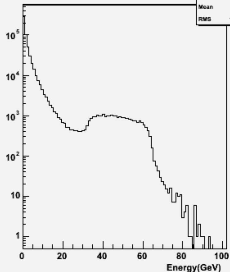
Particle Energy : w104621 e1e1h_o
