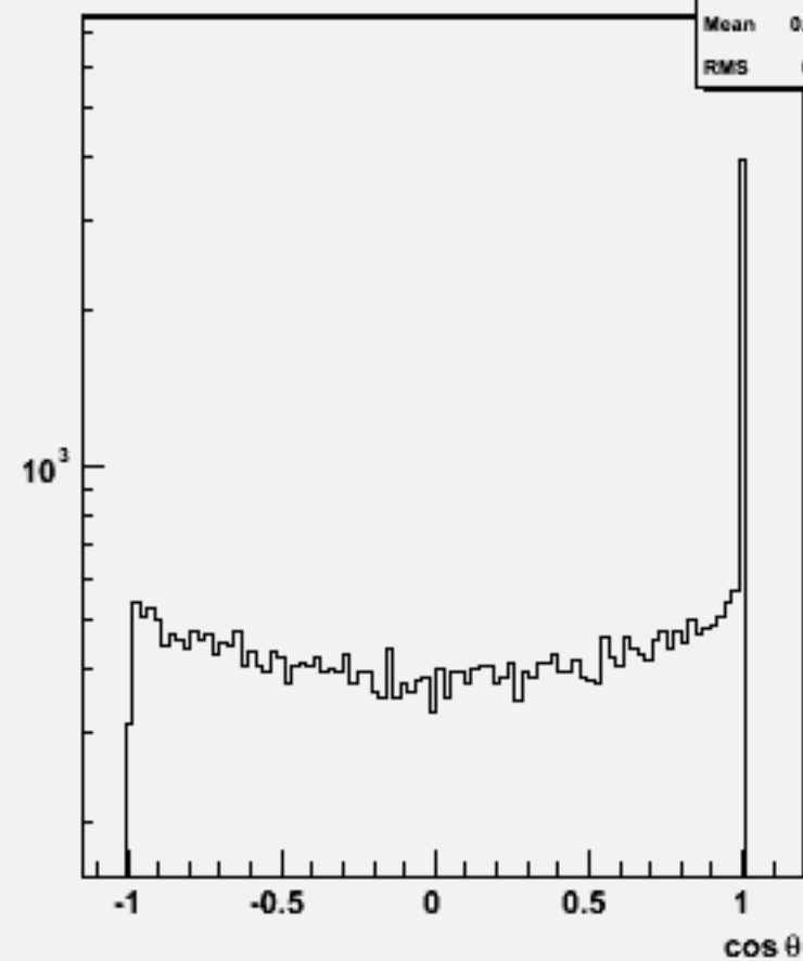
Jet cos \theta (All jets)w104621 e1e1h_o
