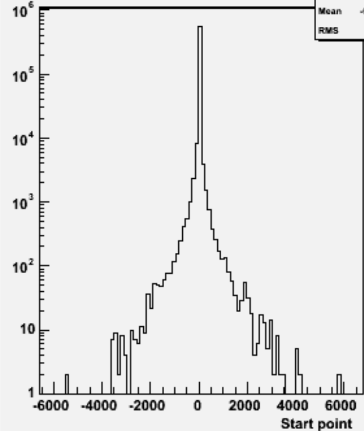
Start point Z : w104621 e1e1h_o
