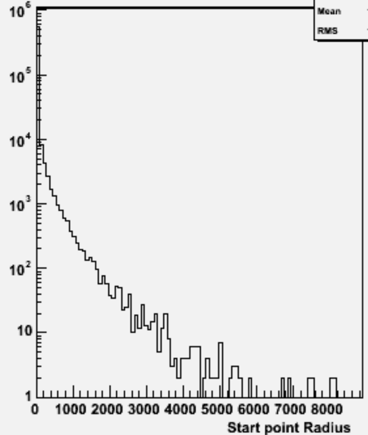
Start point R : w104621 e1e1h_o
