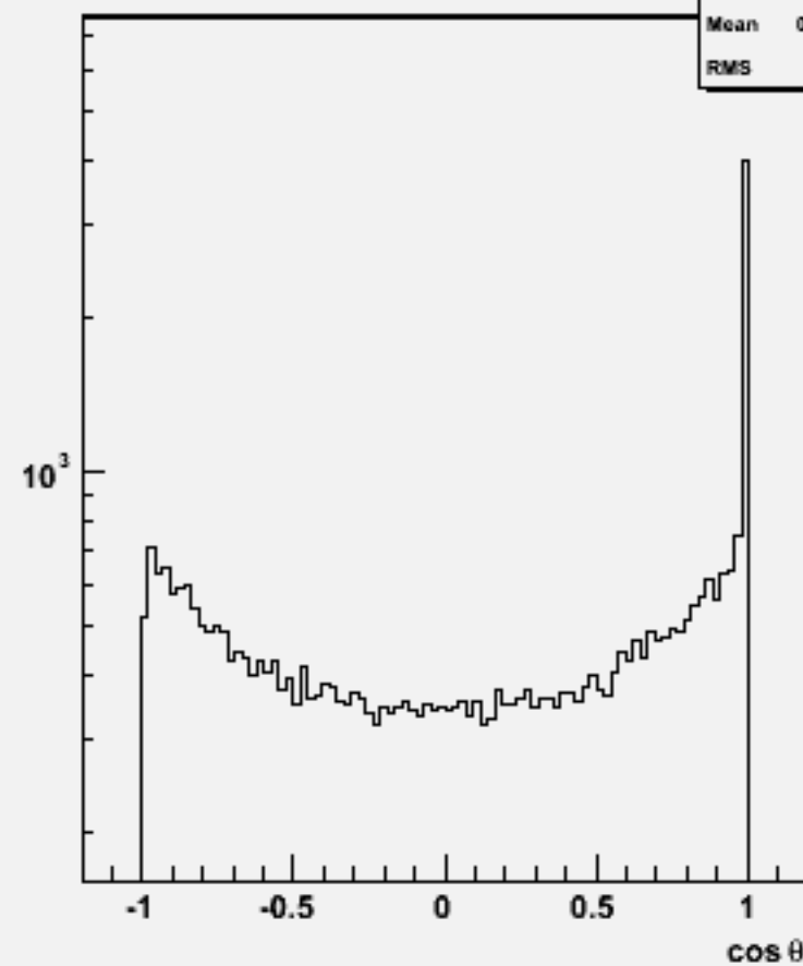
Jet cos \theta (All jets)w104620 e1e1h_o
