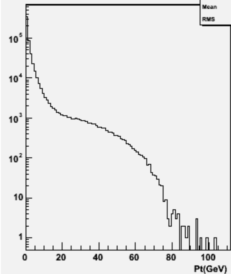
Particle Pt : w104620 e1e1h_o
