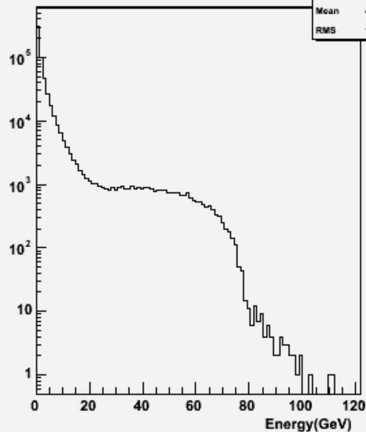
Particle Energy : w104620 e1e1h_o
