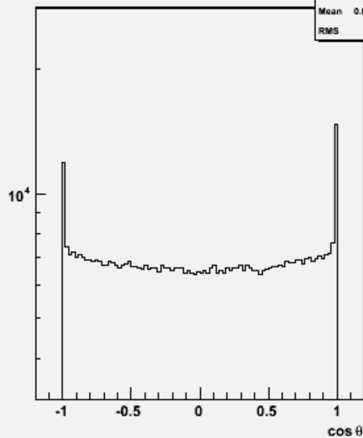
Particle cosθ : w104620 e1e1h_o
