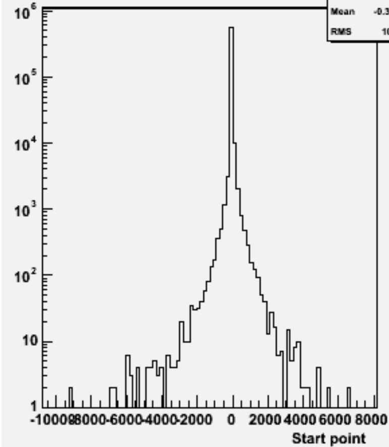
Start point Z : w104620 e1e1h_o
