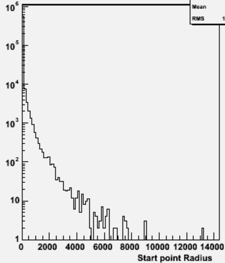
Start point R : w104620 e1e1h_o
