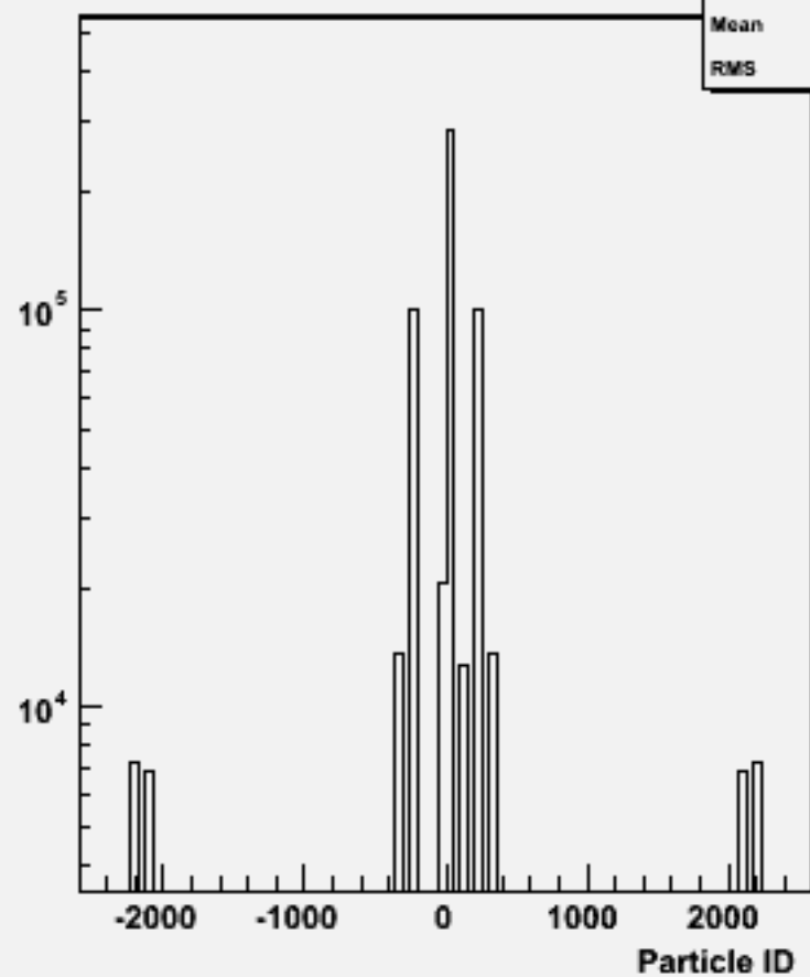
Particle ID : w104620 e1e1h_o
