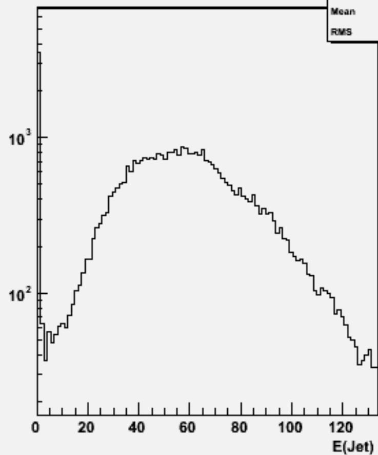
Jet energies(All jets)w104620 e1e1h_o
