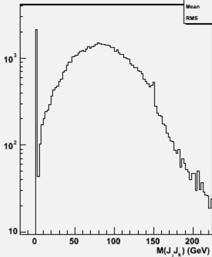
2jets mass(All comb)w104620 e1e1h_o
