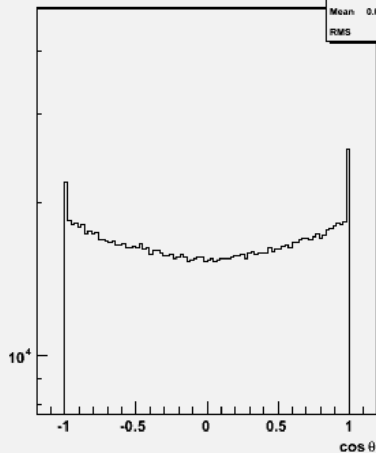
Particle \cos\theta : w104618 cch_o
