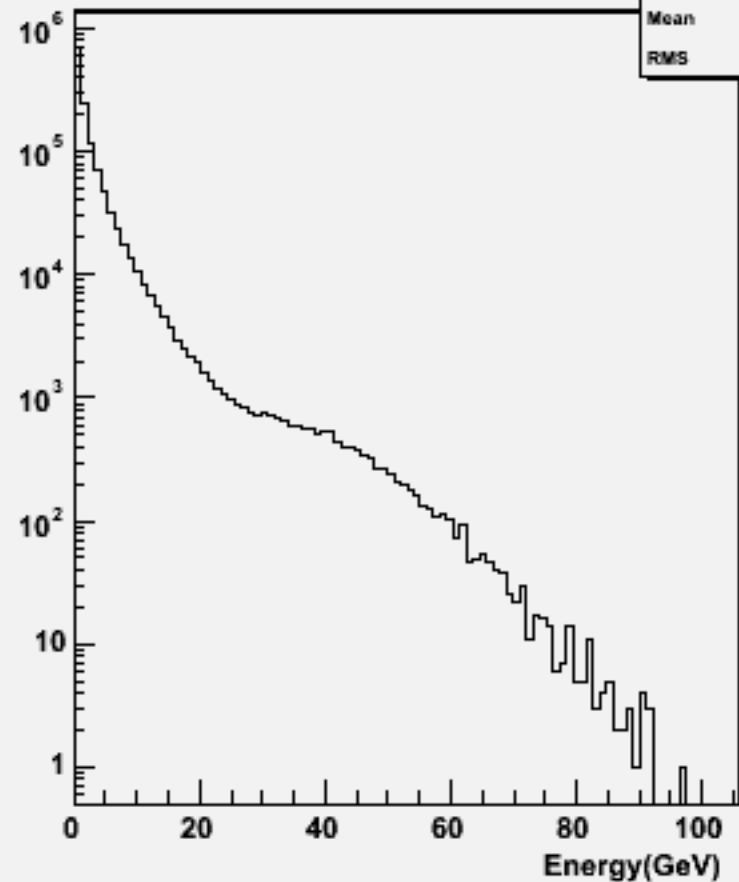
Start point R : w104614 uuh_o
