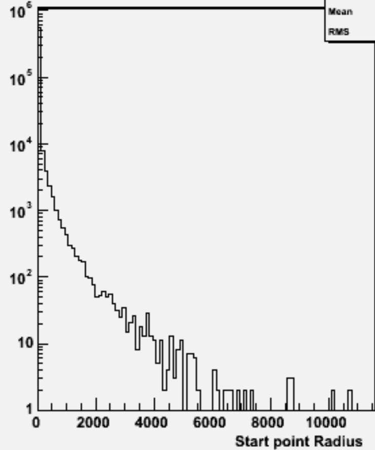
Start point R : w104610 n3n3h_o
