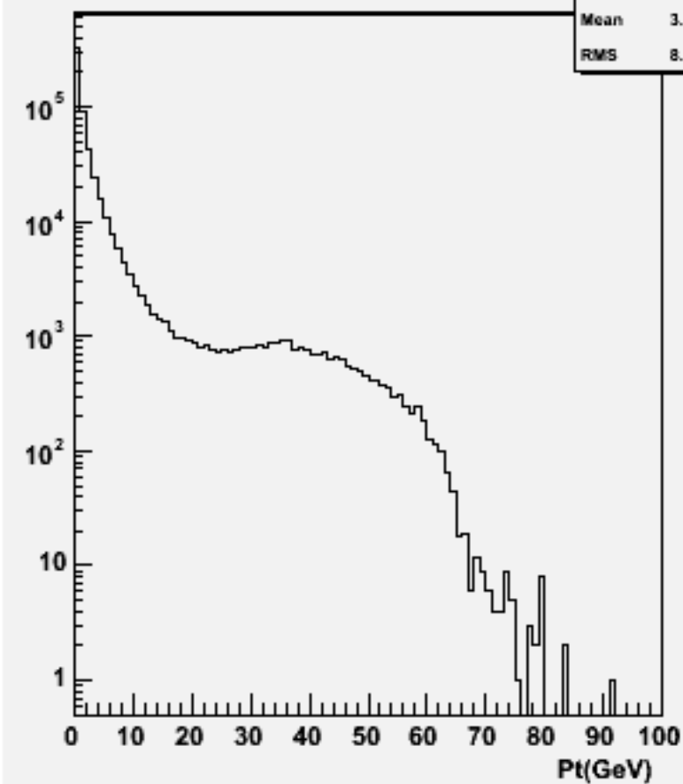
Particle Pt : w104610 n3n3h_o
