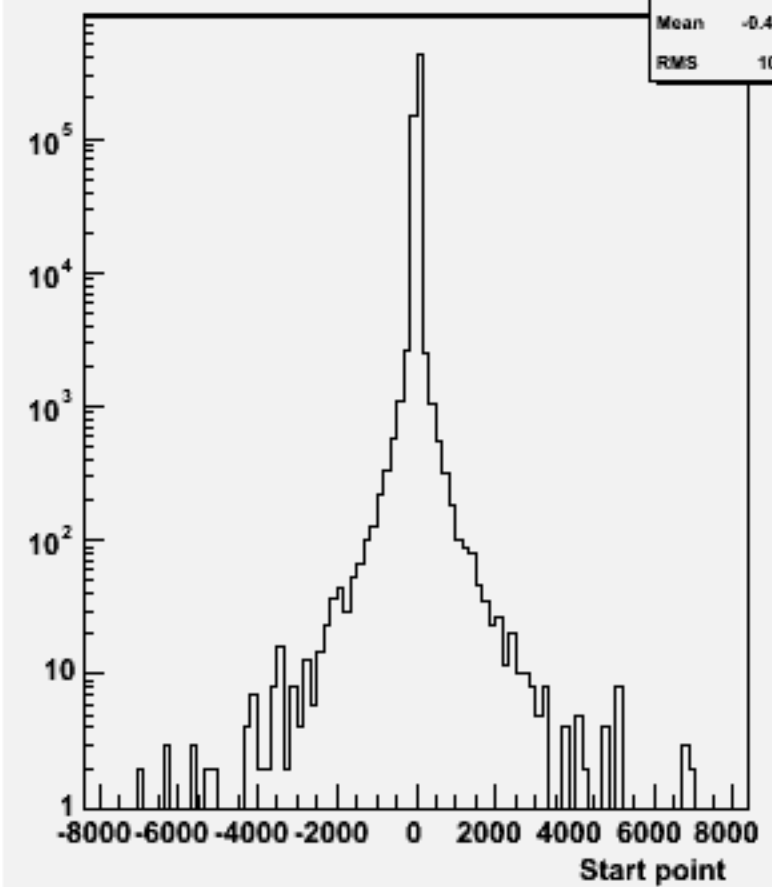
Start point Z : w104610 n3n3h_o
