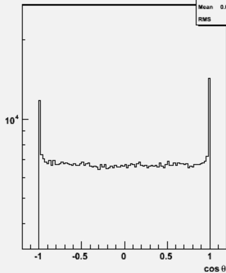
Particle cosθ : w104610 n3n3h_o
