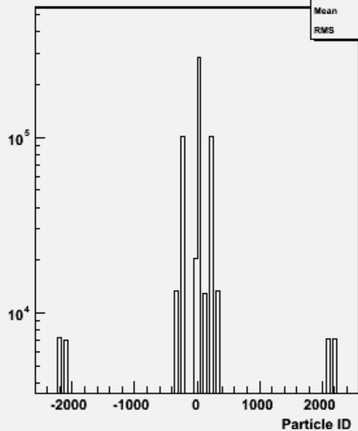
Particle ID : w104610 n3n3h_o
