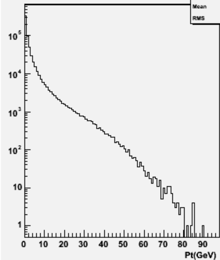
Particle Pt : w104579 e3e3h_o
