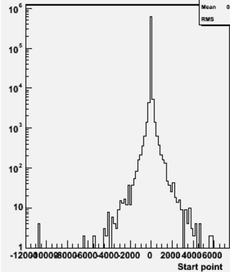
Start point Z : w104579 e3e3h_o
