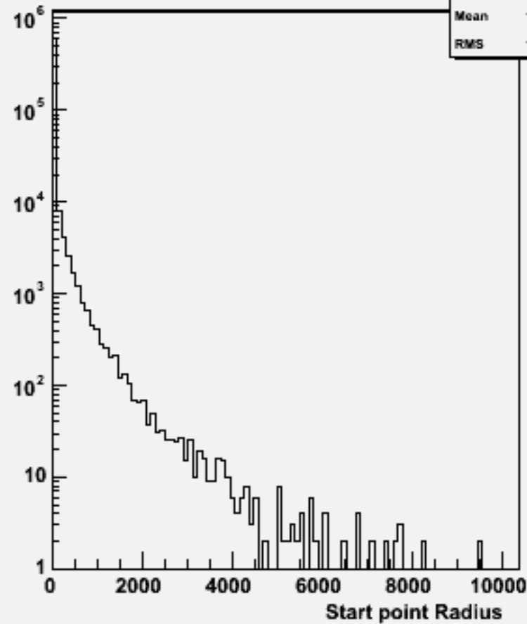
Start point R : w104579 e3e3h_o
