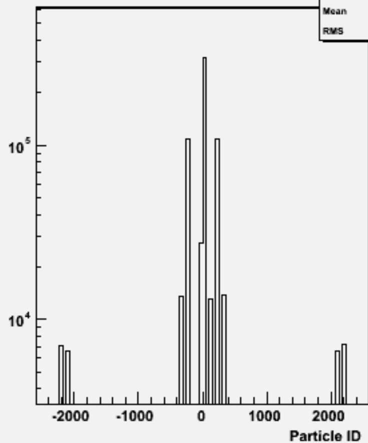
Particle ID : w104579 e3e3h_o
