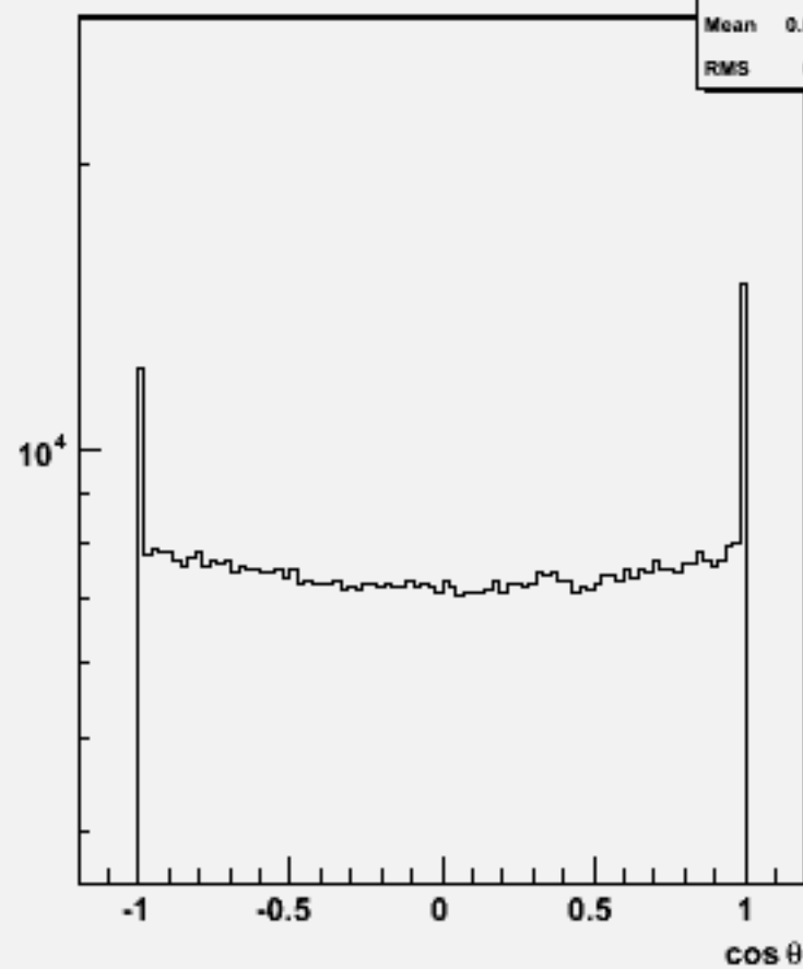
Particle \cos\theta : w104579 e3e3h_o
