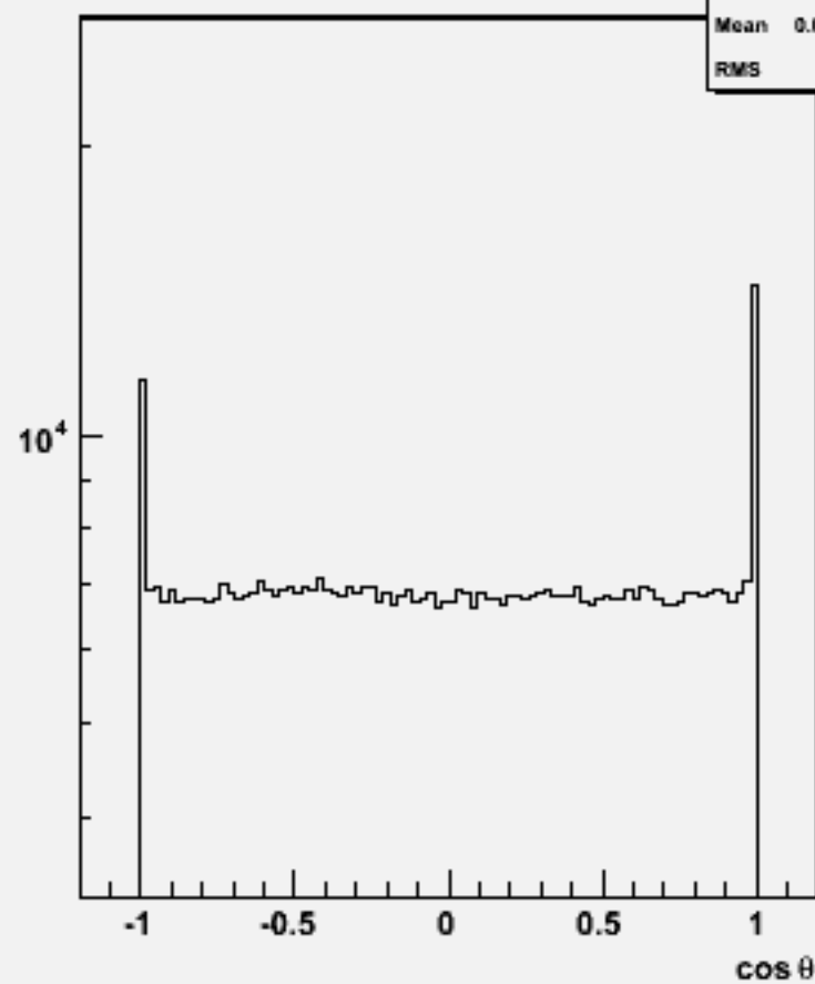
Particle cosθ : w104576 e2e2h_o
