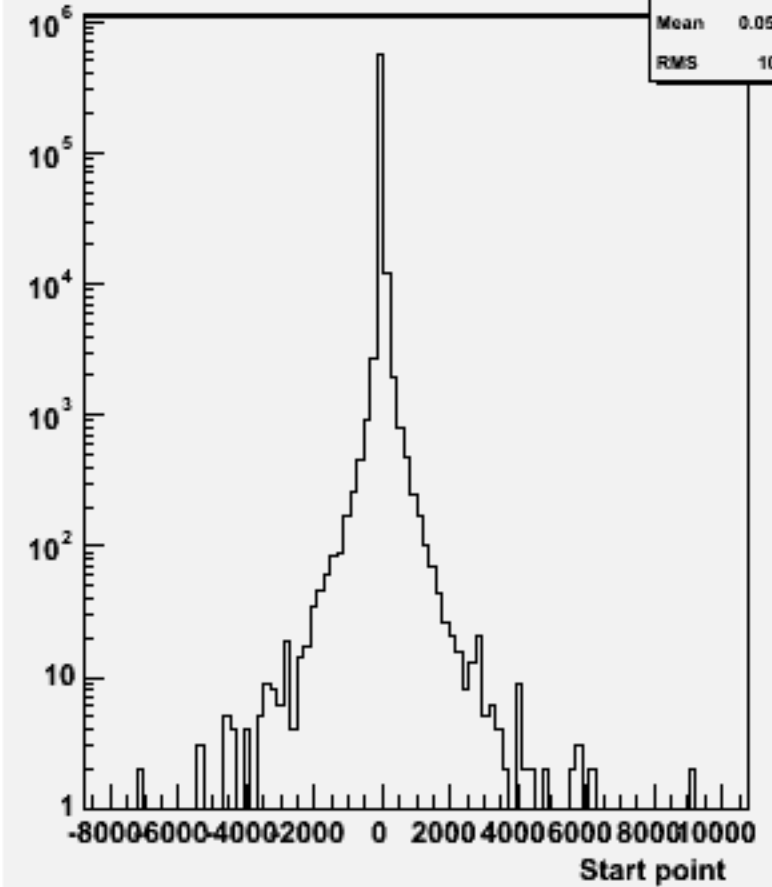
Start point Z : w104576 e2e2h_o
