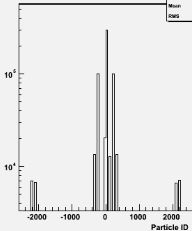
Particle ID : w104576 e2e2h_o
