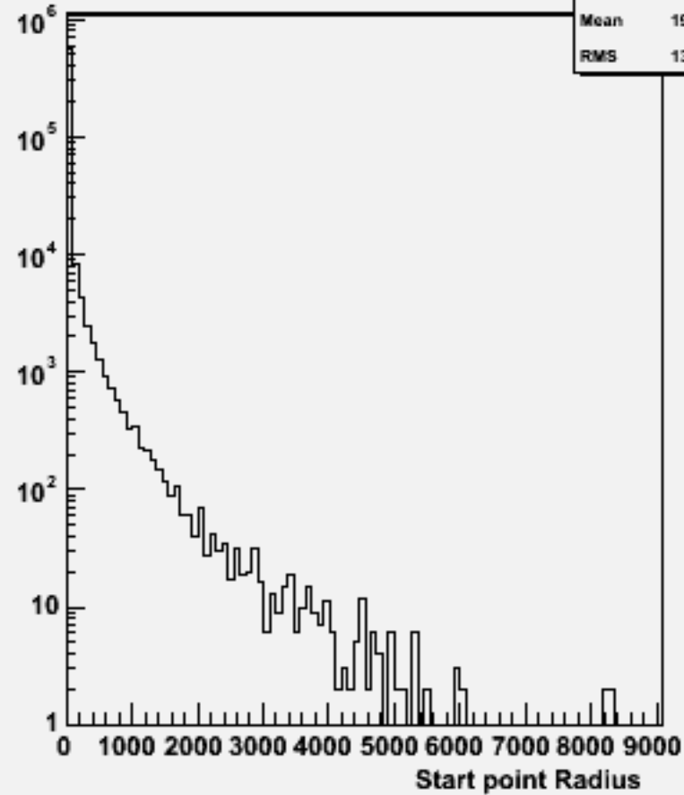
Start point R : w104576 e2e2h_o
