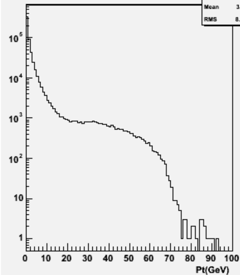
Particle Pt : w104576 e2e2h_o
