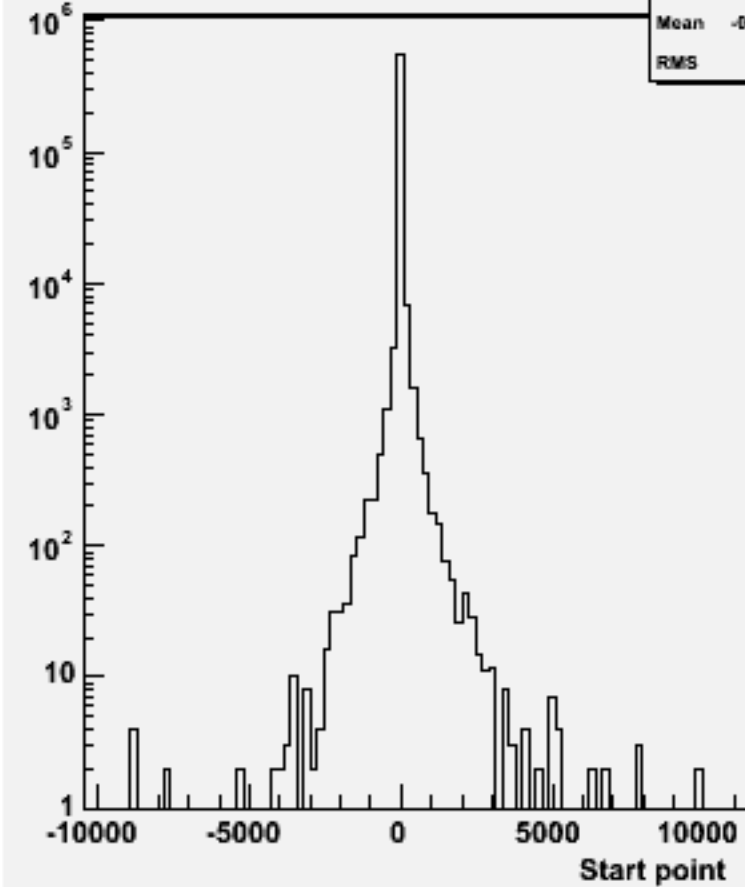
Start point Z : w104573 e1e1h_o
