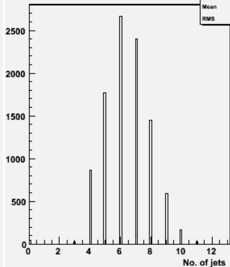
No. jets (ycut=0.001) : w104573 e1e1h_o
