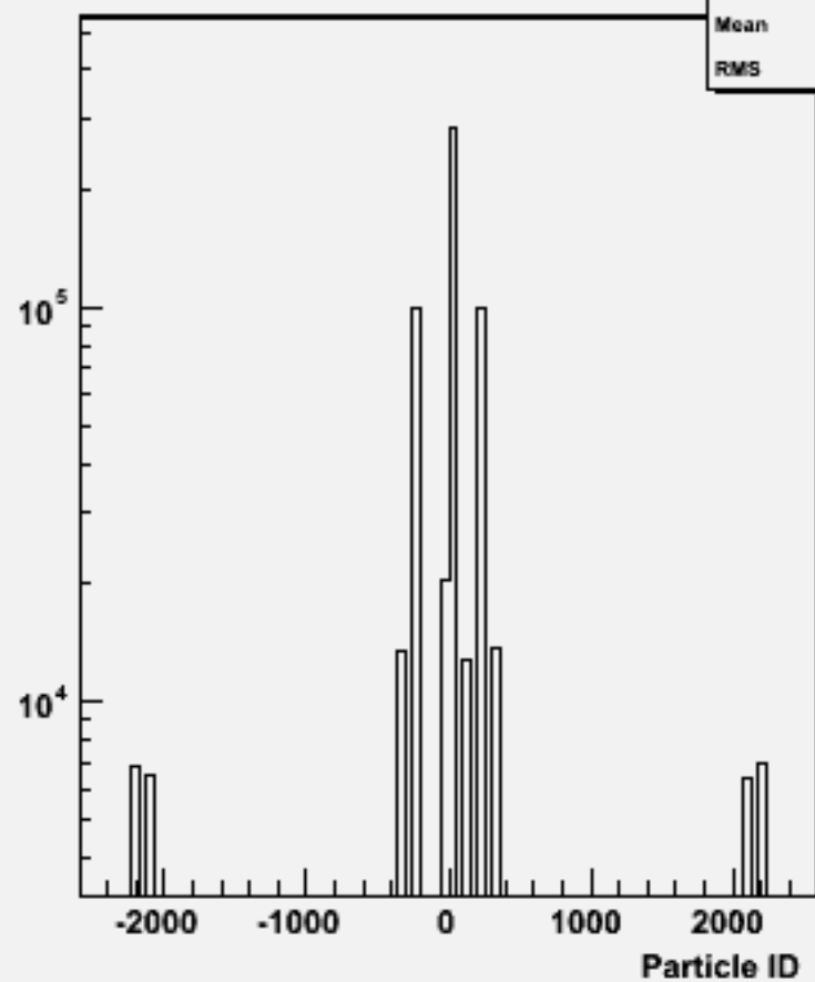
Particle ID : w104573 e1e1h_o
