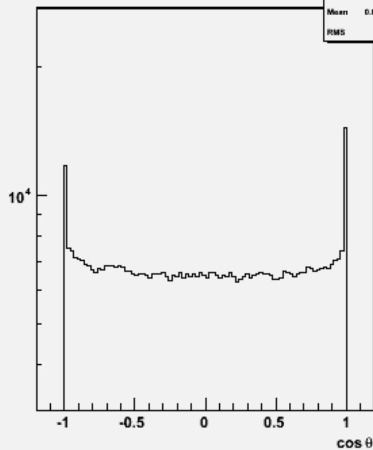
Particle cosθ : w104573 e1e1h_o
