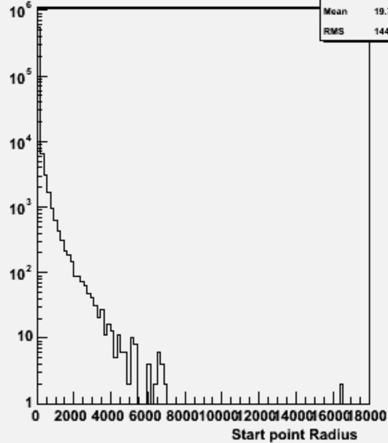
Start point R : w104573 e1e1h_o
