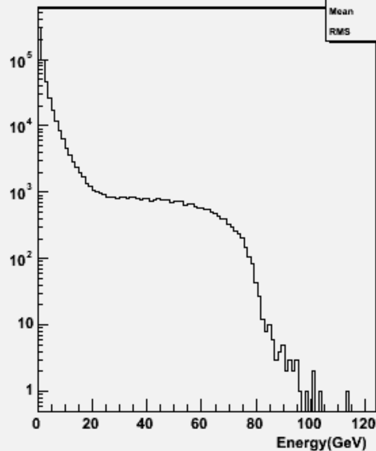
Particle Energy : w104573 e1e1h_o
