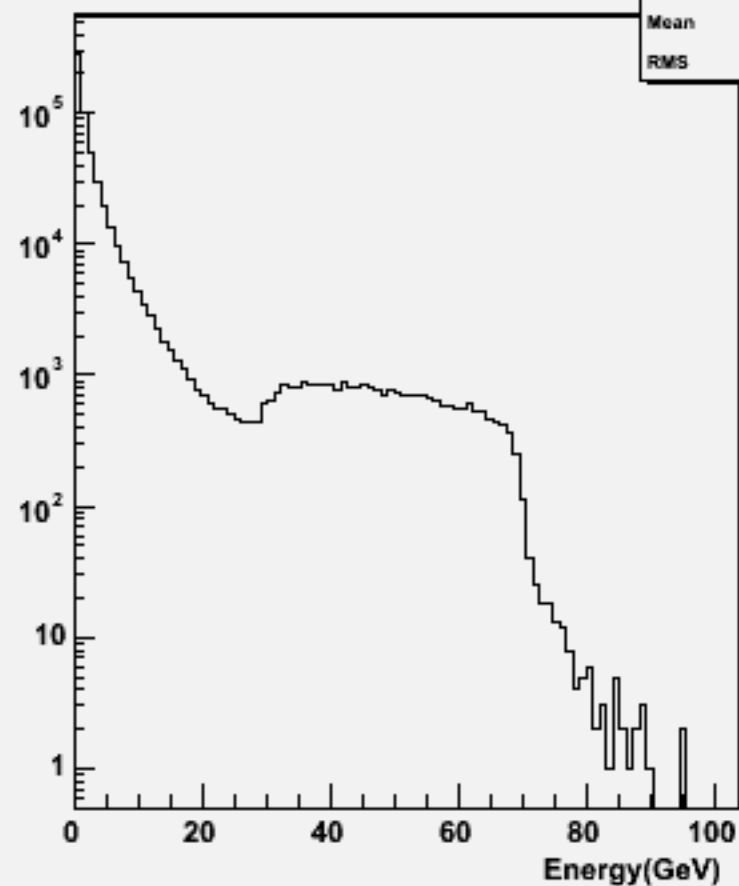
Particle Energy : w104572 e1e1h_o
