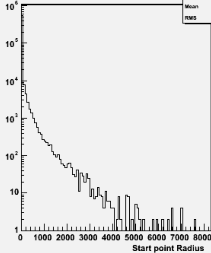
Start point R : w104572 e1e1h_o
