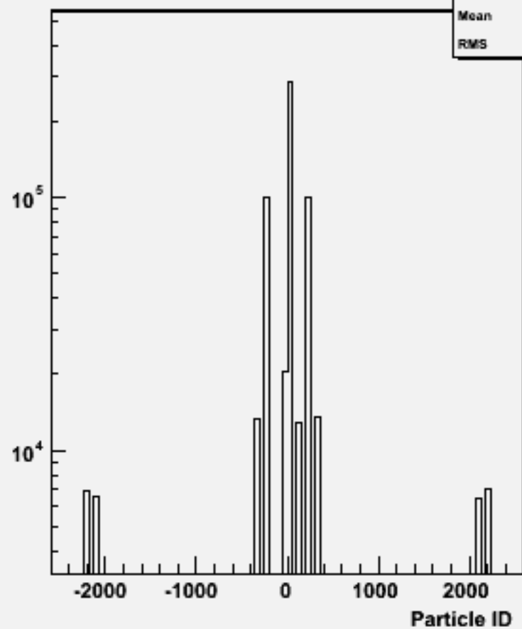
Particle ID : w104572 e1e1h_o
