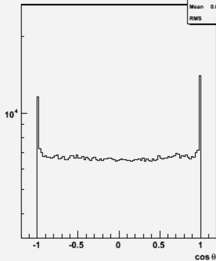
Particle cosθ : w104572 e1e1h_o
