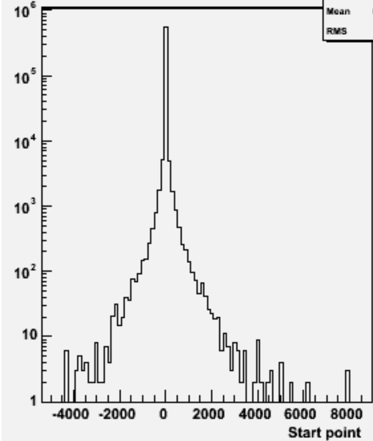
Start point Z : w104572 e1e1h_o
