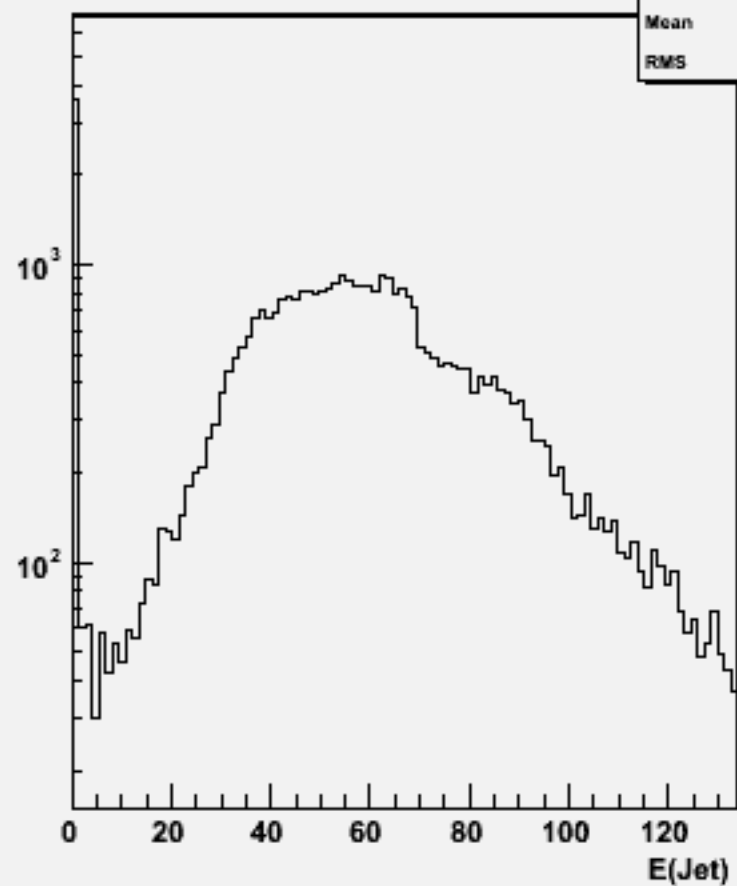
Jet energies(All jets)w104572 e1e1h_o
