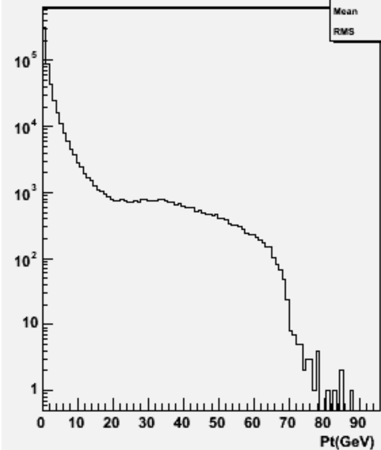
Particle Pt : w104572 e1e1h_o
