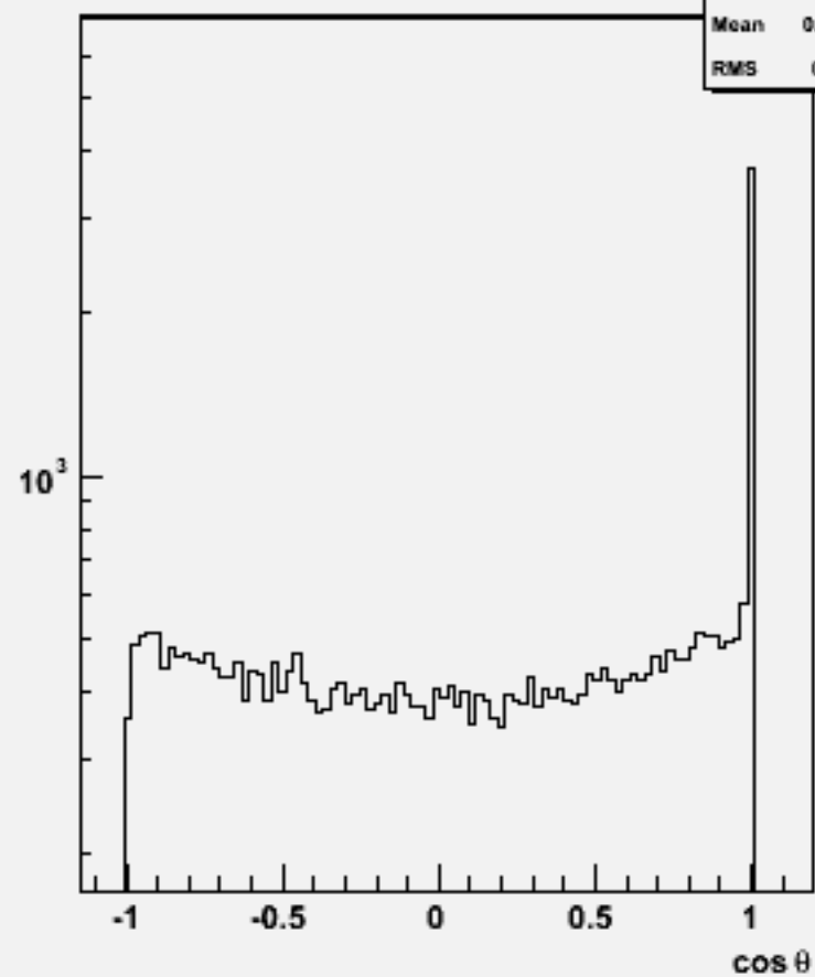
Jet cos \theta (All jets)w104572 e1e1h_o
