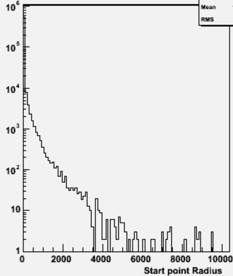
Start point R : w104571 e1e1h_o
