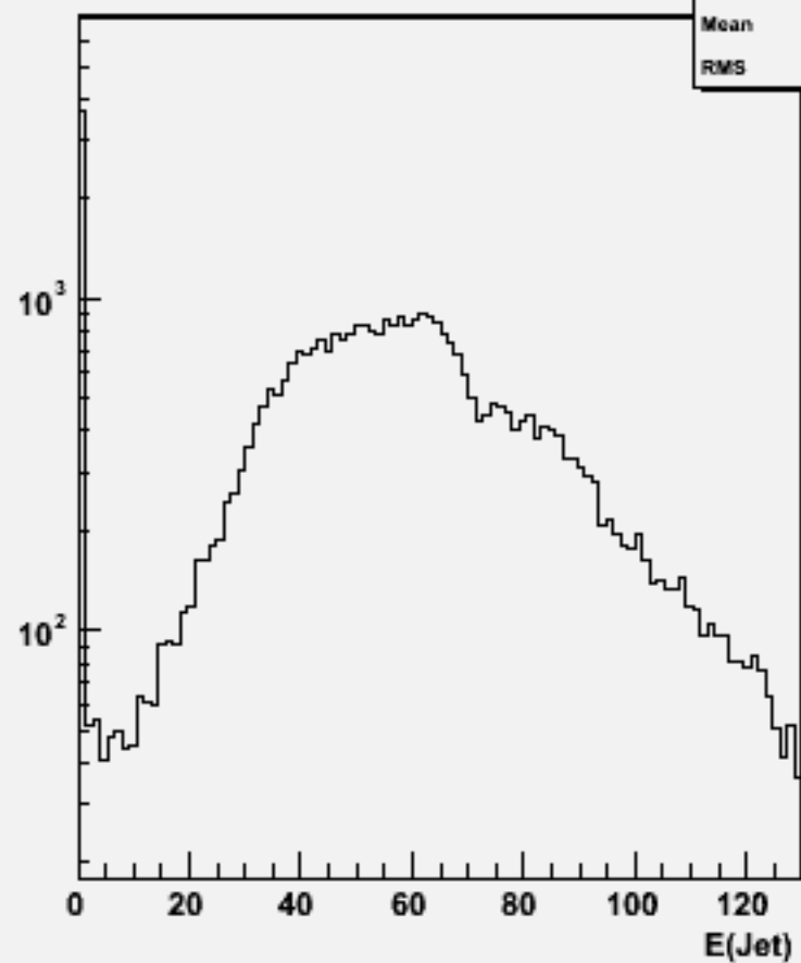
Jet energies(All jets)w104571 e1e1h_o
