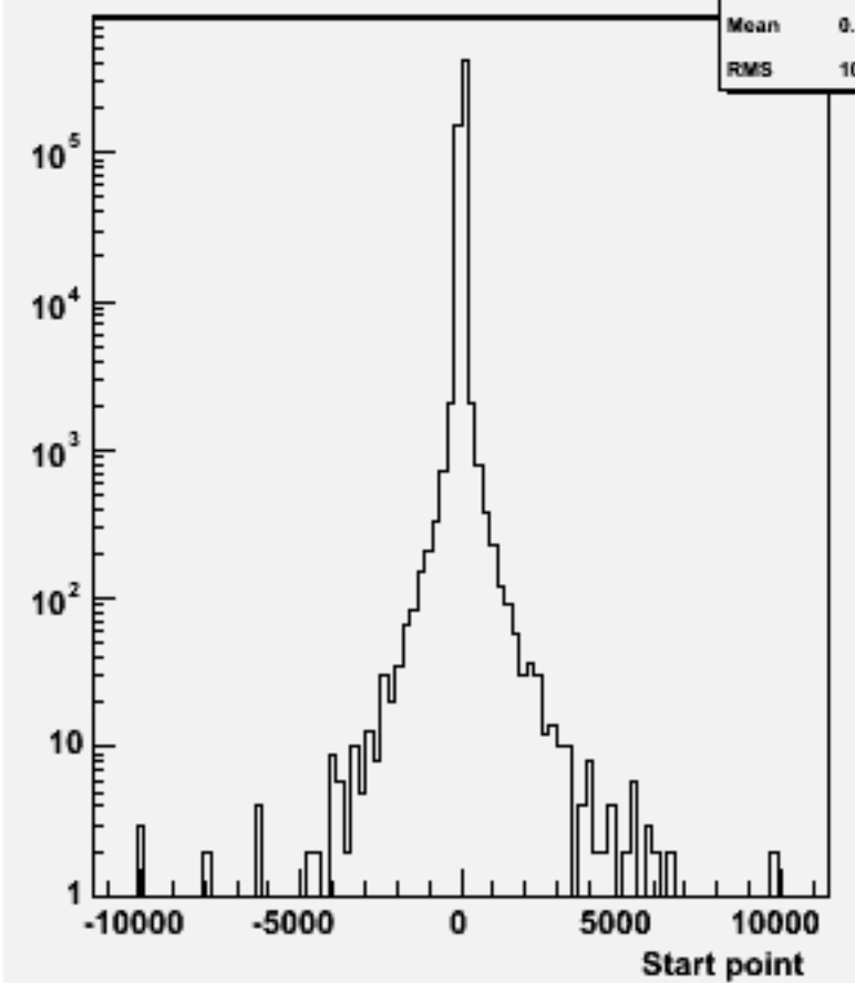
Start point Z : w104571 e1e1h_o
