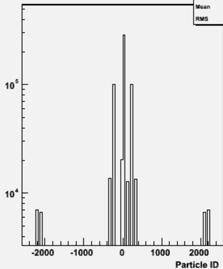
Particle ID : w104571 e1e1h_o
