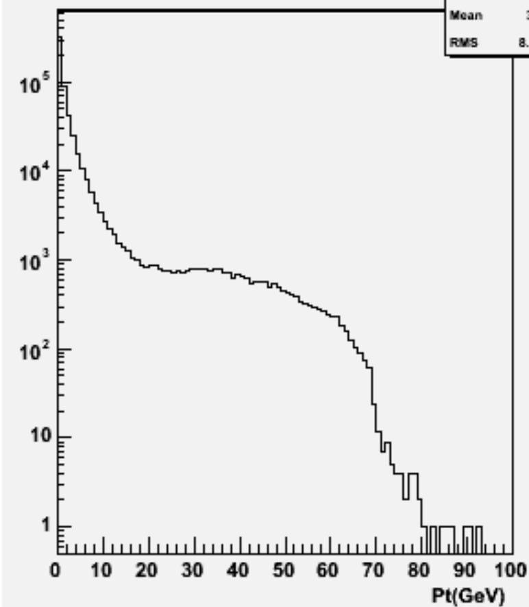
Particle Pt : w104571 e1e1h_o
