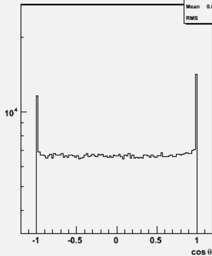
Particle cos \theta : w104571 e1e1h_o
