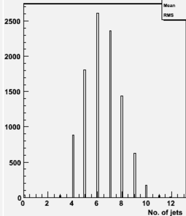
No. jets (ycut=0.001) : w104571 e1e1h_o
