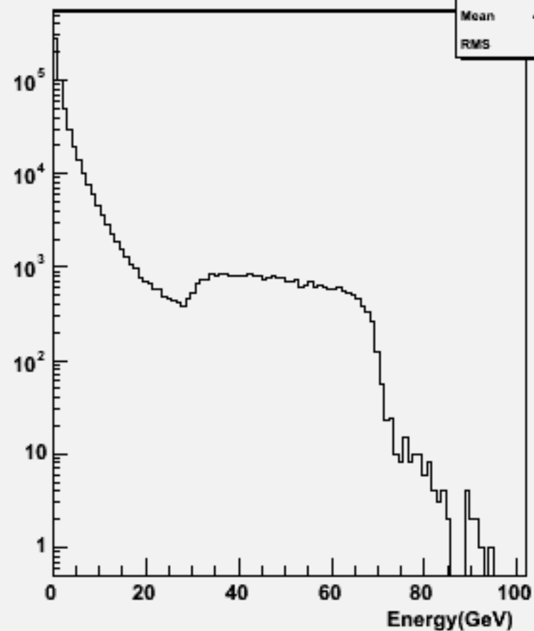
Particle Energy : w104571 e1e1h_o
