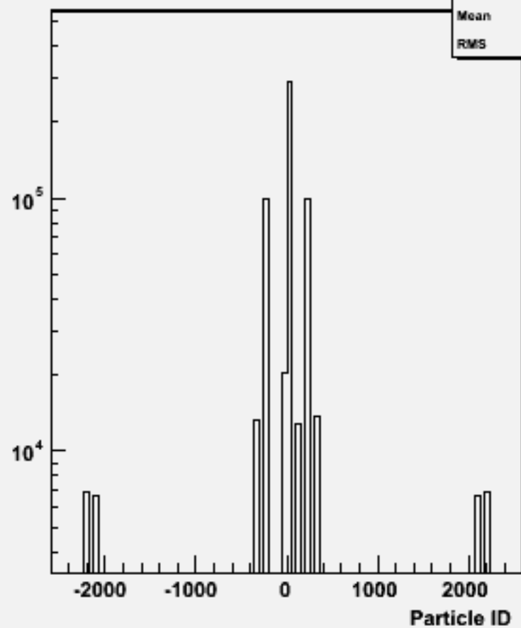
Particle ID : w104570 e1e1h_o
