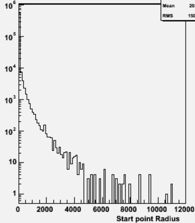
Start point R : w104570 e1e1h_o
