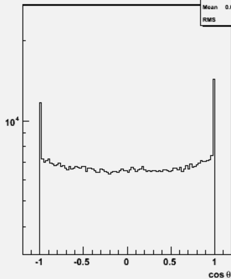
Particle cosθ : w104570 e1e1h_o
