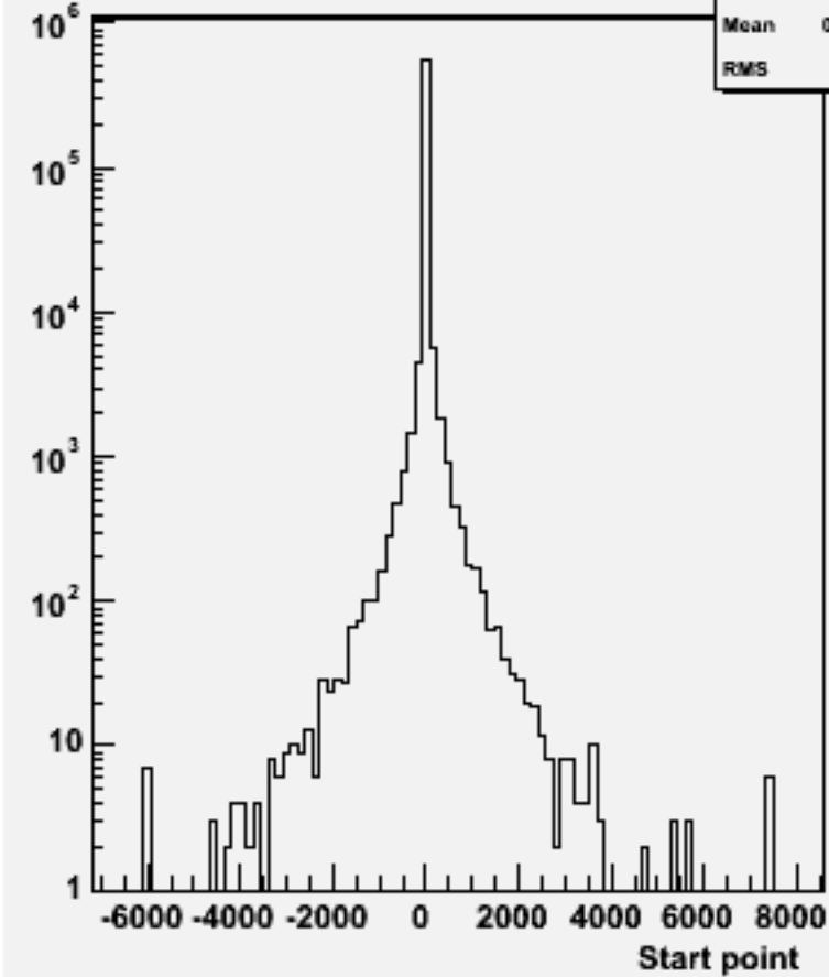
Start point Z : w104570 e1e1h_o
