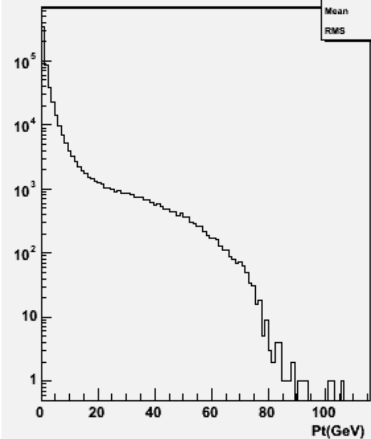
Particle Pt : w104570 e1e1h_o
