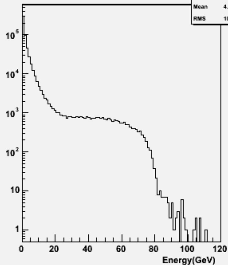
Particle Energy : w104570 e1e1h_o
