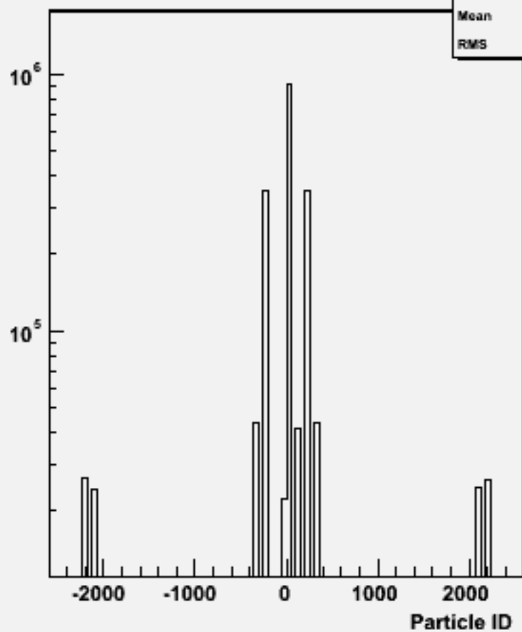
Particle ID : w104564 uuh_o
