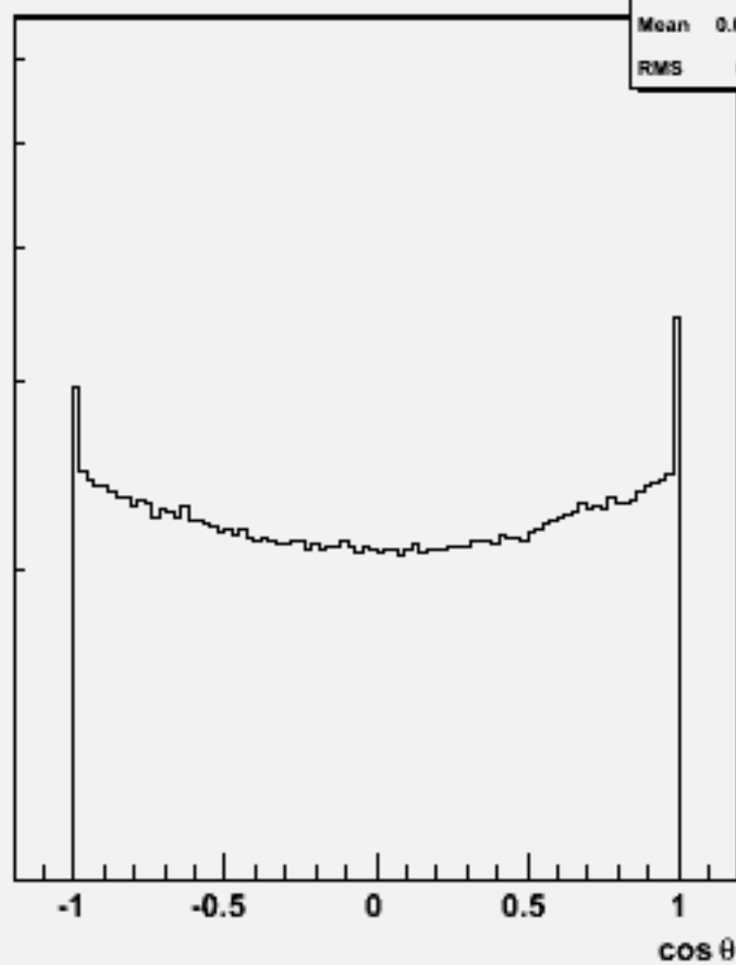
Particle \cos\theta : w104564 uuh_o
