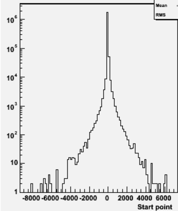
Start point Z : w104564 uuh_o
