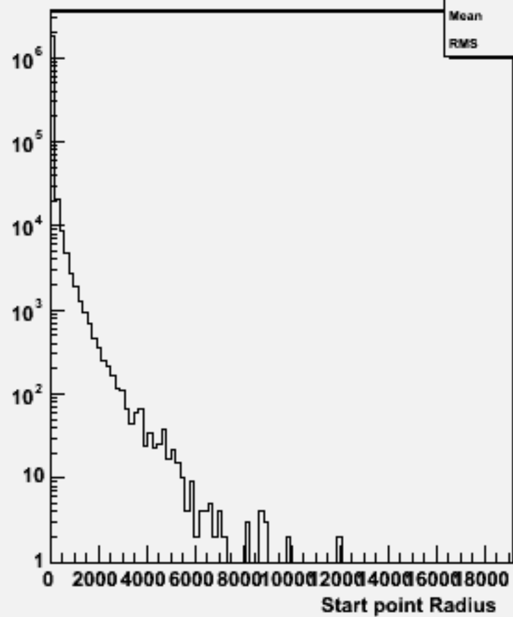
Start point R : w104564 uuh_o
