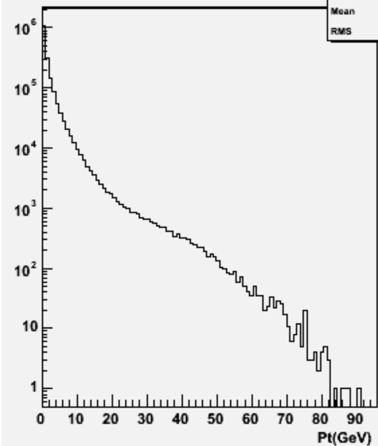
Particle Pt : w104564 uuh_o
