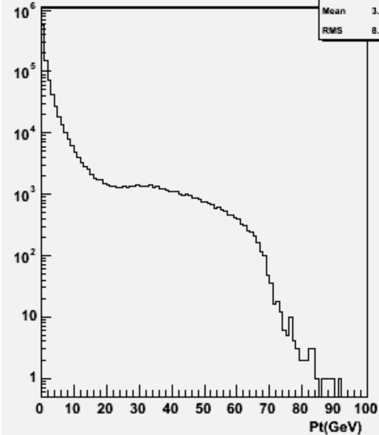
Particle Pt : w104559 n3n3h_o
