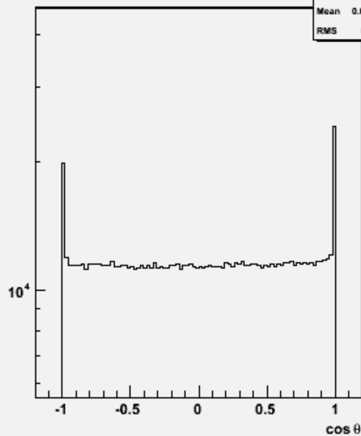
Particle cos \theta : w104559 n3n3h_o
