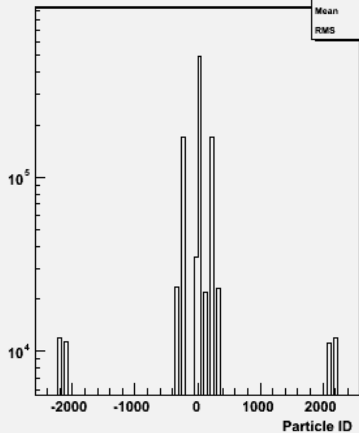
Particle ID : w104559 n3n3h_o
