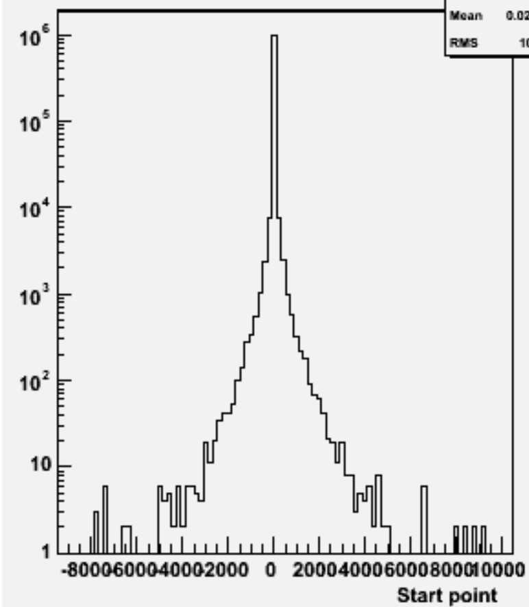
Start point Z : w104559 n3n3h_o
