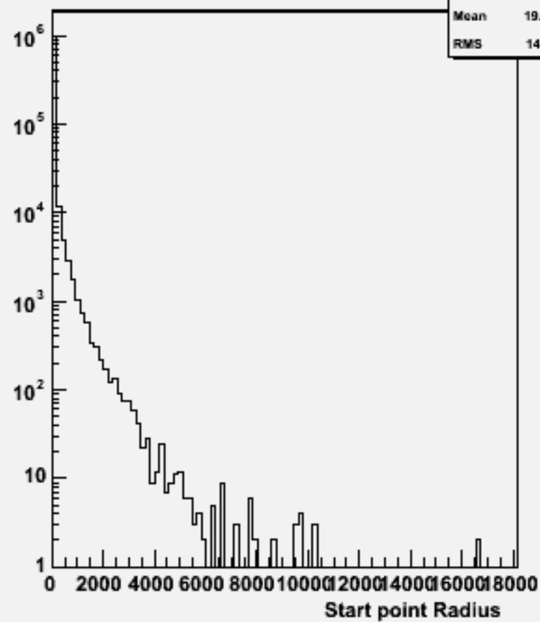
Start point R : w104559 n3n3h_o
