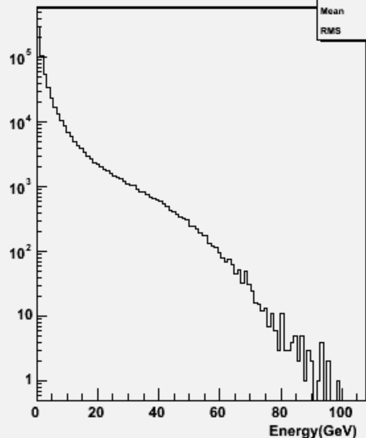
Particle Energy : w104530 e3e3h_o
