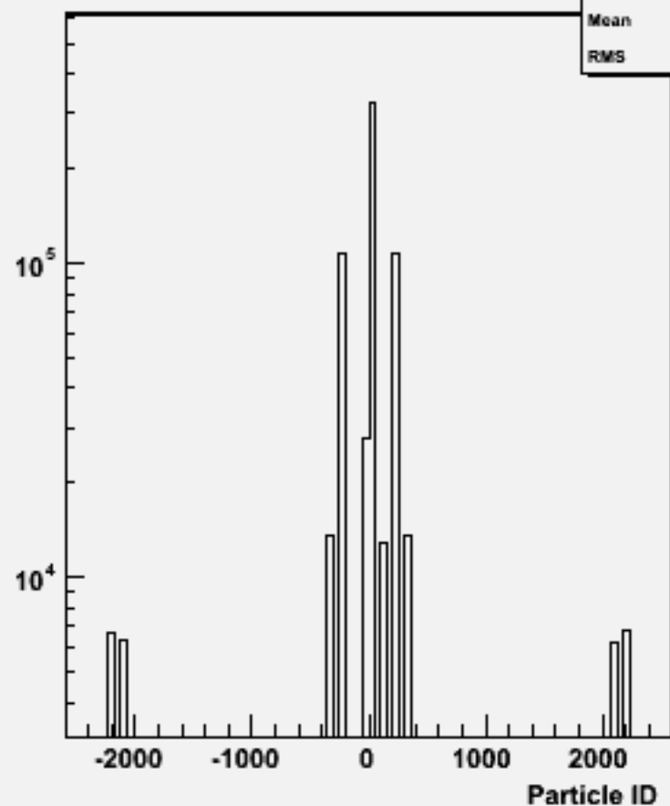
Particle ID : w104530 e3e3h_o
