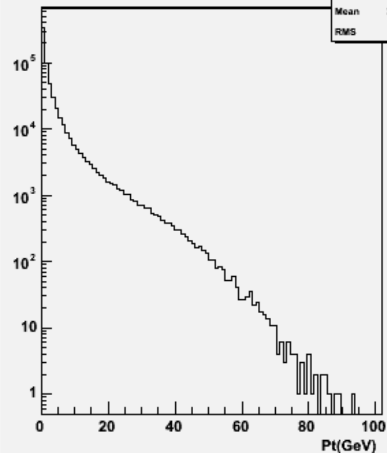
Particle Pt : w104530 e3e3h_o
