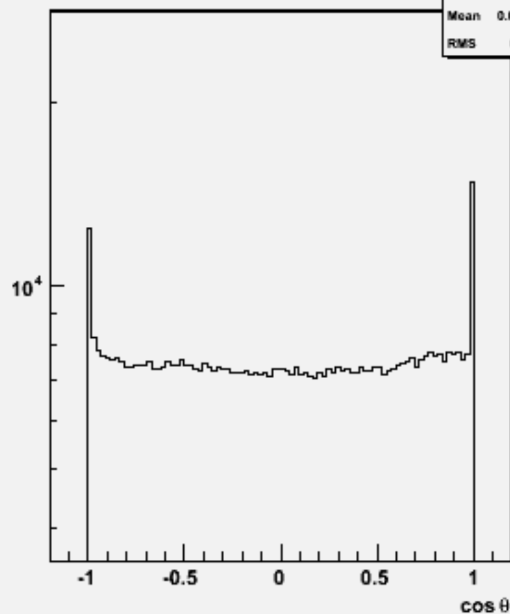
Particle cosθ : w104530 e3e3h_o
