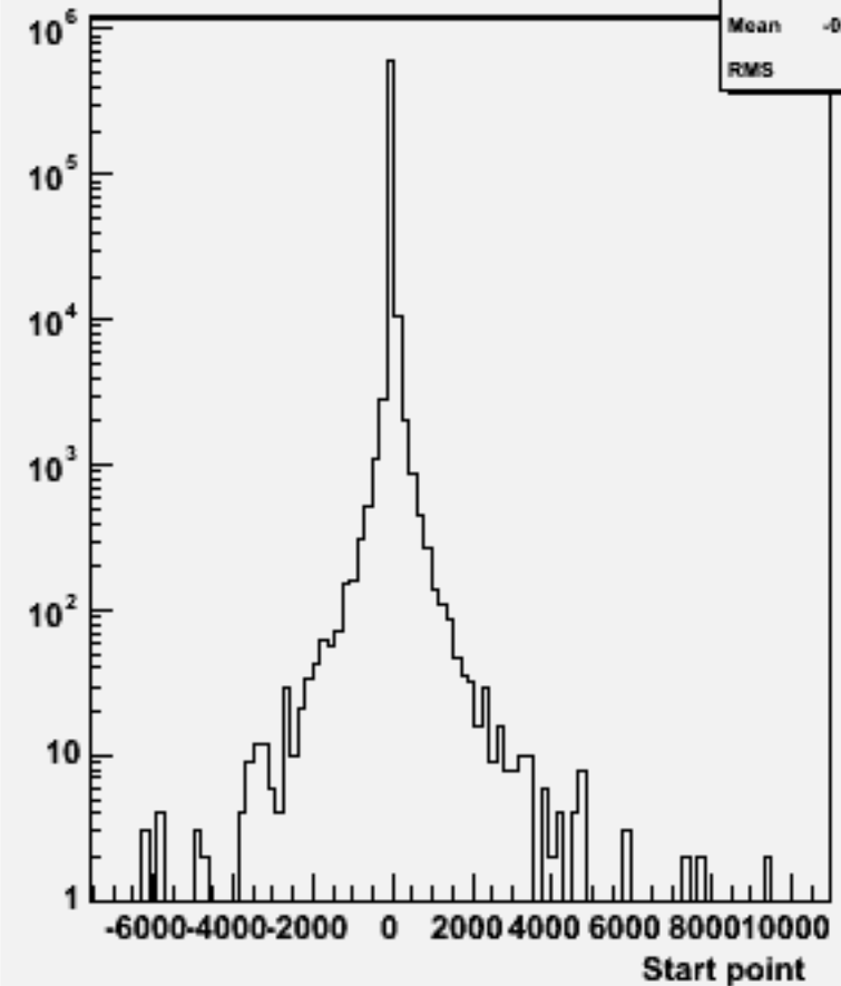
Start point Z : w104530 e3e3h_o
