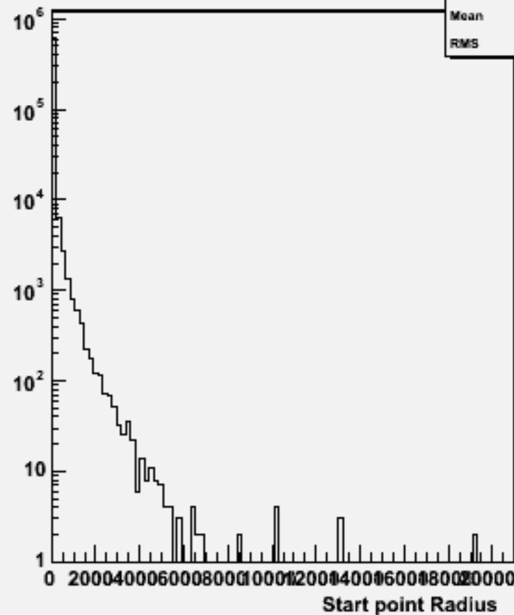
Start point R : w104530 e3e3h_o
