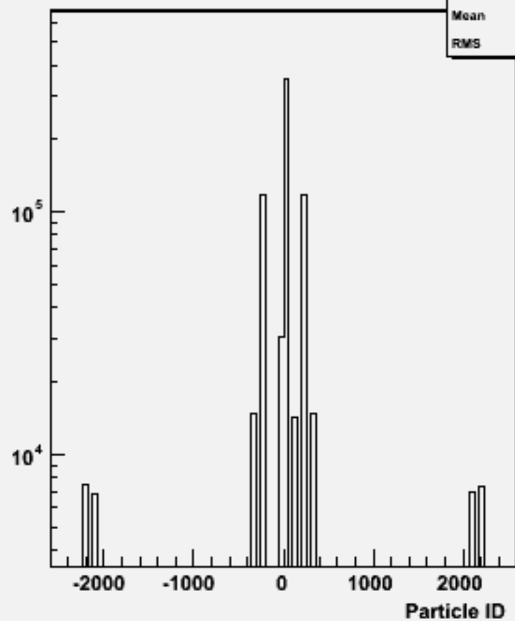
Particle ID : w104529 e3e3h_o
