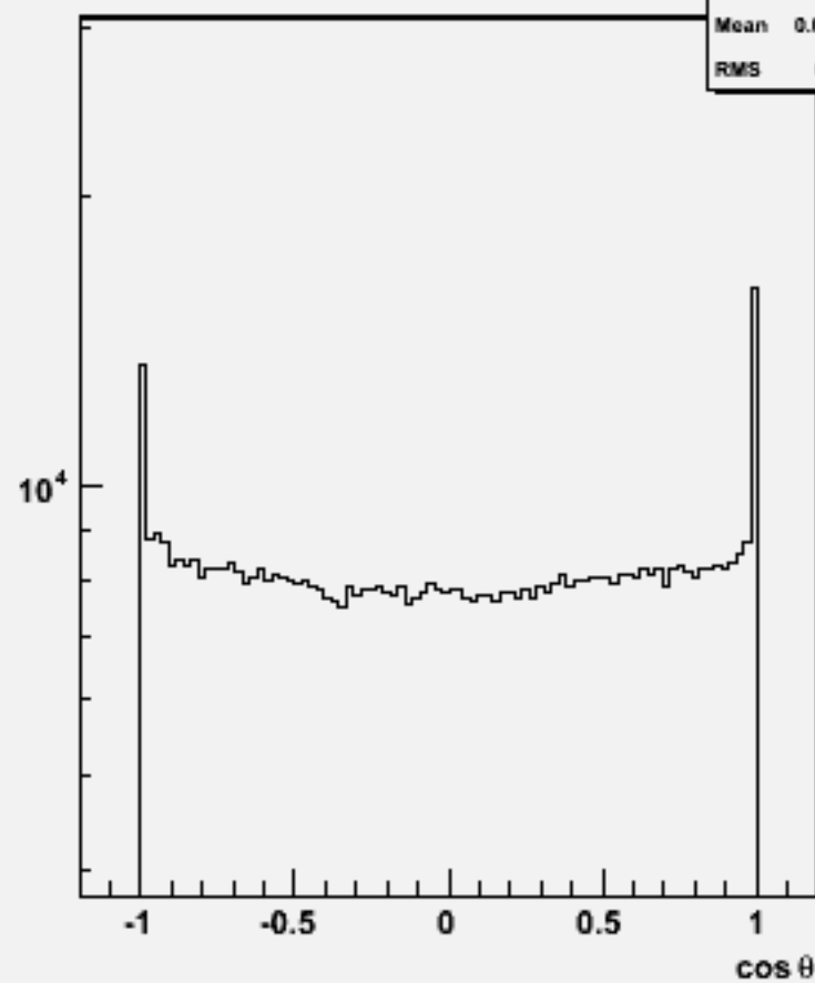
Particle cosθ : w104529 e3e3h_o
