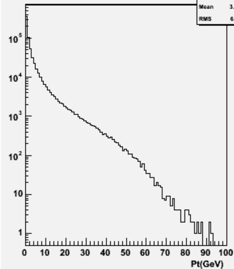
Particle Pt : w104529 e3e3h_o
