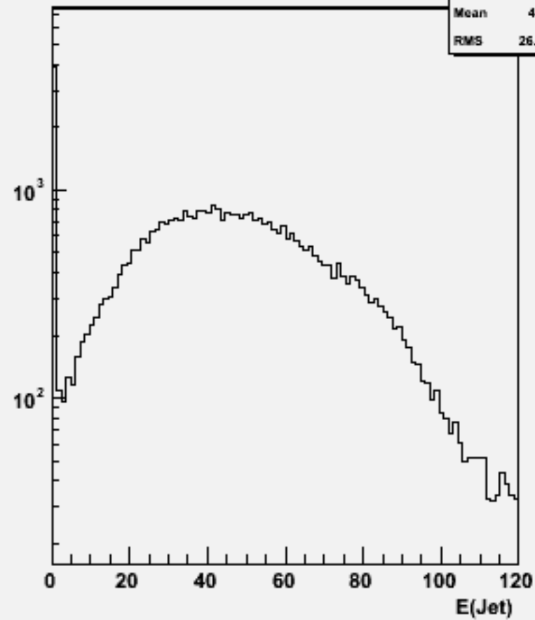
Jet energies(All jets)w104529 e3e3h_o
