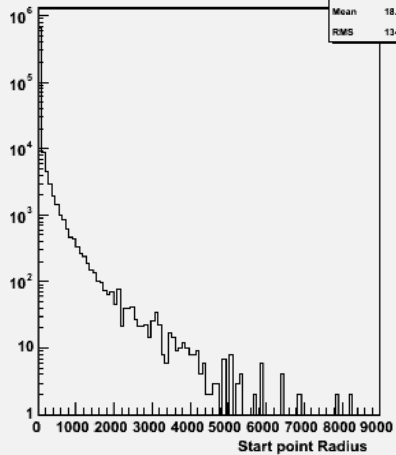
Start point R : w104529 e3e3h_o
