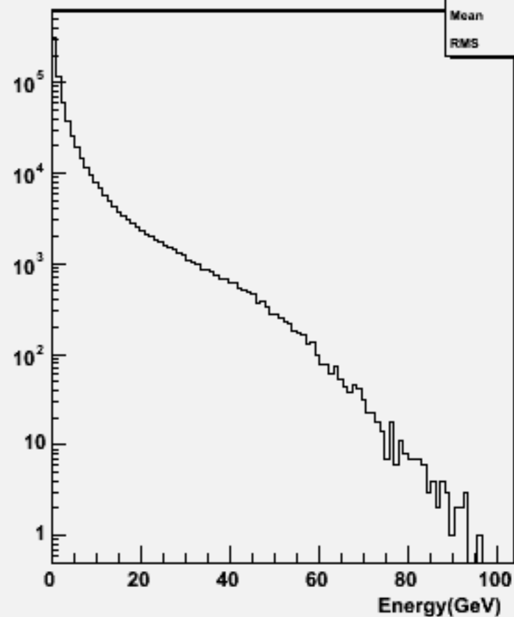
Particle Energy : w104529 e3e3h_o
