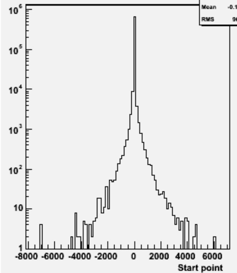
Start point Z : w104529 e3e3h_o
