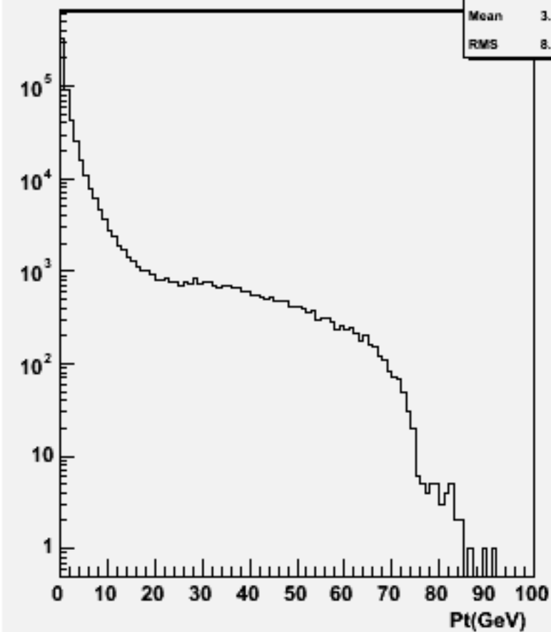
Particle Pt : w104526 e2e2h_o
