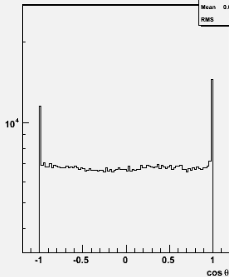
Particle cosθ : w104526 e2e2h_o
