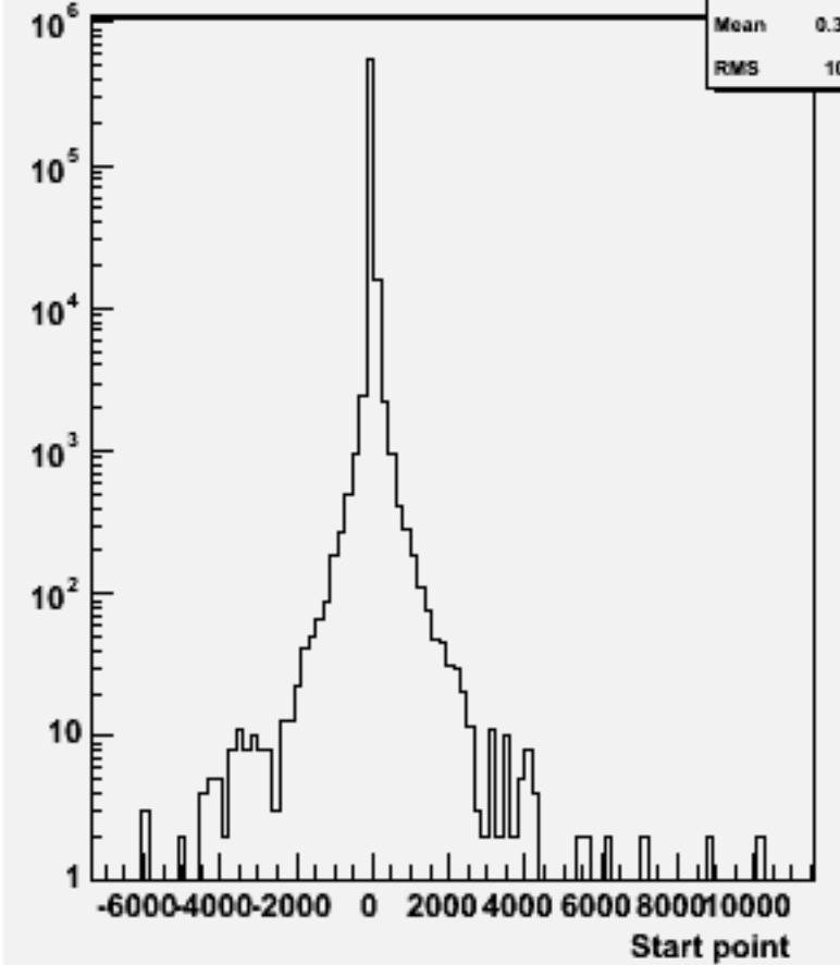
Start point Z : w104526 e2e2h_o
