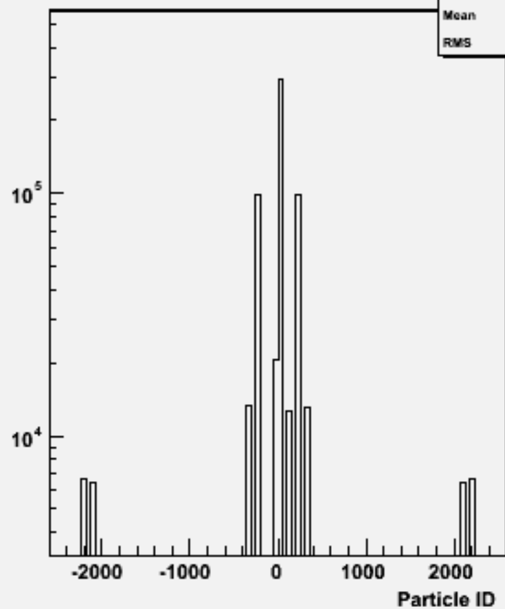
Particle ID : w104526 e2e2h_o
