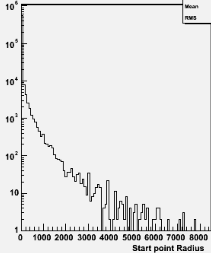
Start point R : w104526 e2e2h_o
