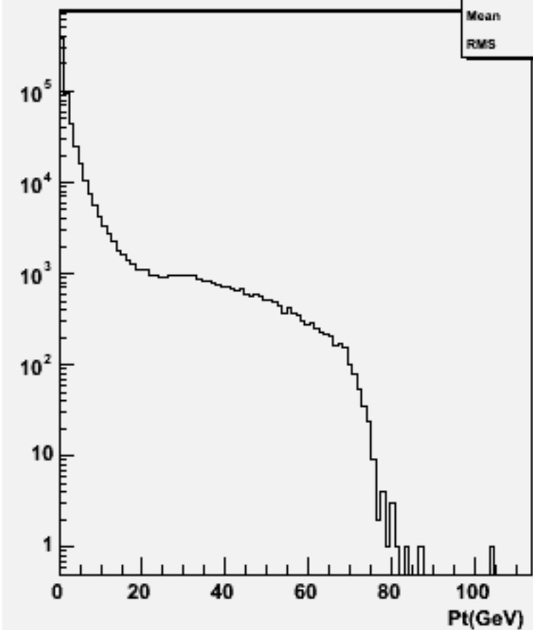
Particle Pt : w104525 e2e2h_o
