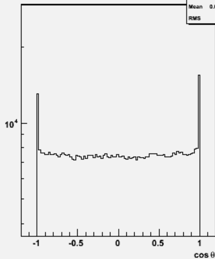
Particle cosθ : w104525 e2e2h_o
