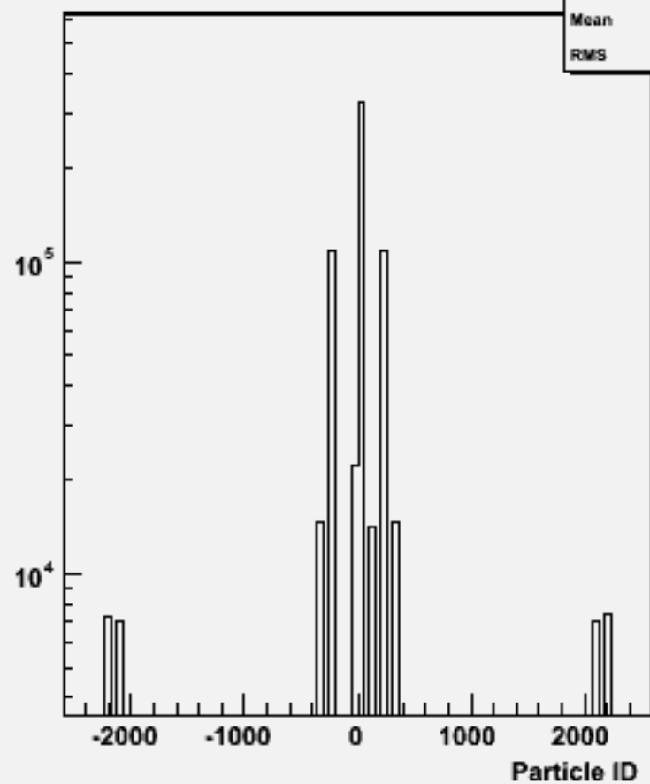
Particle ID : w104525 e2e2h_o
