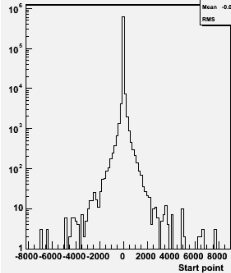
Start point Z : w104525 e2e2h_o
