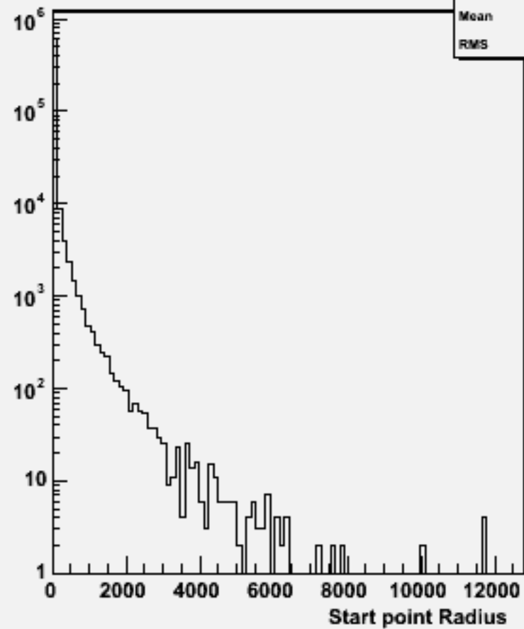
Start point R : w104525 e2e2h_o
