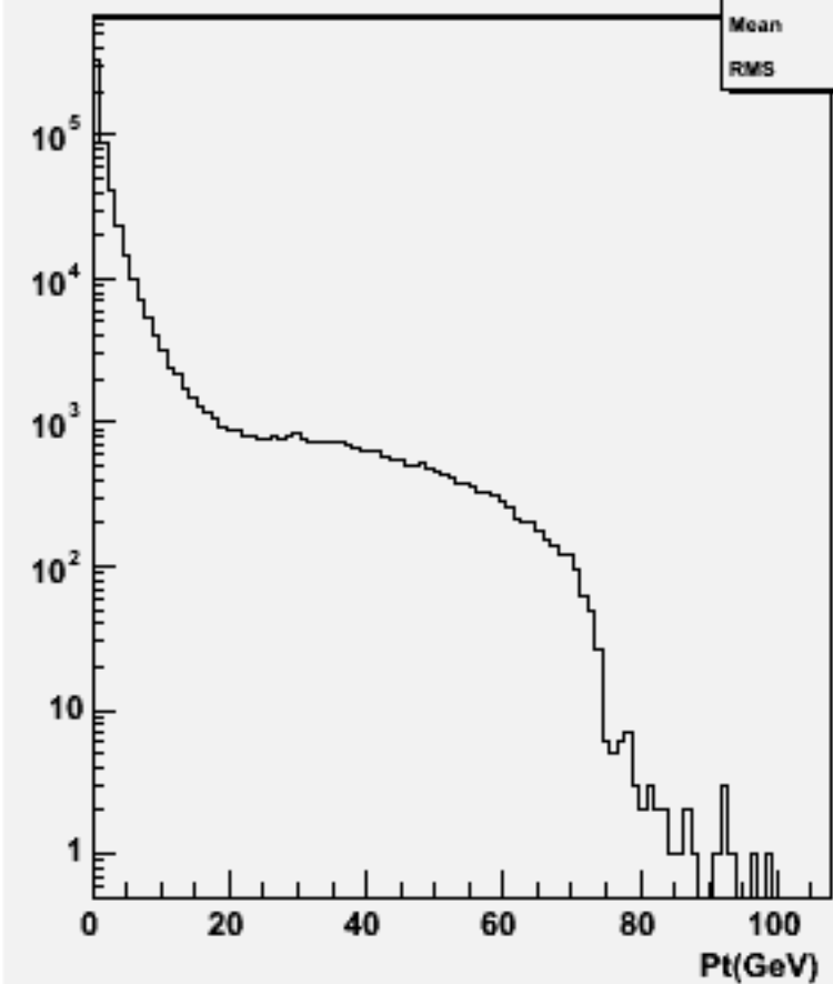
Particle Pt : w104522 e1e1h_o
