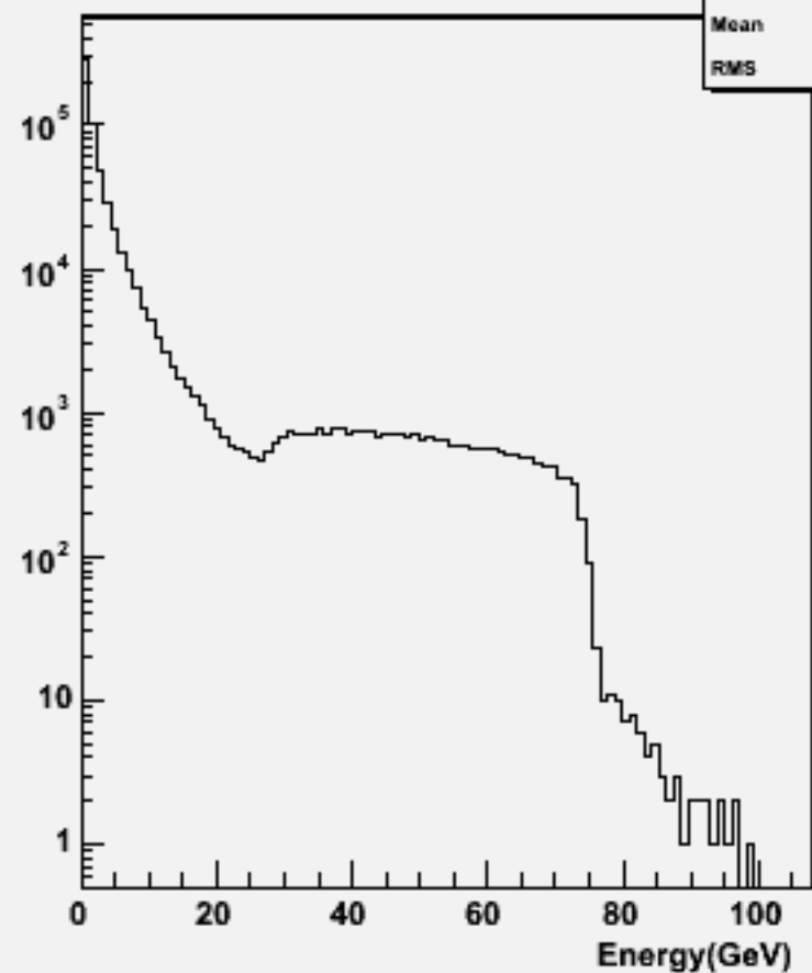
Particle Energy : w104522 e1e1h_o
