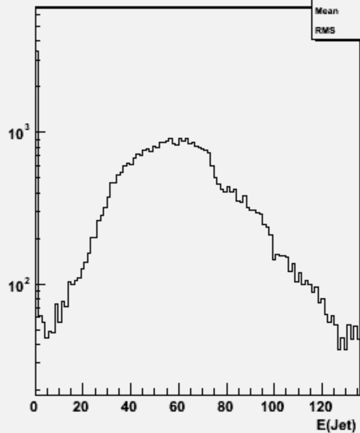
Jet energies(All jets)w104522 e1e1h_o
