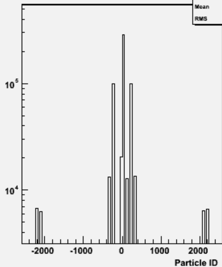
Particle ID : w104522 e1e1h_o
