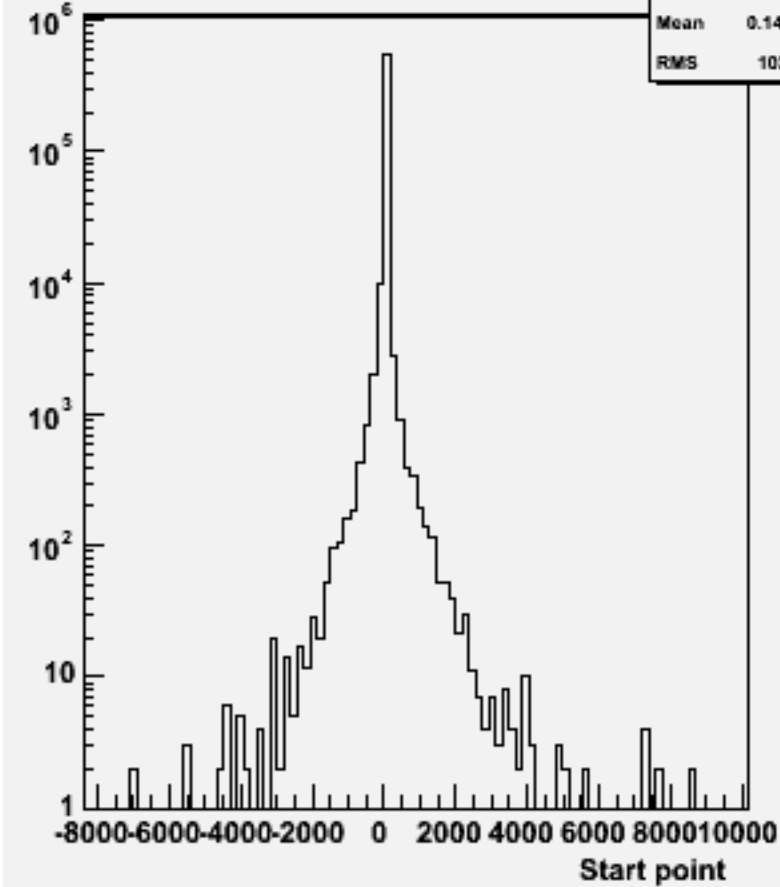
Start point Z : w104522 e1e1h_o
