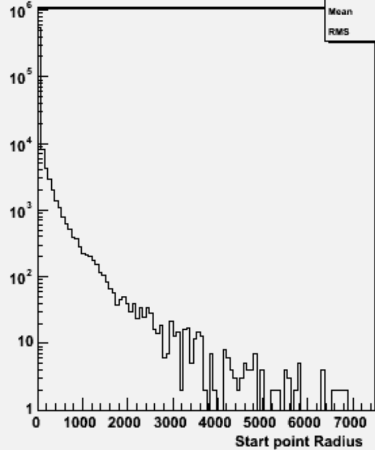
Start point R : w104522 e1e1h_o
