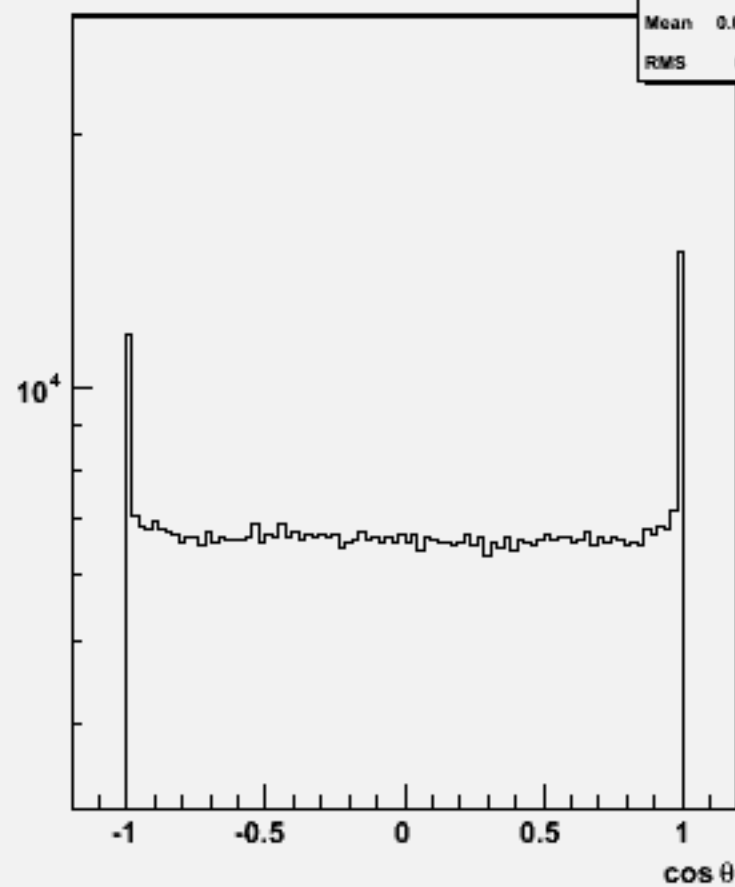
Particle cosθ : w104522 e1e1h_o
