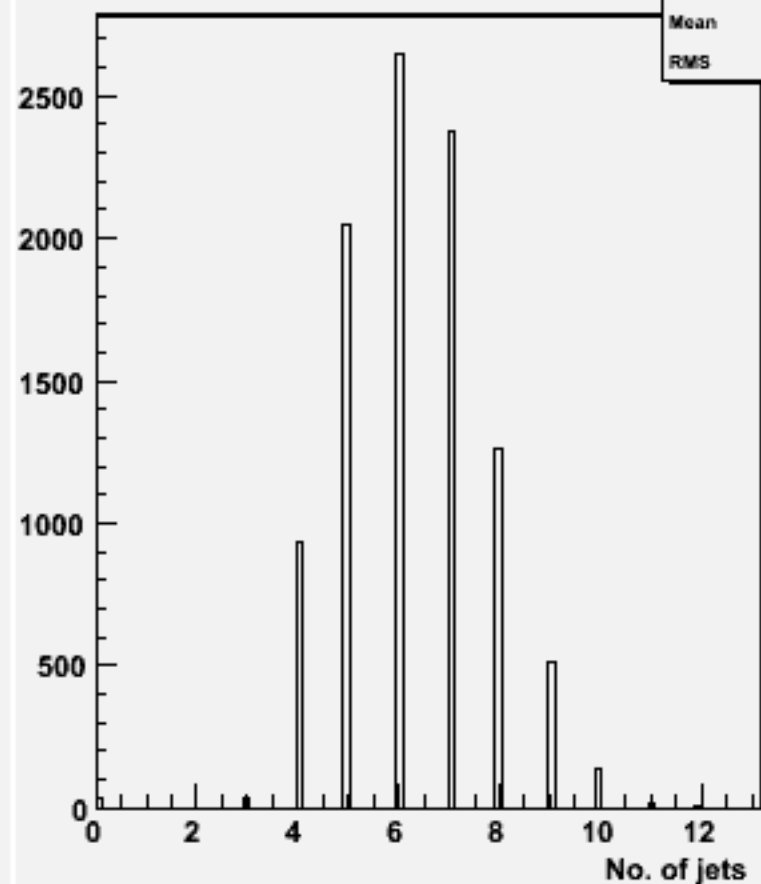
No. jets (ycut=0.001) : w104522 e1e1h_o
