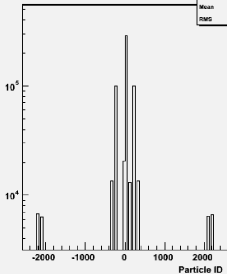
Particle ID : w104520 e1e1h_o
