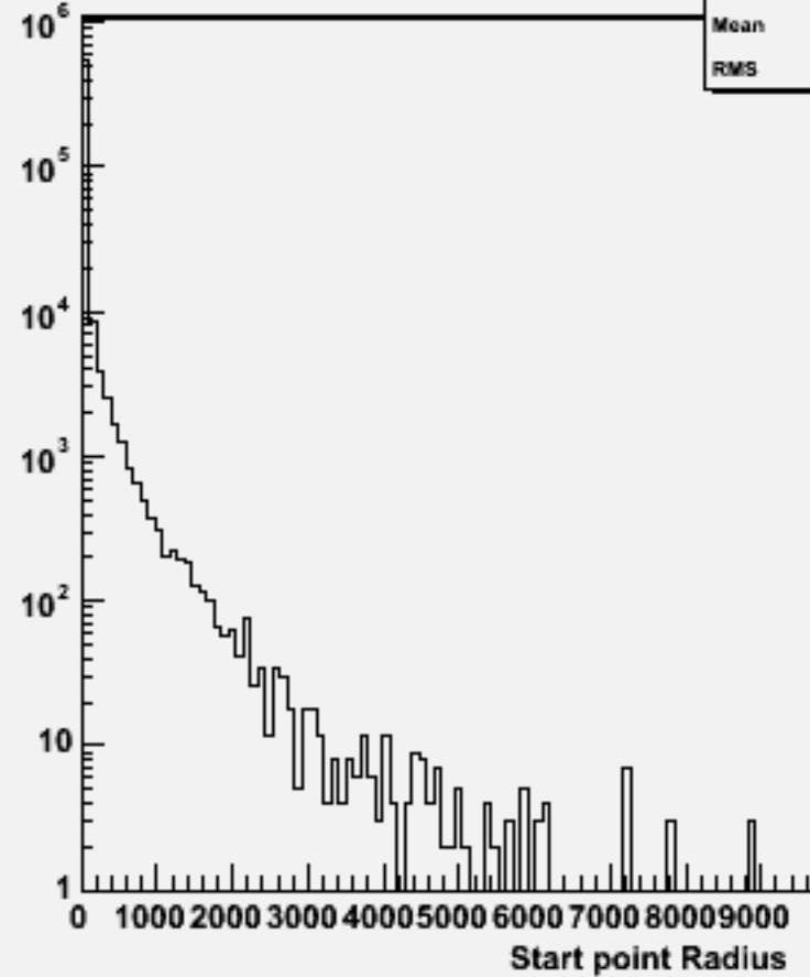
Start point R : w104520 e1e1h_o
