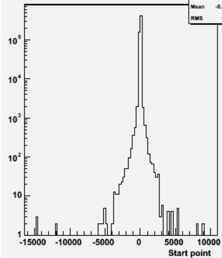
Start point Z : w104520 e1e1h_o
