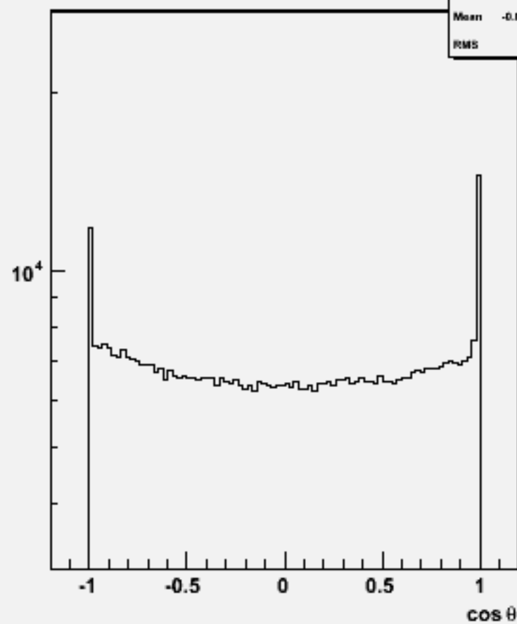
Particle cosθ : w104520 e1e1h_o
