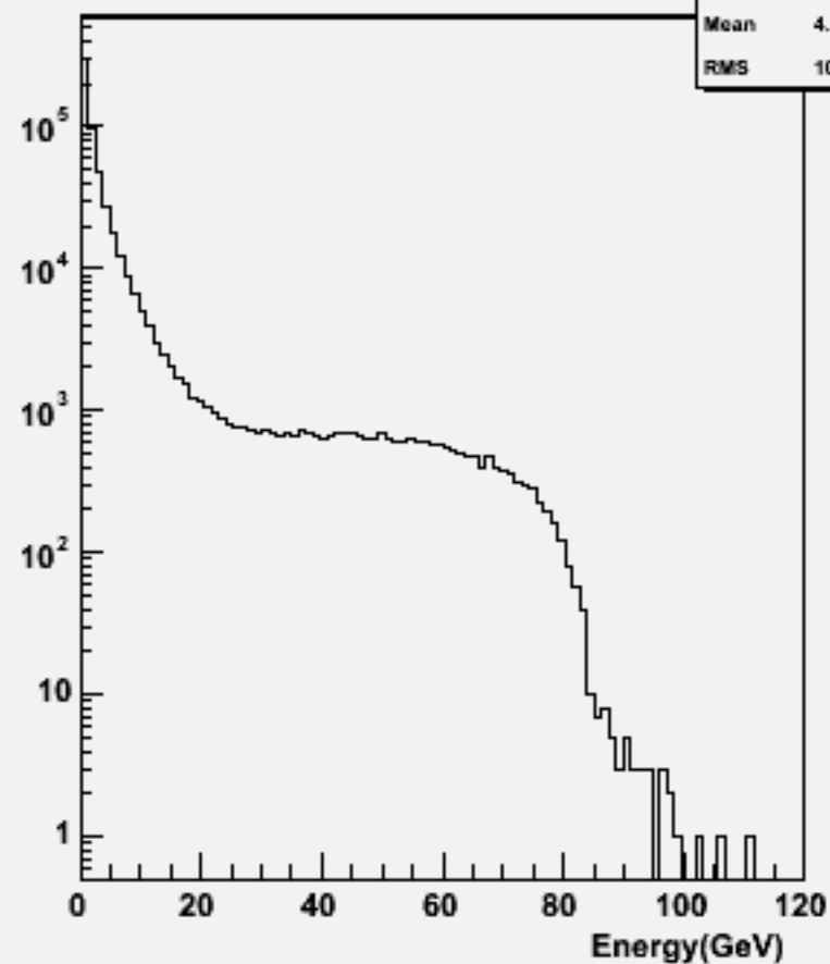
Particle Energy : w104520 e1e1h_o
