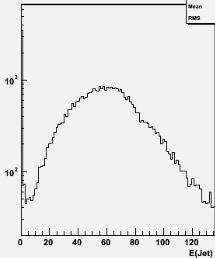
Jet energies(All jets)w104520 e1e1h_o
