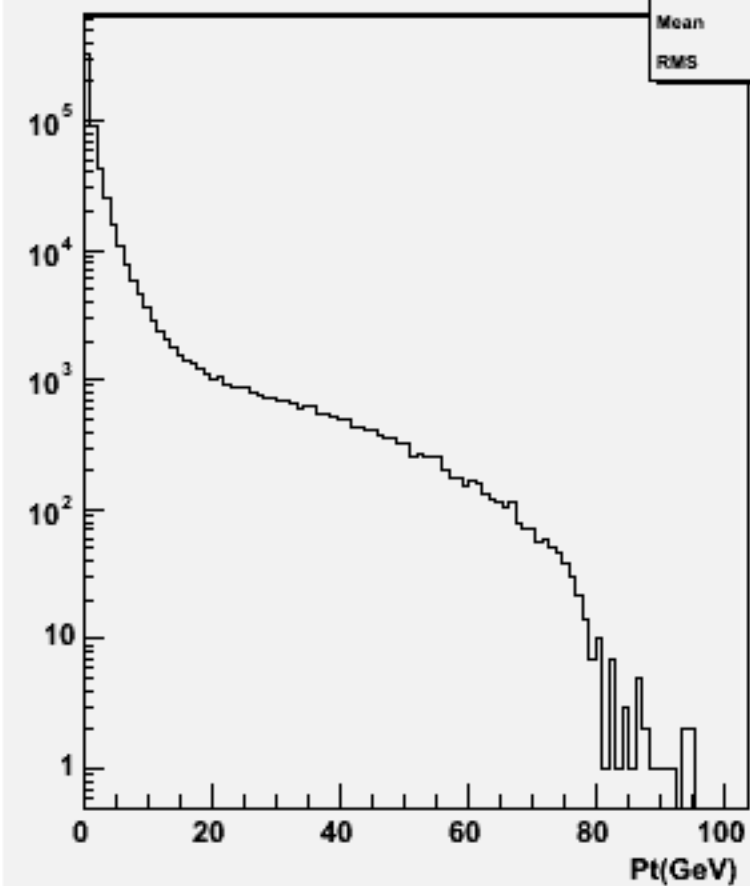
Particle Pt : w104520 e1e1h_o
