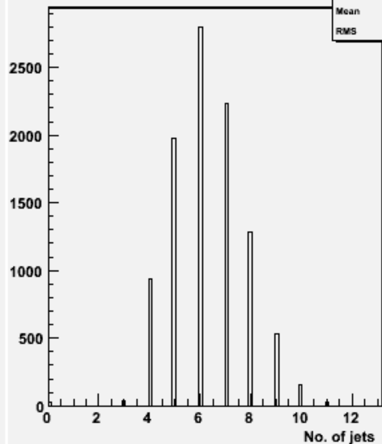
No. jets (ycut=0.001) : w104520 e1e1h_o
