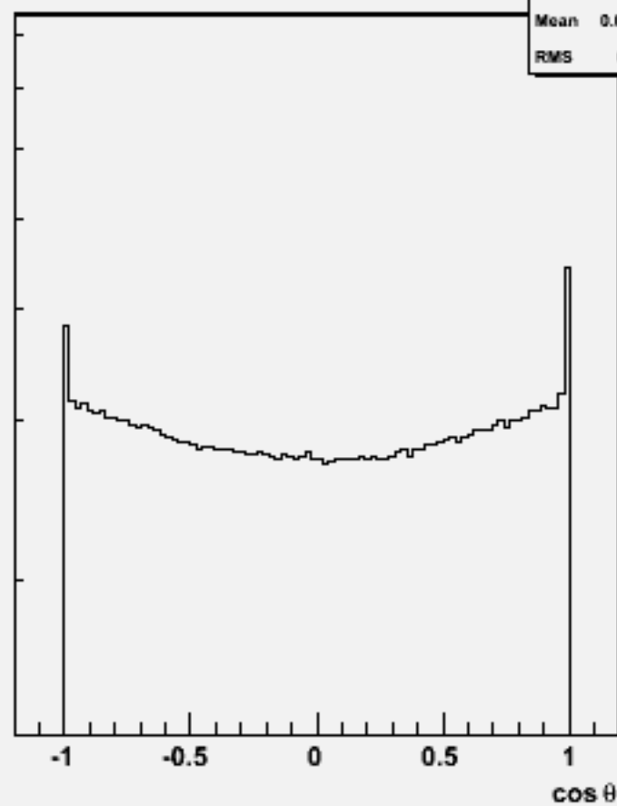
Particle cosθ : w104518 cch_o
