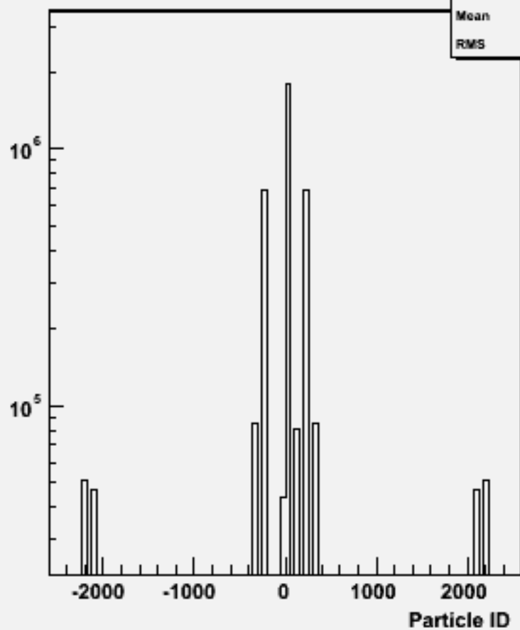
Particle ID : w104513 uuh_o
