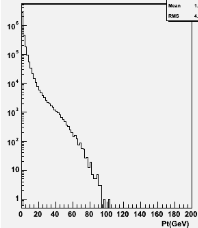
Particle Pt : w104513 uuh_o
