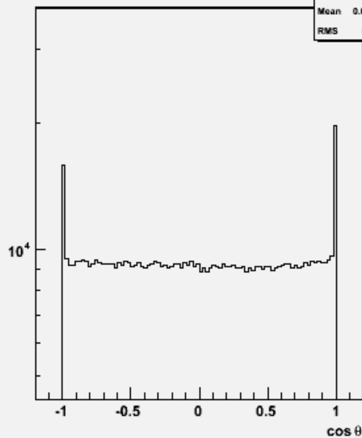
Particle \cos\theta : w104510 n3n3h_o
