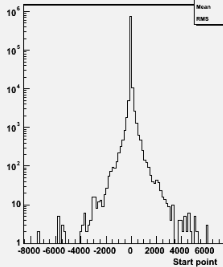
Start point Z : w104510 n3n3h_o
