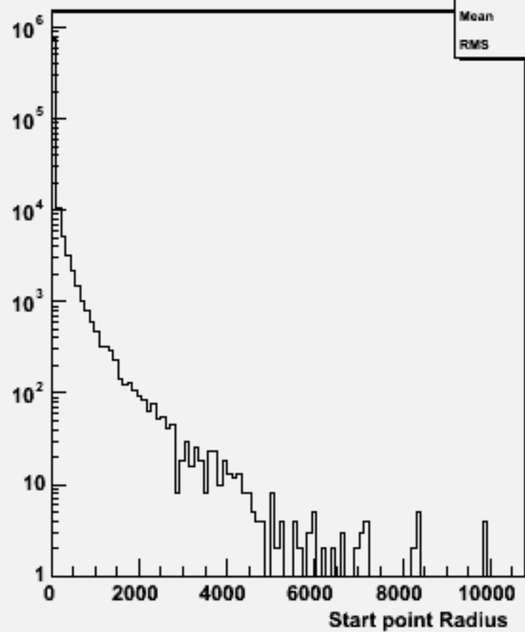
Start point R : w104510 n3n3h_o
