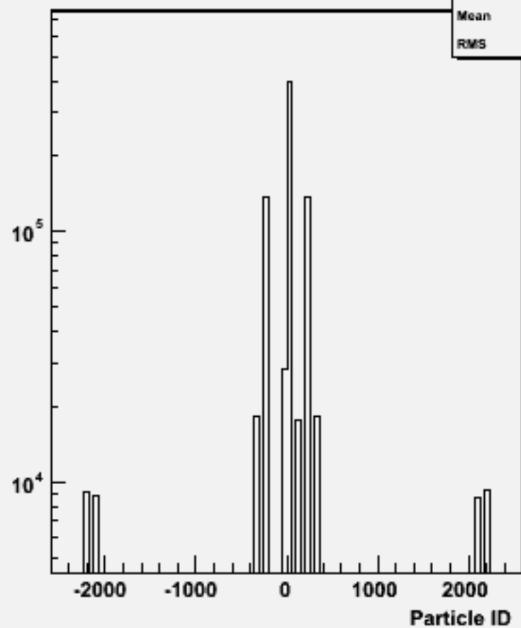
Particle ID : w104510 n3n3h_o
