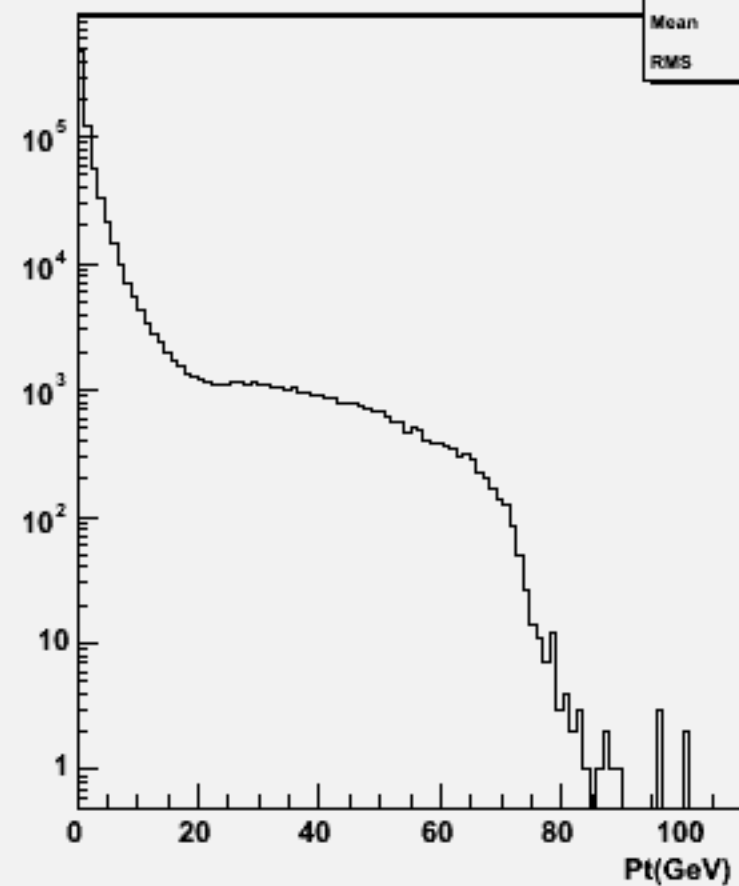
Particle Pt : w104510 n3n3h_o
