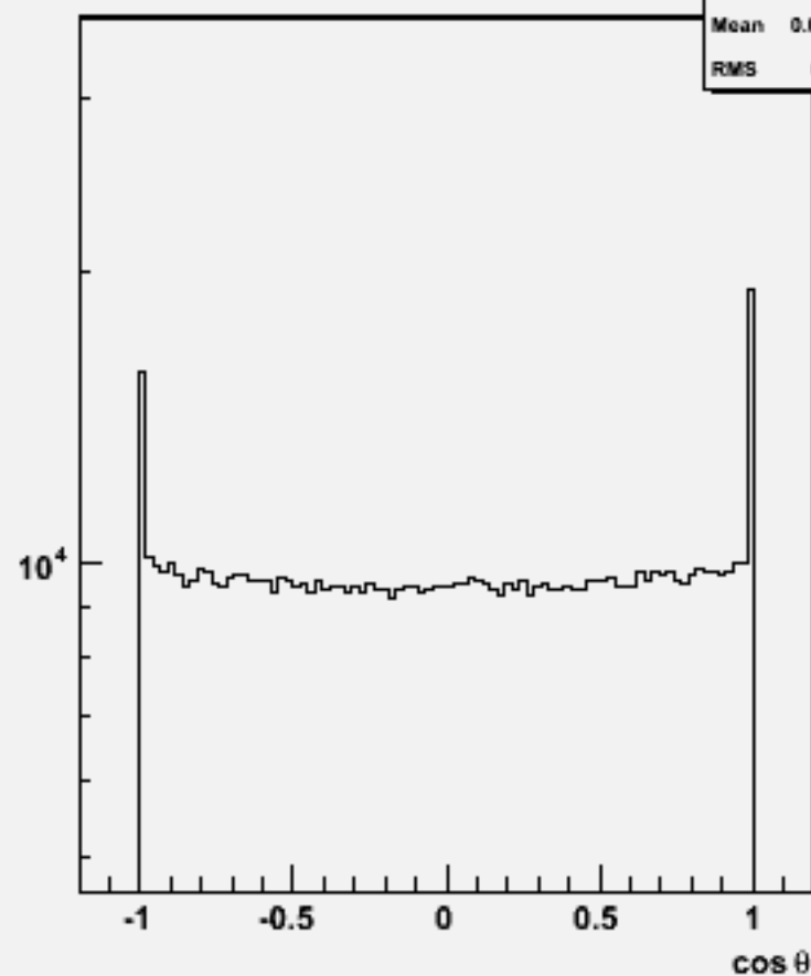
Particle cosθ : w104479 e3e3h_o
