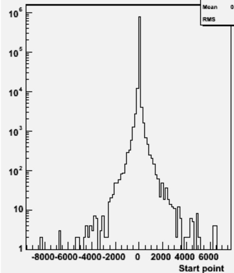
Start point Z : w104479 e3e3h_o
