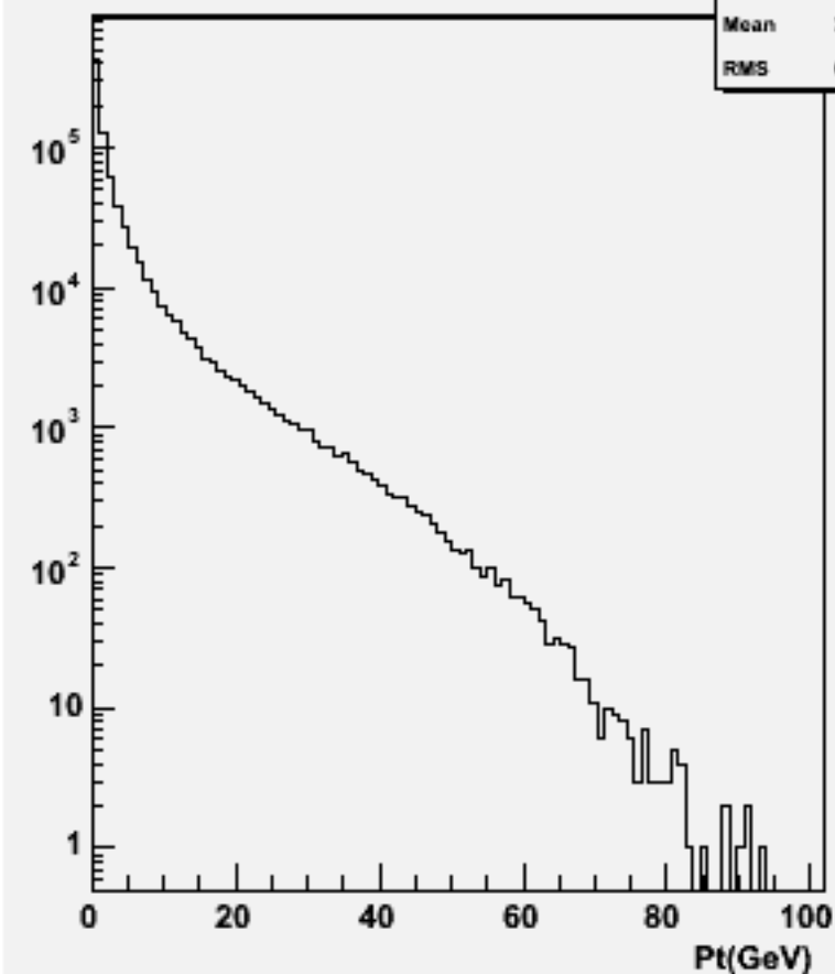
Particle Pt : w104479 e3e3h_o
