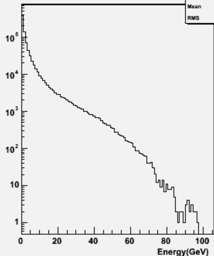
Particle Energy : w104479 e3e3h_o
