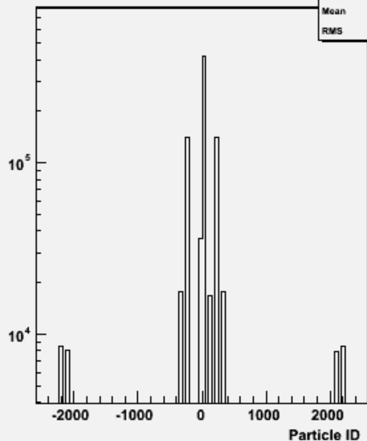
Particle ID : w104479 e3e3h_o
