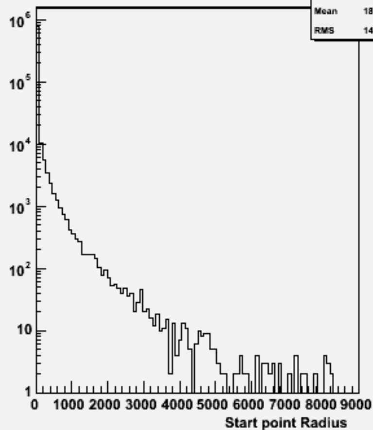
Start point R : w104479 e3e3h_o
