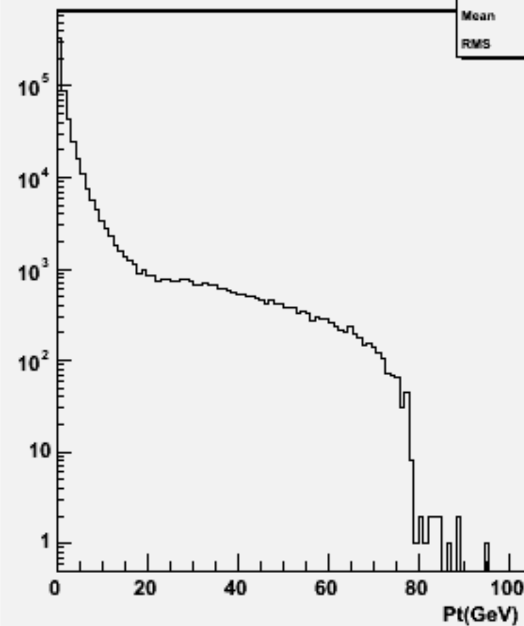
Particle Pt : w104476 e2e2h_o
