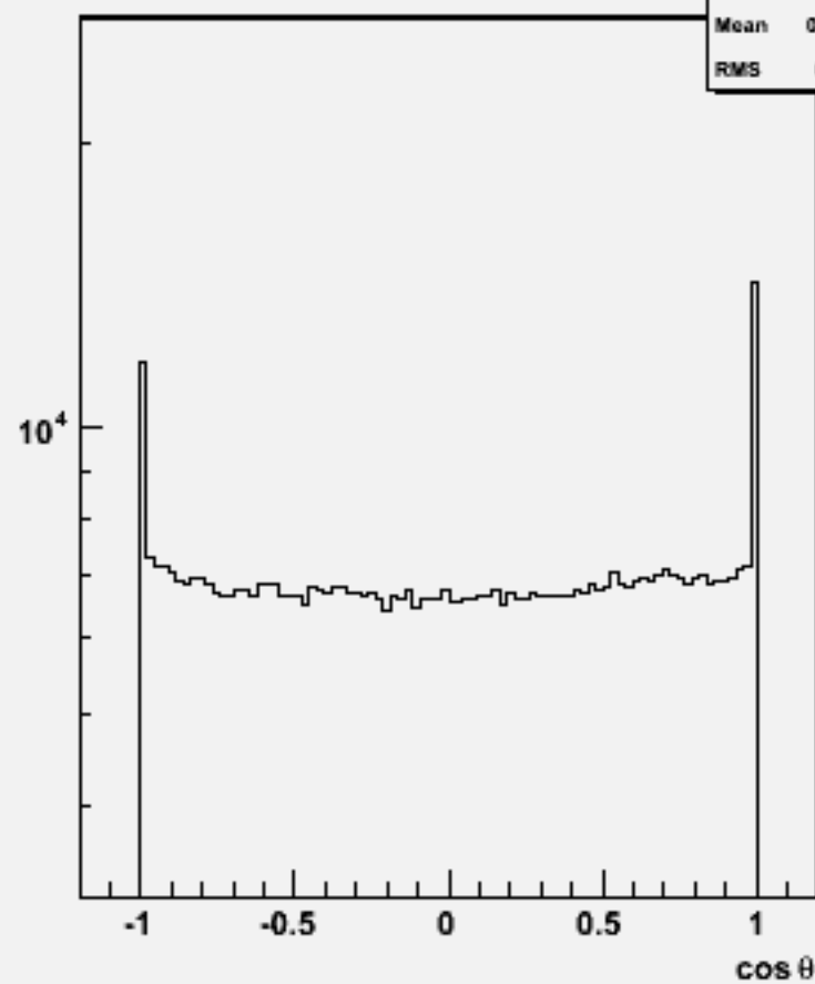
Particle cos \theta : w104476 e2e2h_o
