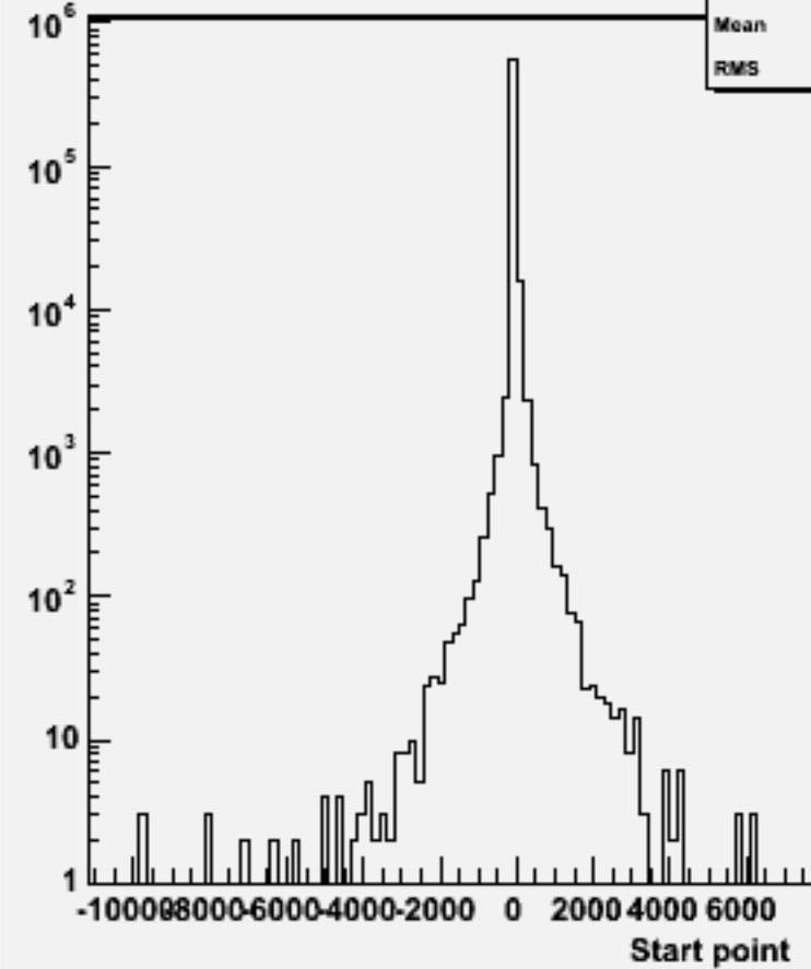
Start point Z : w104476 e2e2h_o
