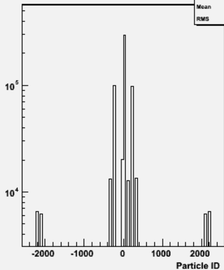
Particle ID : w104476 e2e2h_o
