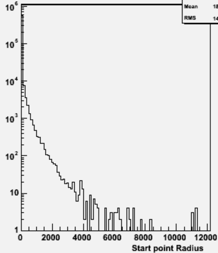
Start point R : w104476 e2e2h_o
