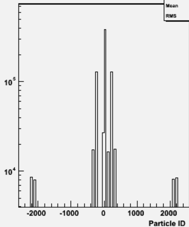
Particle ID : w104475 e2e2h_o
