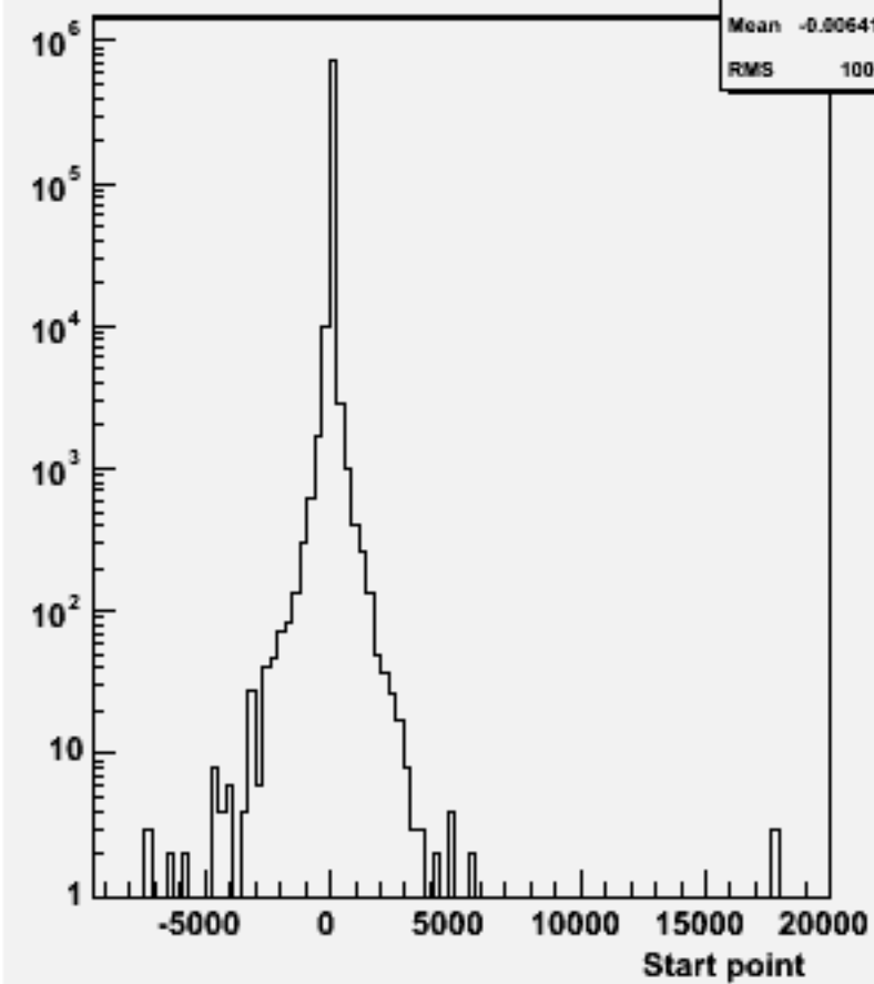
Start point Z : w104475 e2e2h_o
