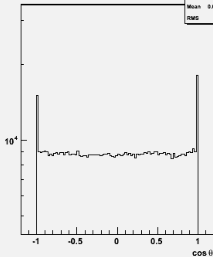
Particle cosθ : w104475 e2e2h_o
