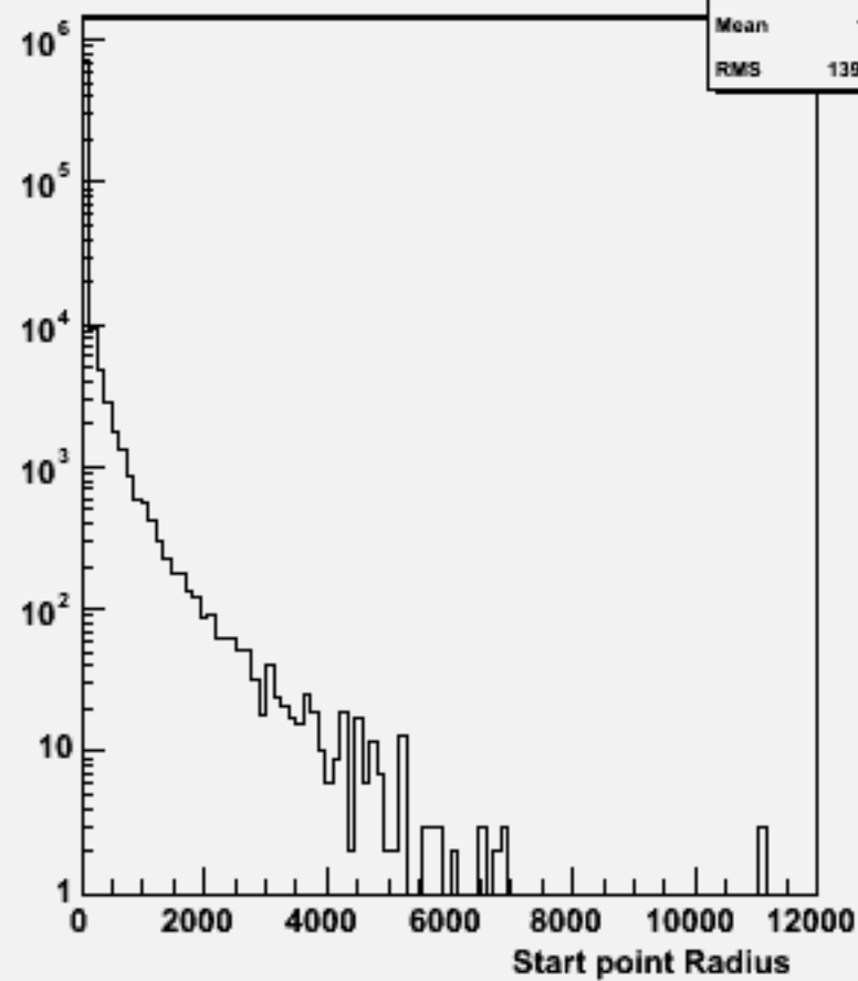
Start point R : w104475 e2e2h_o
