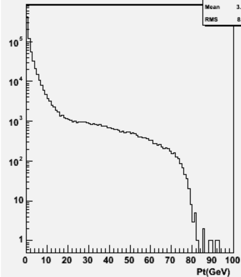
Particle Pt : w104475 e2e2h_o
