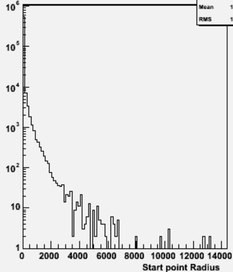
Start point R : w104473 e1e1h_o
