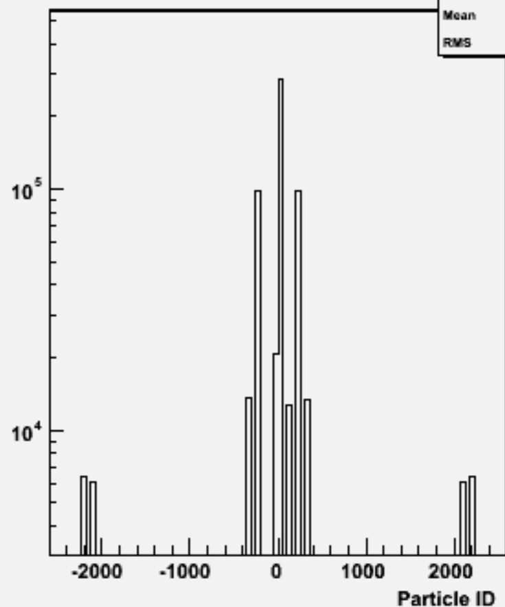
Particle ID : w104473 e1e1h_o
