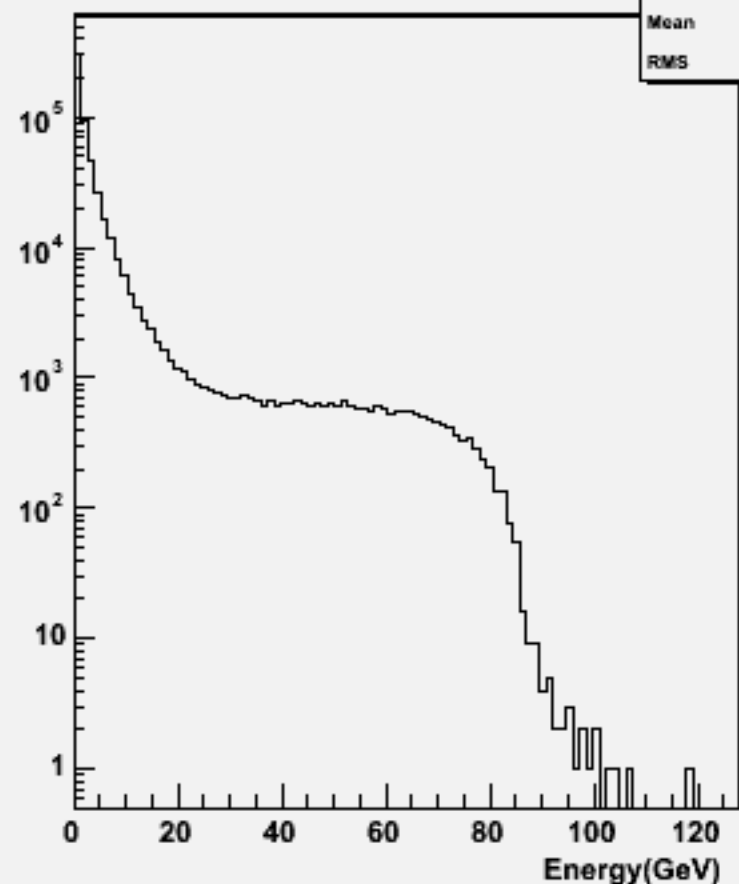
Particle Energy : w104473 e1e1h_o
