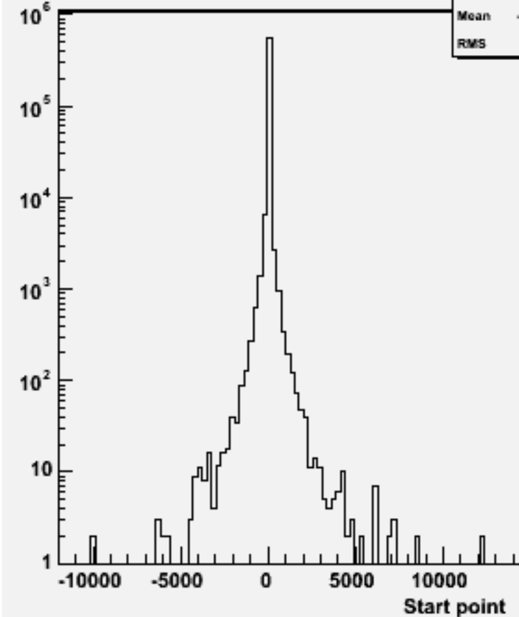
Start point Z : w104473 e1e1h_o
