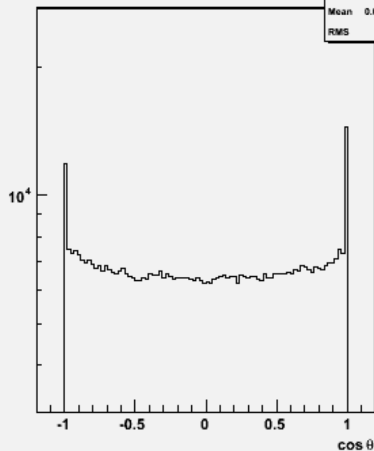
Particle cosθ : w104473 e1e1h_o
