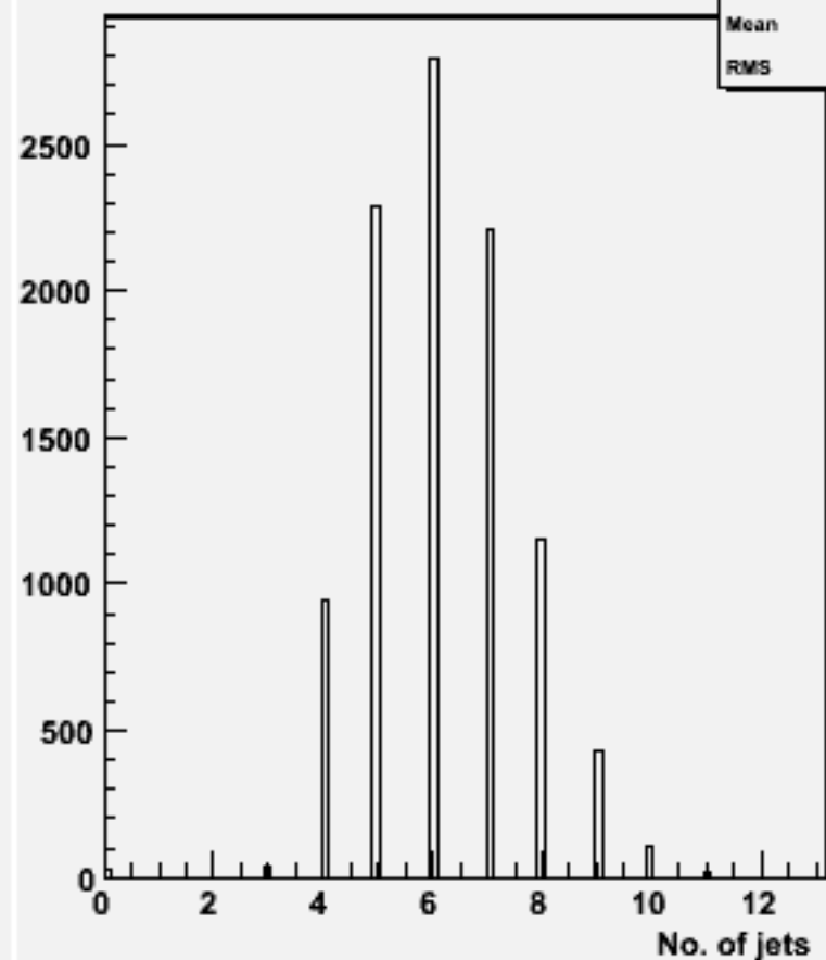
No. jets (ycut=0.001) : w104473 e1e1h_o
