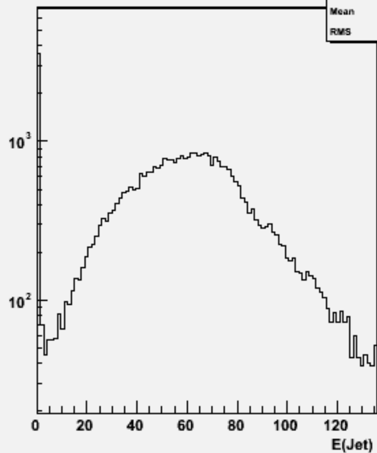
Jet energies(All jets)w104473 e1e1h_o
