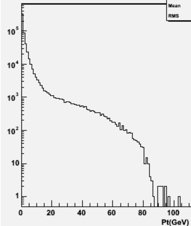
Particle Pt : w104473 e1e1h_o
